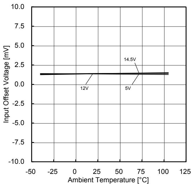
Figure 15. 入力オフセット電圧 vs 温度特性 ( V_{ICM}=V_{DD}/2 , E_K=-V_{DD}/2 )
