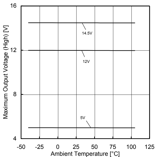
Figure 30. 最大出力電圧(High) vs 温度特性 ( R_L=10k\Omega )
