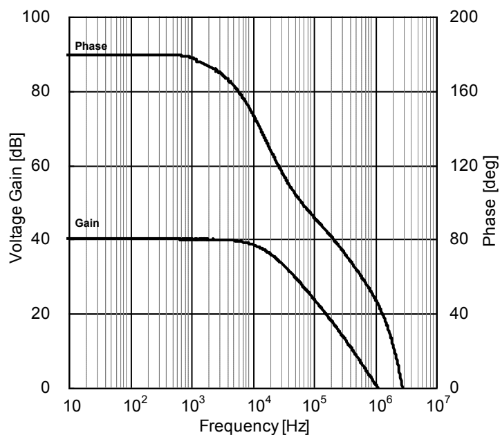
Figure 47. 電圧利得・位相 vs 周波数特性
