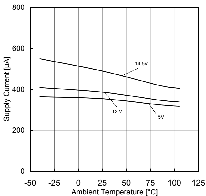
Figure 5. 回路電流 vs 温度特性
