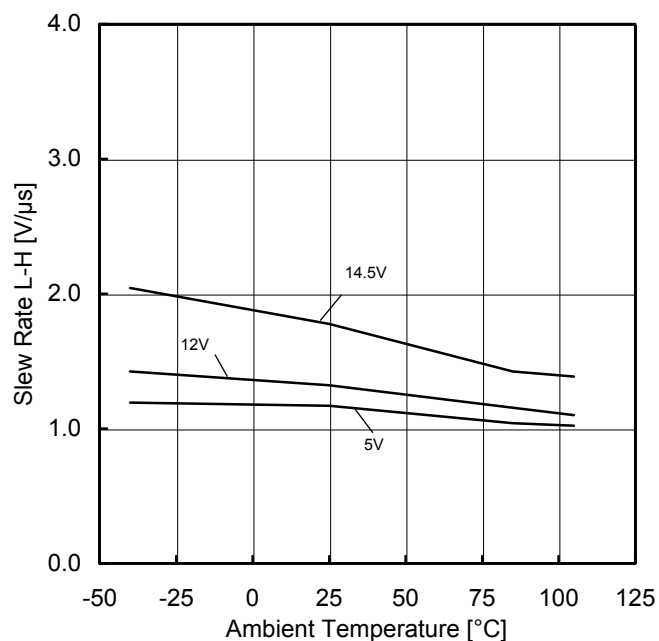
Figure 45. スルーレート(L-H) vs 温度特性
