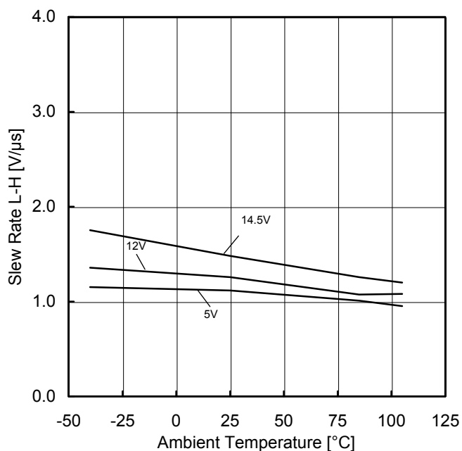
Figure 22. スルーレート(L-H) vs 温度特性
