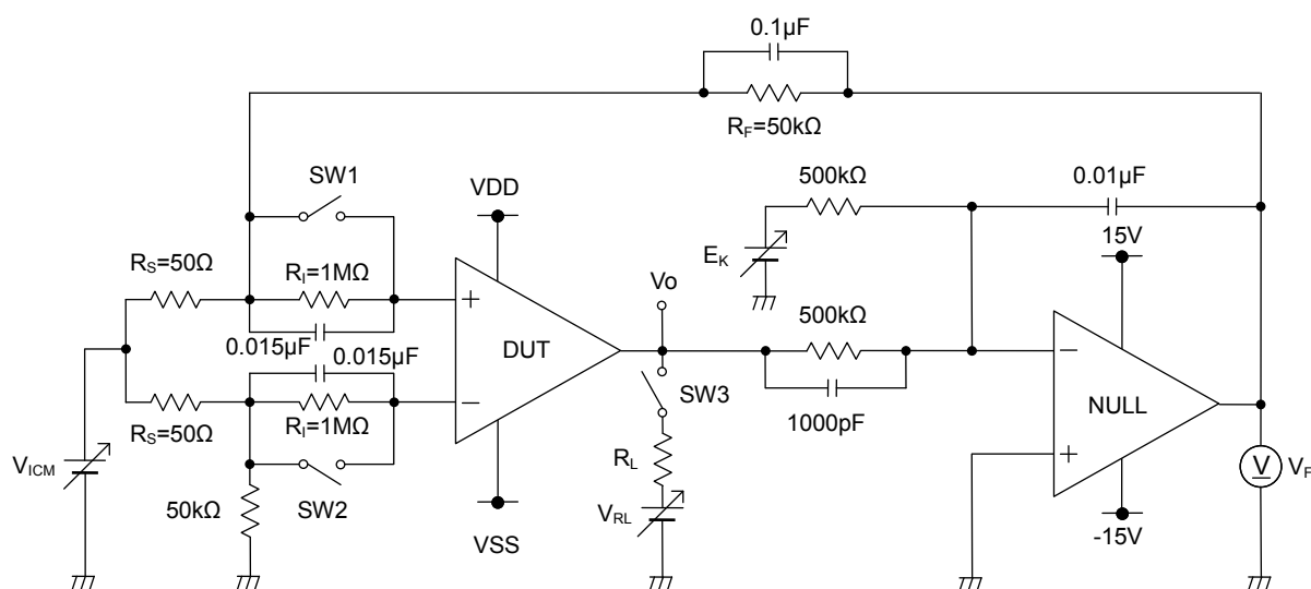
Figure 48. 測定回路 1 (1 チャンネルのみ)
