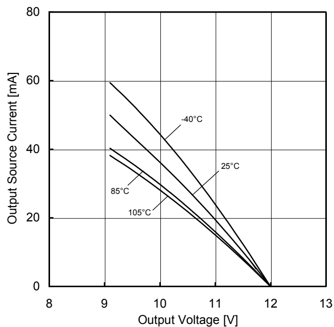
Figure 10. 出力ソース電流 vs 出力電圧特性 (VDD=12V)
