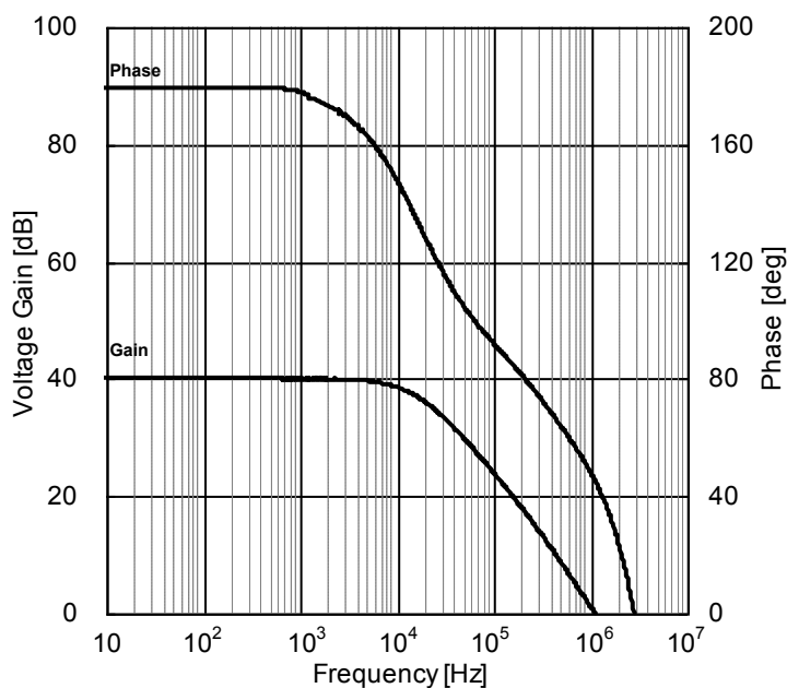
Figure 24. 電圧利得・位相 vs 周波数特性
