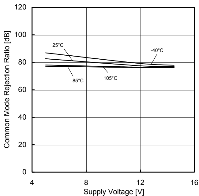
Figure 19. 同相信号除去比 vs 電源電圧特性 (VDD=12V)
