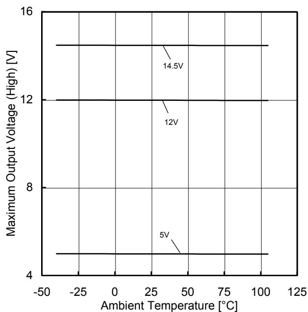
Figure 7. 最大出力電圧(High) vs 温度特性 ( R_L=10k\Omega )
