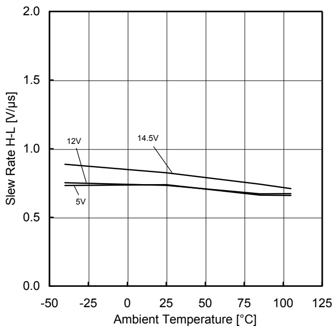
Figure 23. スルーレート(H-L) vs 温度特性
