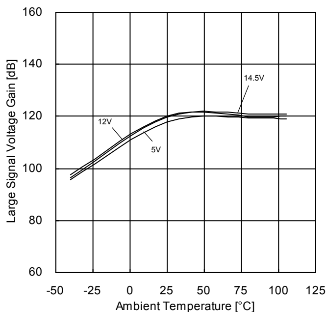
Figure 41. 大振幅電圧利得 vs 温度特性
