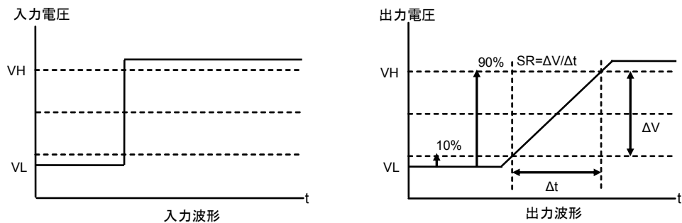
Figure 50. スルーレート測定時 入出力波形
