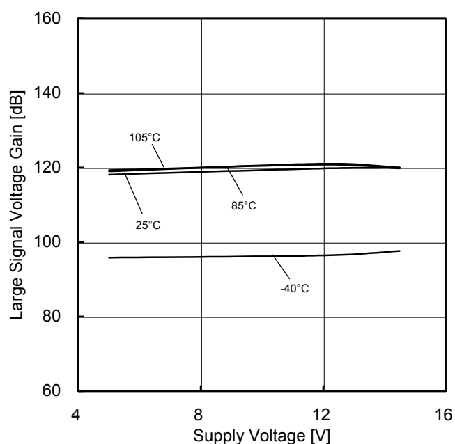
Figure 40. 大振幅電圧利得 vs 電源電圧特性
