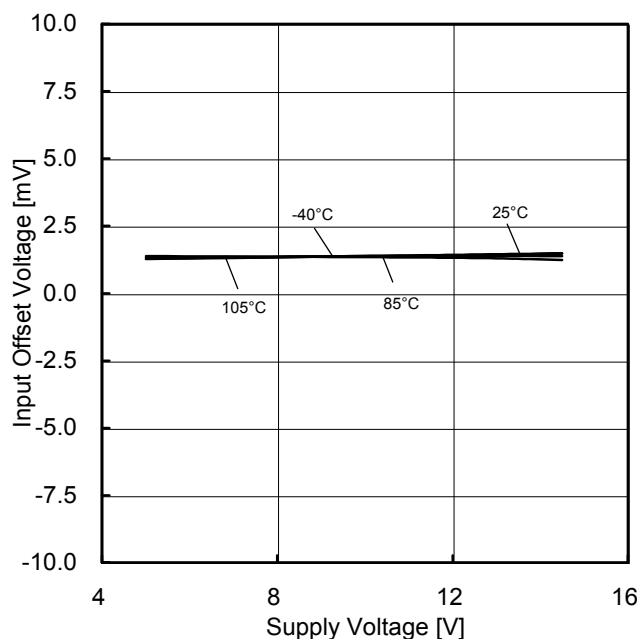
Figure 14. 入力オフセット電圧 vs 電源電圧特性 ( V_{ICM}=V_{DD}/2 , E_K=-V_{DD}/2 )
