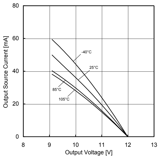
Figure 33. 出力ソース電流 vs 出力電圧特性 (VDD=12V)
