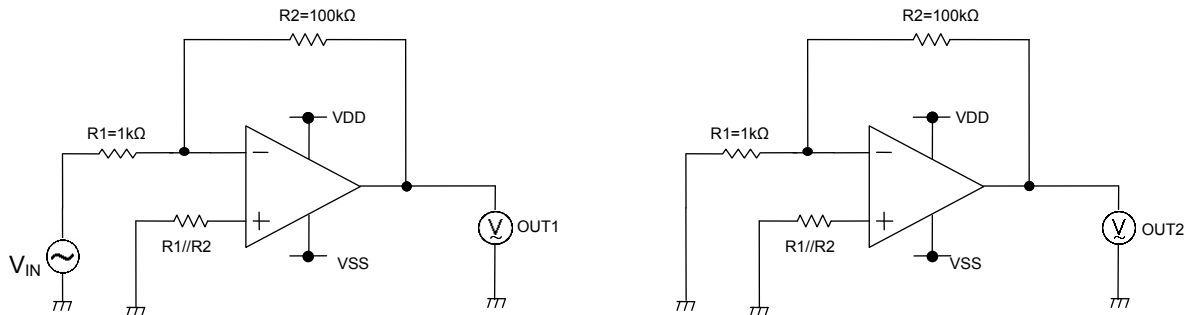
Figure 51. 測定回路 3 (チャンネルセパレーション)
