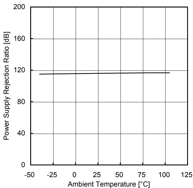
Figure 44. 電源電圧除去比 vs 温度特性
