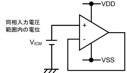
Figure 53. 未使用回路処理例
