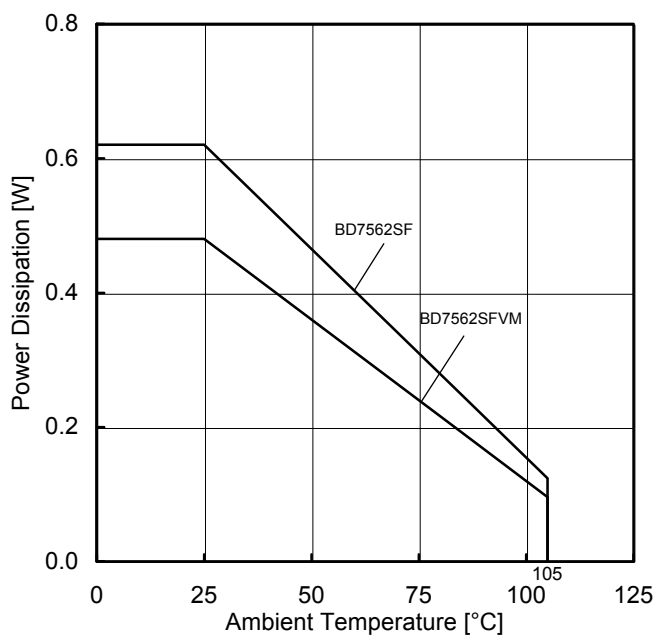
Figure 26. ディレーティングカーブ
