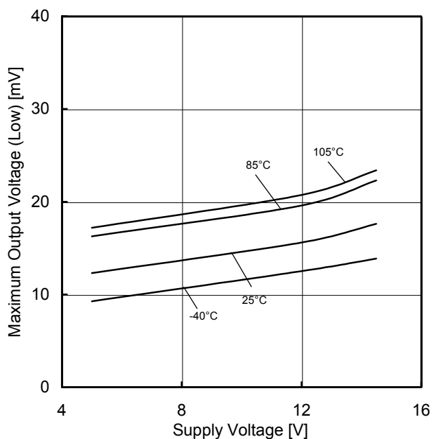
Figure 8. 最大出力電圧(Low) vs 電源電圧特性 ( R_L=10k\Omega )
