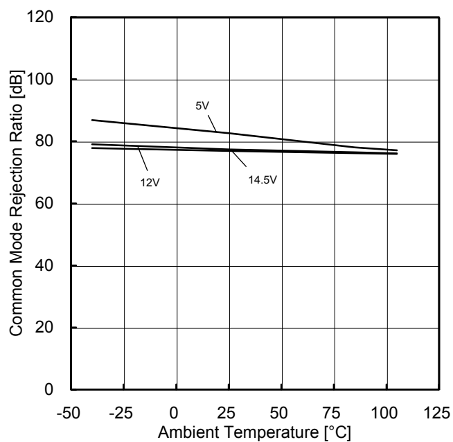
Figure 20. 同相信号除去比 vs 温度特性 (VDD=12V)
