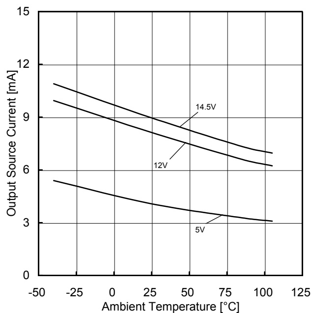
Figure 11. 出力ソース電流 vs 温度特性 (OUT=VDD-0.4V)
