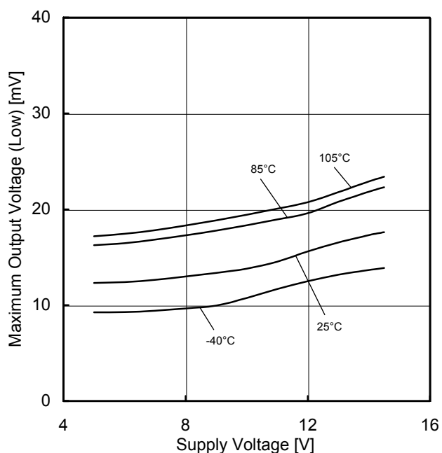
Figure 31. 最大出力電圧(Low) vs 電源電圧特性 ( R_L=10k\Omega )
