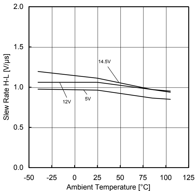
Figure 46. スルーレート(H-L) vs 温度特性
