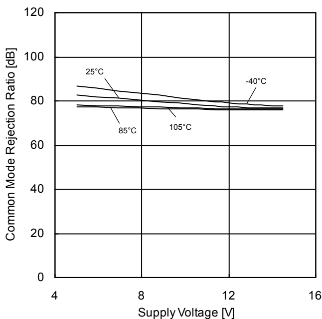
Figure 42. 同相信号除去比 vs 電源電圧特性 (VDD=12V)
