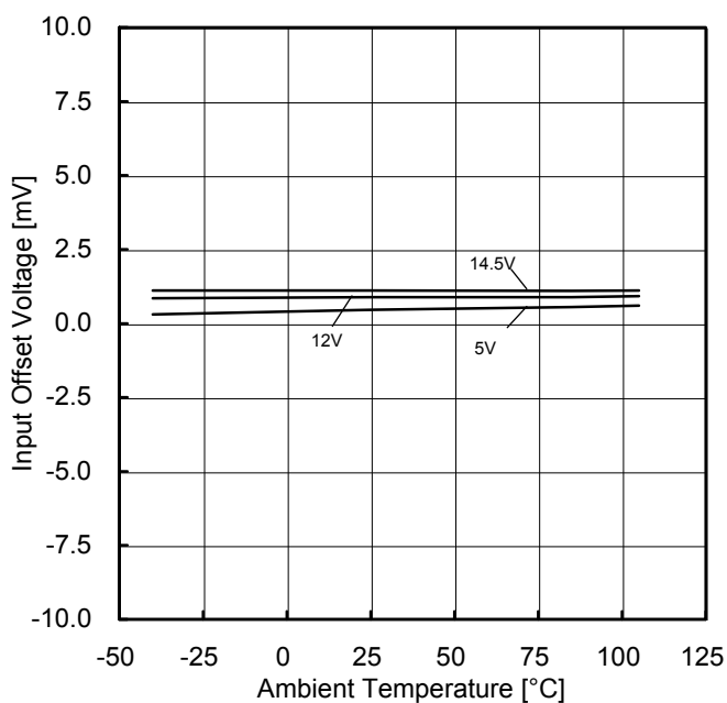
Figure 38. 入力オフセット電圧 vs 温度特性 ( V_{ICM}=V_{DD}/2 , E_K=-V_{DD}/2 )
