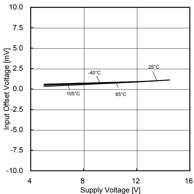
Figure 37. 入力オフセット電圧 vs 電源電圧特性 ( V_{ICM}=V_{DD}/2 , E_K=-V_{DD}/2 )
