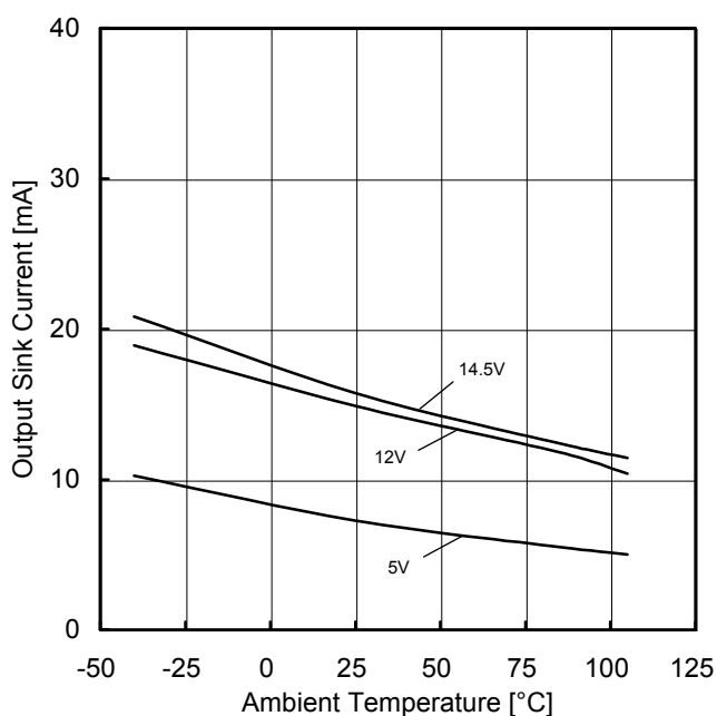
Figure 13. 出力シンク電流 vs 温度特性 (OUT=VSS+0.4V)
