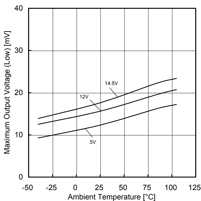
Figure 32. 最大出力電圧(Low) vs 温度特性 ( R_L=10k\Omega )
