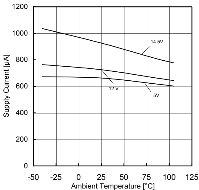
Figure 28. 回路電流 vs 温度特性
