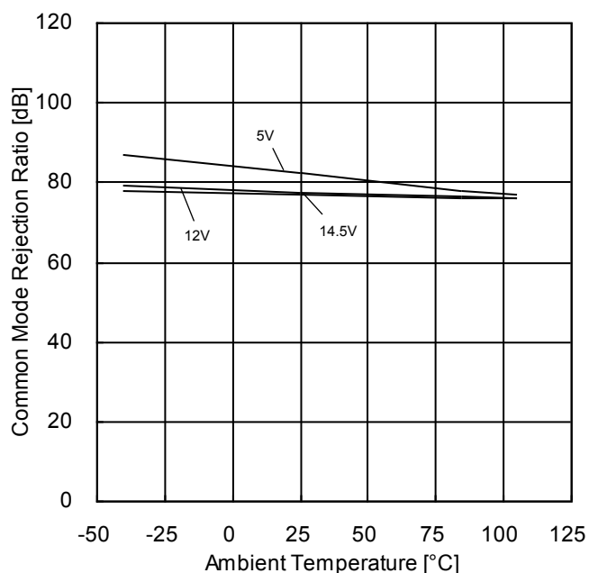
Figure 43. 同相信号除去比 vs 温度特性 (VDD=12V)
