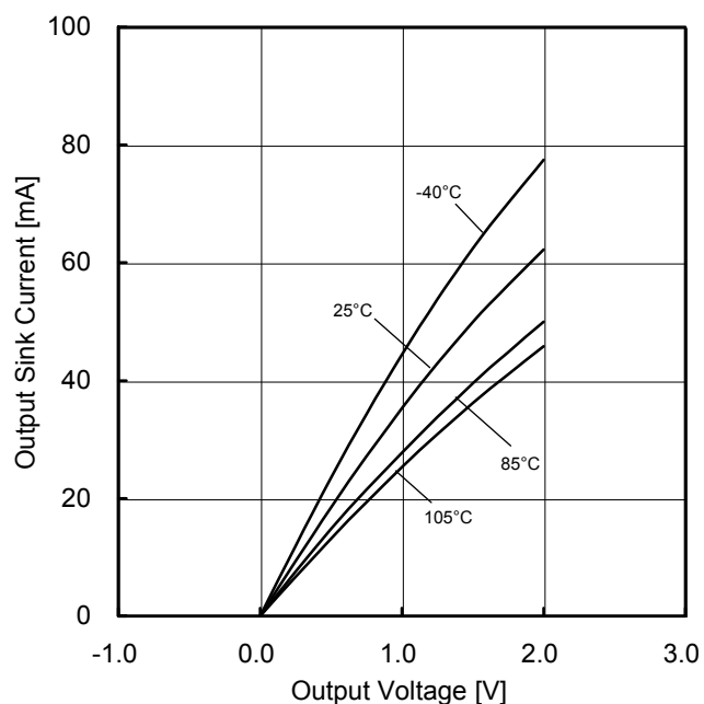
Figure 12. 出力シンク電流 vs 出力電圧特性 (VDD=3V)
