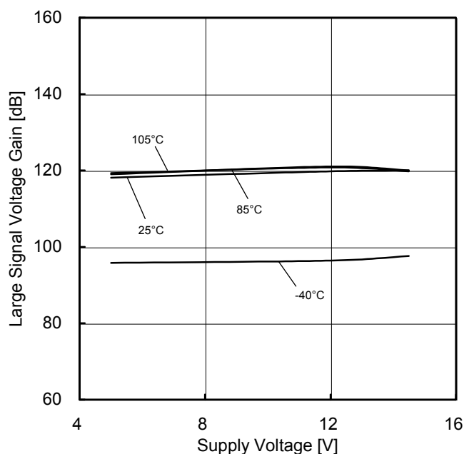
Figure 17. 大振幅電圧利得 vs 電源電圧特性
