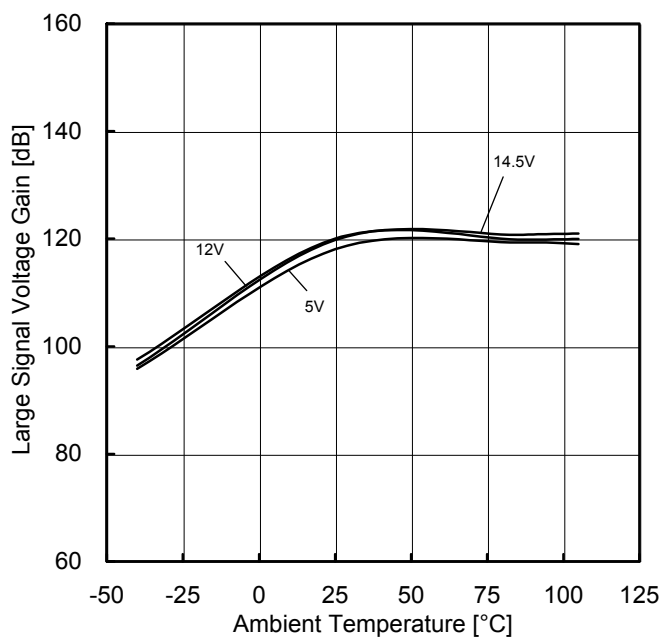
Figure 18. 大振幅電圧利得 vs 温度特性
