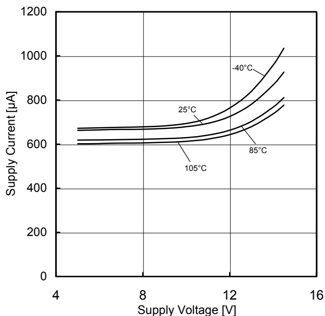
Figure 27. 回路電流 vs 電源電圧特性
