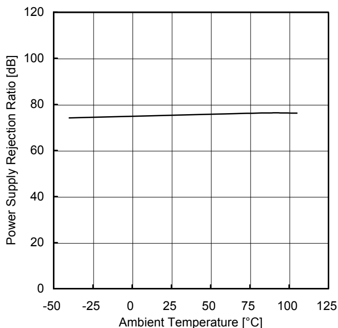
Figure 21. 電源電圧除去比 vs 温度特性
