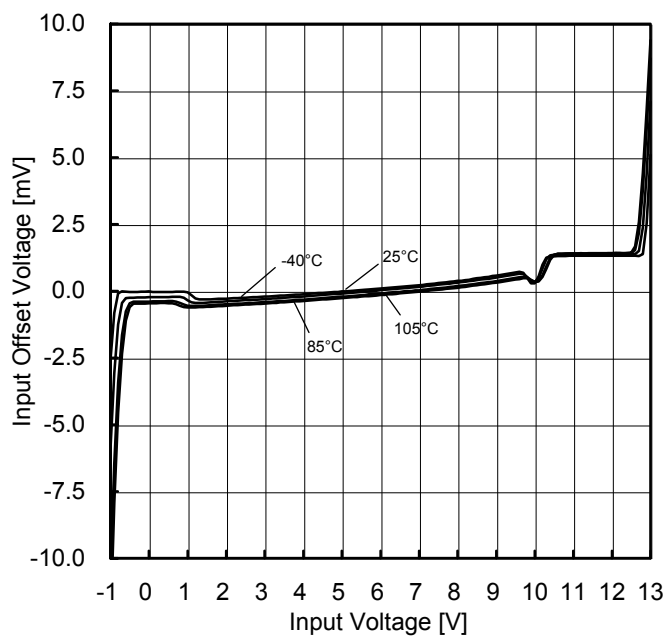
Figure 16. 同相入力電圧範囲 ( V_{DD}=12V )
