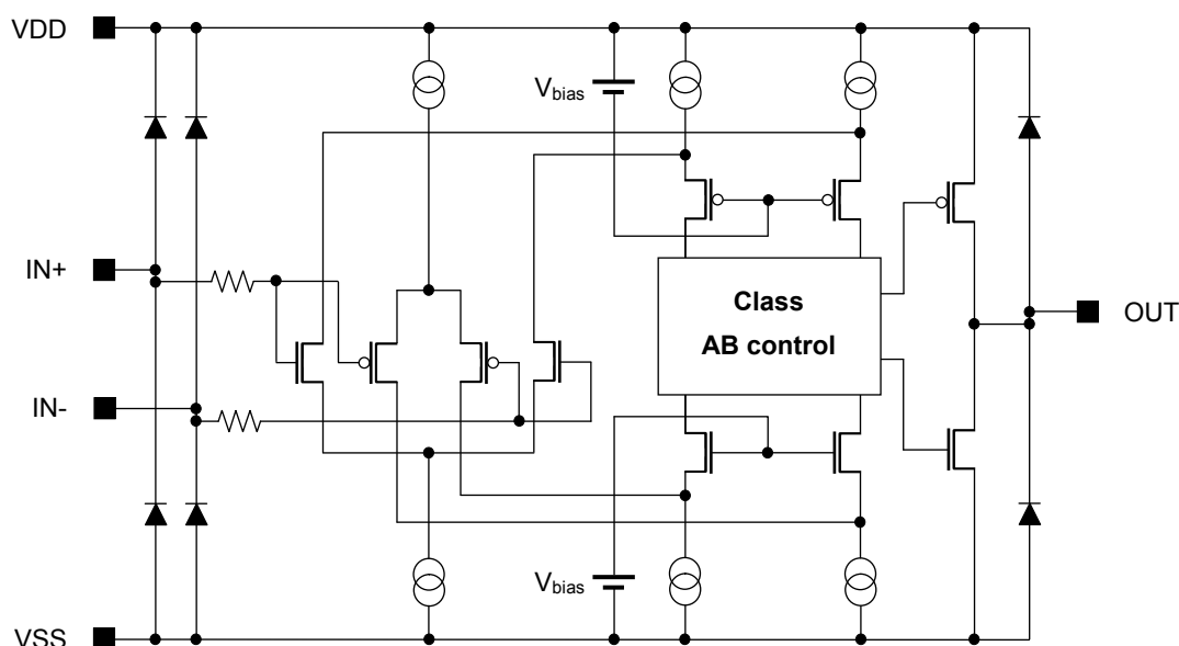
Figure 1. 内部等価回路図(1 チャンネルのみ)
