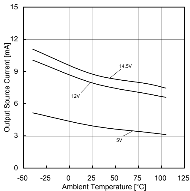
Figure 34. 出力ソース電流 vs 温度特性 (OUT=VDD-0.4V)
