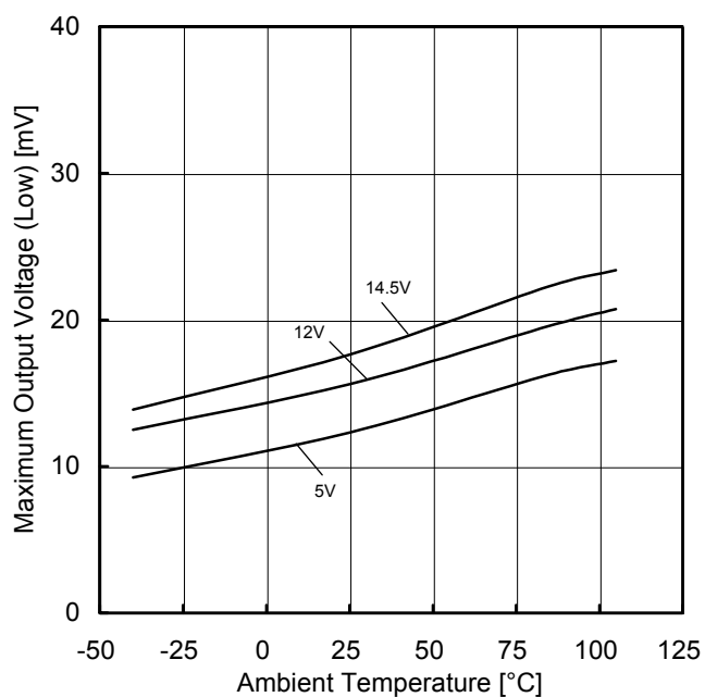
Figure 9. 最大出力電圧(Low) vs 温度特性 ( R_L=10k\Omega )
