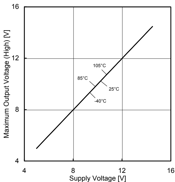
Figure 6. 最大出力電圧(High) vs 電源電圧特性 ( R_L=10k\Omega )
