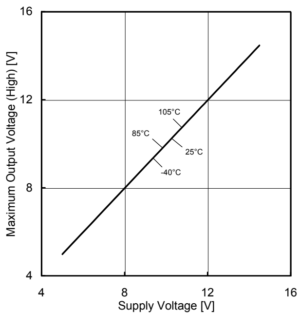
Figure 29. 最大出力電圧(High) vs 電源電圧特性 ( R_L=10k\Omega )
