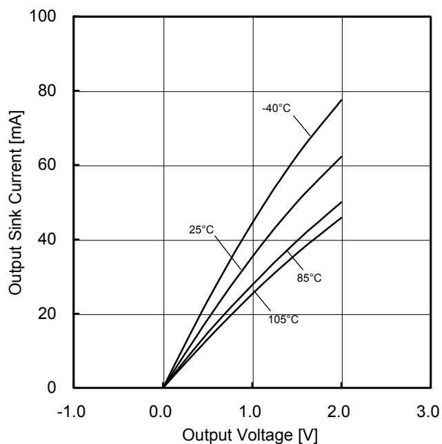
Figure 35. 出力シンク電流 vs 出力電圧特性 (VDD=3V)
