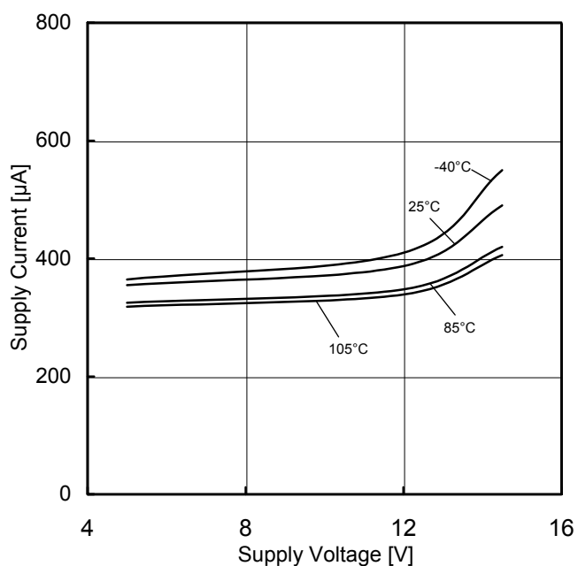
Figure 4. 回路電流 vs 電源電圧特性
