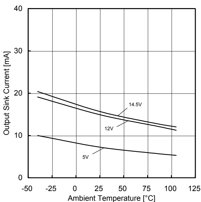
Figure 36. 出力シンク電流 vs 温度特性 (OUT=VSS+0.4V)
