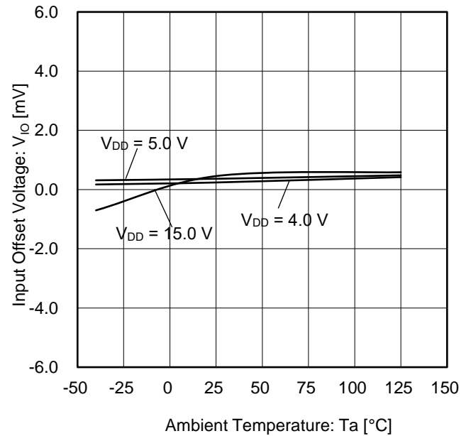
Figure 12. 入力オフセット電圧 vs 温度 ( V_{ICM} = V_{DD}/2, E_K = -V_{DD}/2 )
