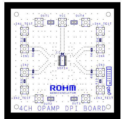
Figure 24. EMI 特性評価ボード (BD87524YFV-C)
