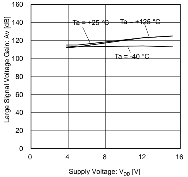
Figure 14. 大振幅電圧利得 vs 電源電圧
