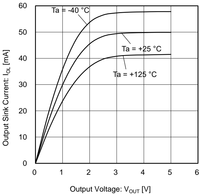
Figure 9. 出力シンク電流 vs 出力電圧 ( V_{DD} = 5\text{ V} )
