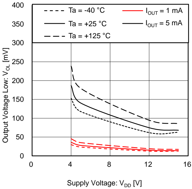
Figure 5. 出力電圧 Low vs 電源電圧
