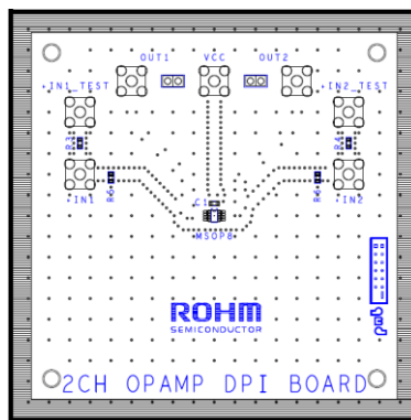
Figure 23. EMI 特性評価ボード (BD87522YFJ-C, BD87522YFVM-C)
