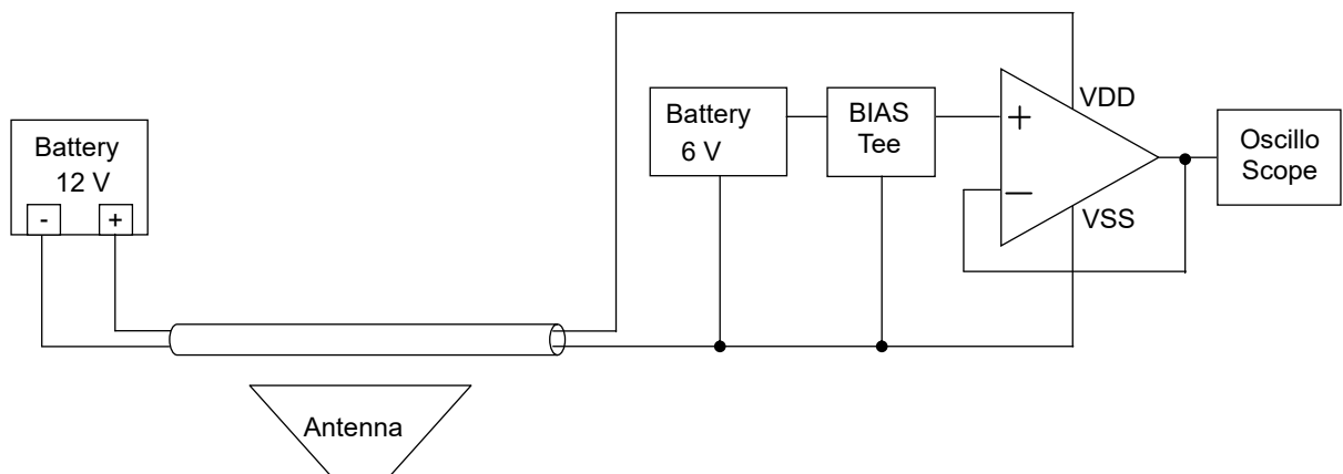
Figure 25. EMI 特性測定回路図
