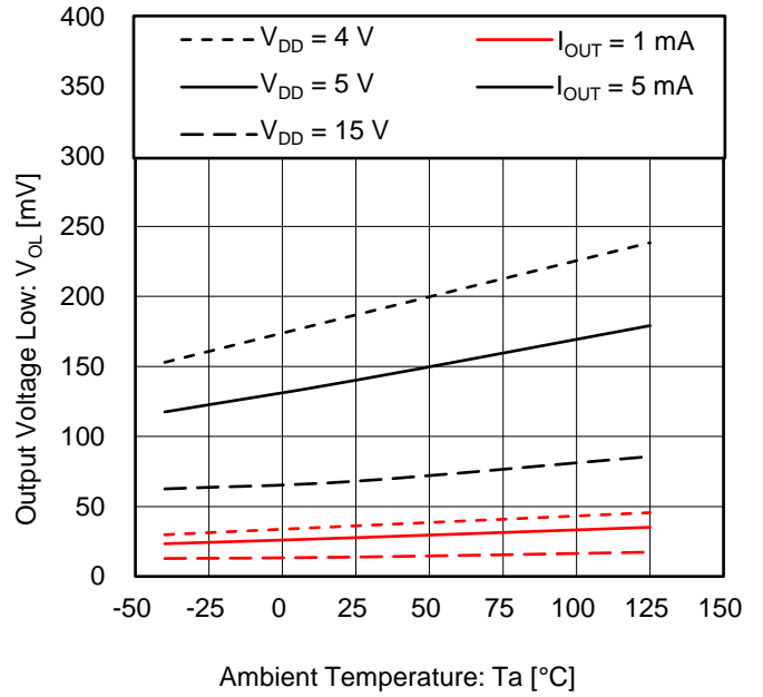
Figure 6. 出力電圧 Low vs 温度
