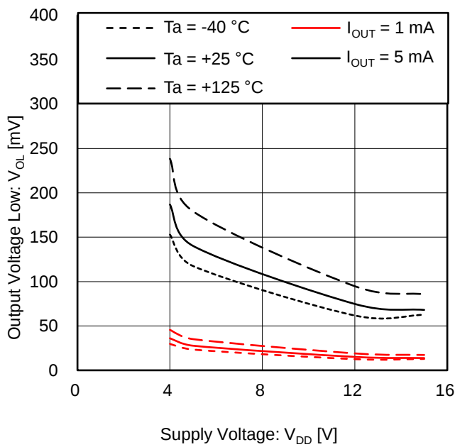
Figure 5. 出力電圧 Low vs 電源電圧
