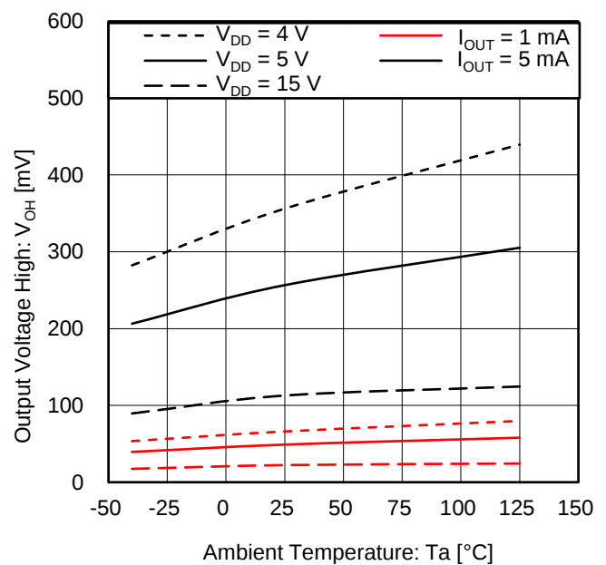
Figure 4. 出力電圧 High vs 温度 ( V_{OH} = V_{DD} - V_{OUT} )
