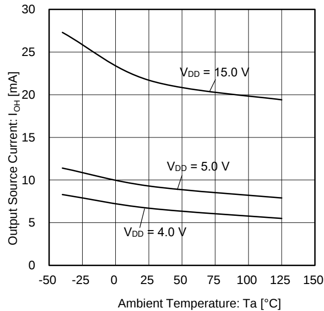
Figure 8. 出力ソース電流 vs 温度 ( V_{OUT} = V_{DD} - 0.5\text{ V} )
