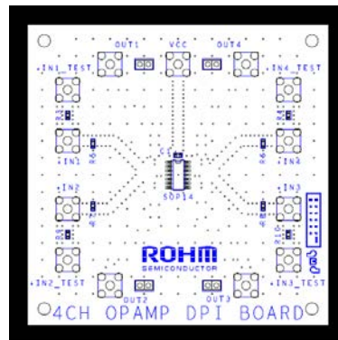
Figure 22. EMI 特性評価ボード (BD87554YFV-C)
