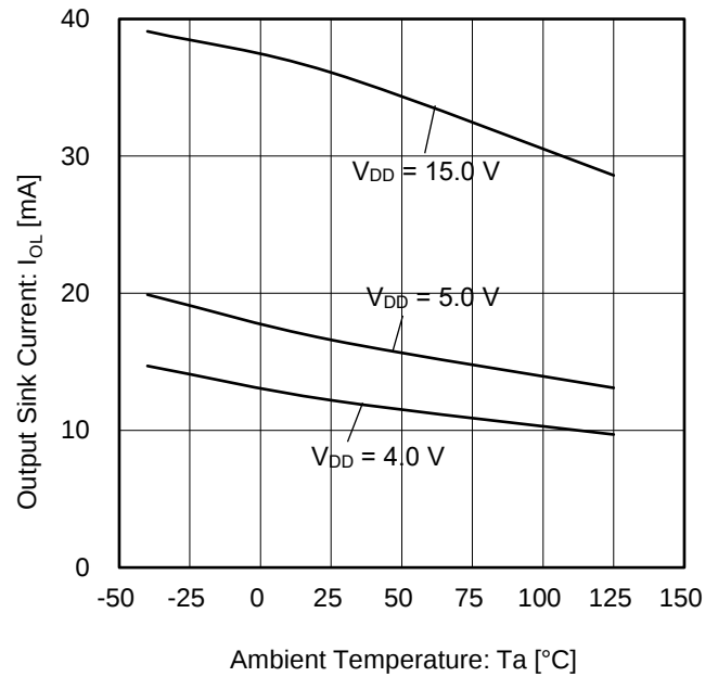
Figure 10. 出力シンク電流 vs 温度 ( V_{OUT} = V_{SS} + 0.5\text{ V} )
