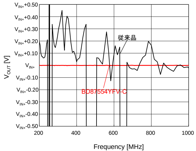
Figure 21. EMI 特性データ
