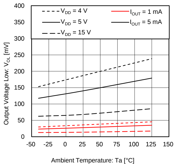
Figure 6. 出力電圧 Low vs 温度
