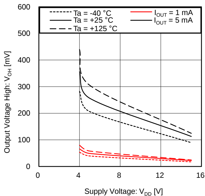
Figure 3. 出力電圧 High vs 電源電圧 ( V_{OH} = V_{DD} - V_{OUT} )
