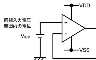
Figure 24. 未使用回路の処理例
