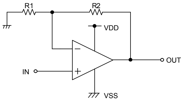
Figure 77. 非反転増幅回路
