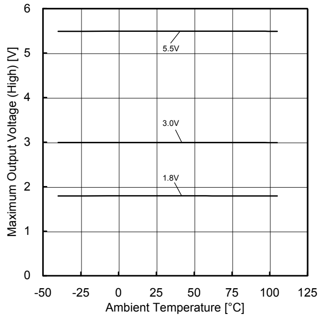
Figure 53. 最大出力電圧(High)－温度特性 ( R_L = 10k\Omega )
