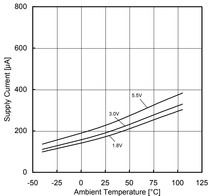
Figure 28. 回路電流－温度特性
