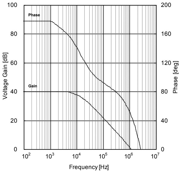
Figure 70. 電圧利得/位相－周波数特性
