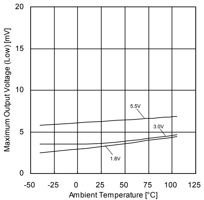
Figure 55. 最大出力電圧(Low)－温度特性 ( R_L = 10k\Omega )
