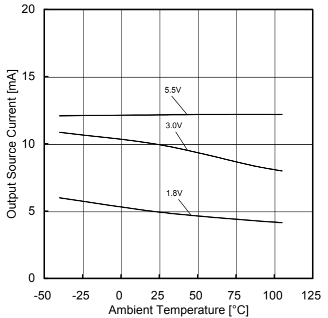
Figure 11. 出カソース電流－温度特性 (OUT=VDD-0.4V)
