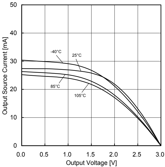
Figure 10. 出カソース電流－出力電圧特性 (VDD=3V)
