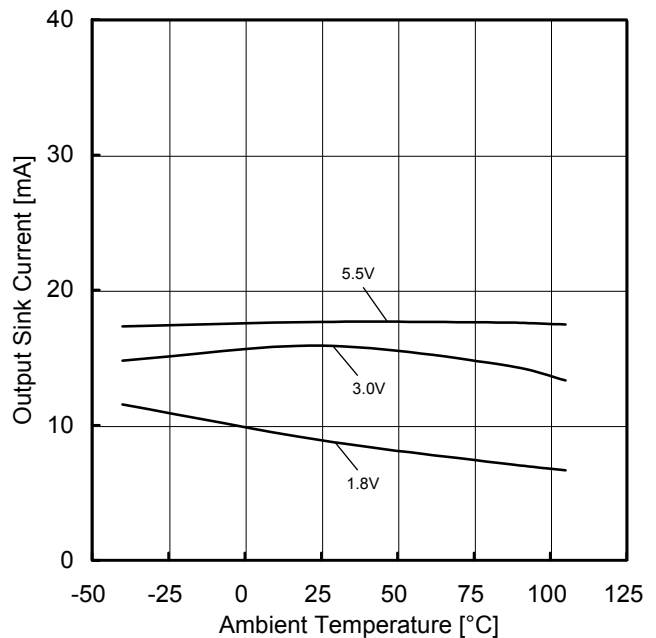
Figure 13. 出カシンク電流－温度特性 (OUT=VSS+0.4V)
