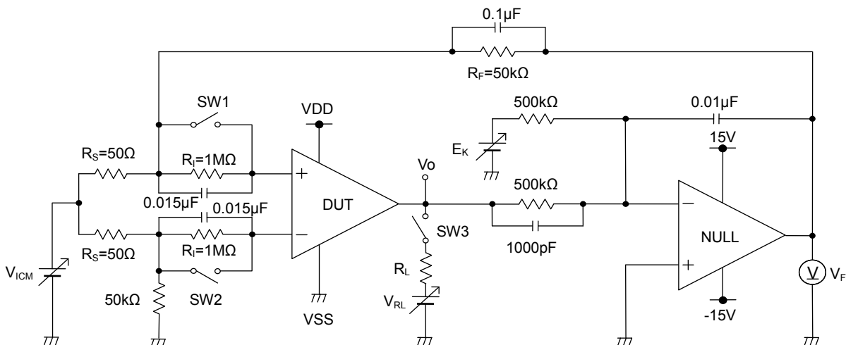
Figure 71. 測定回路 1(1 チャンネルのみ)
