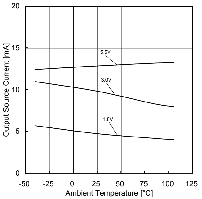
Figure 34. 出力シンク電流－温度特性 (OUT=VDD-0.4V)
