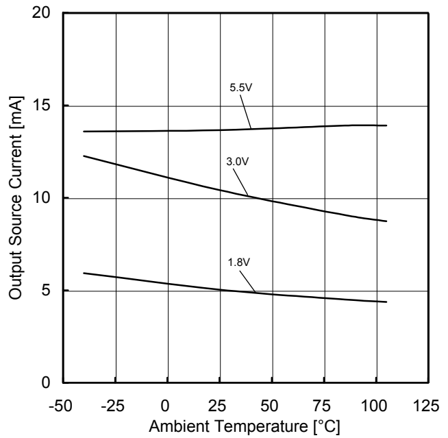
Figure 57. 出力ソース電流－温度特性 (OUT=VDD-0.4V)
