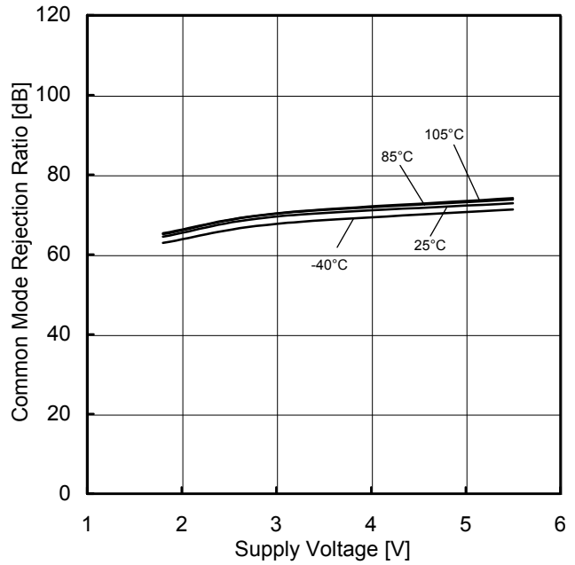
Figure 65. 同相信号除去比－電源電圧特性
