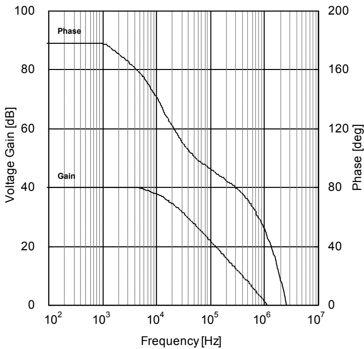
Figure 24. 電圧利得/位相–周波数特性
