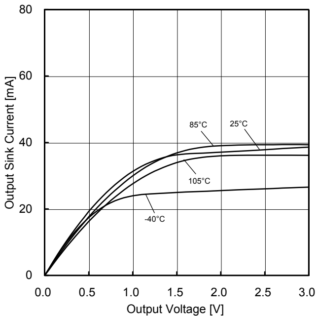
Figure 12. 出カシンク電流－出力電圧特性 (VDD=3V)
