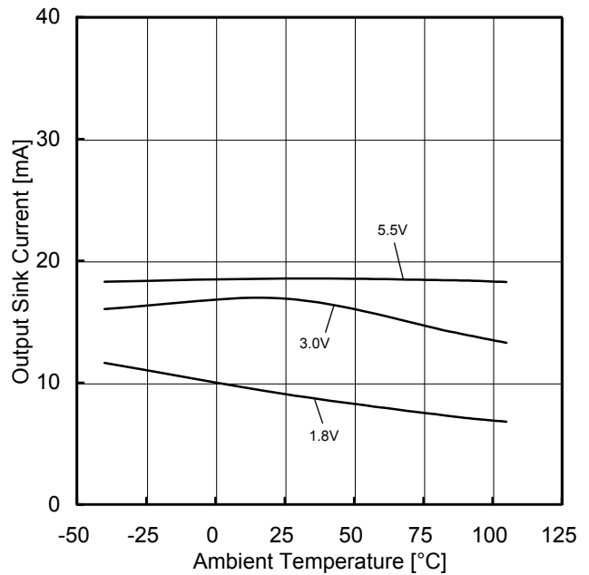
Figure 36. 出力シンク電流－温度特性 (OUT=VSS+0.4V)
