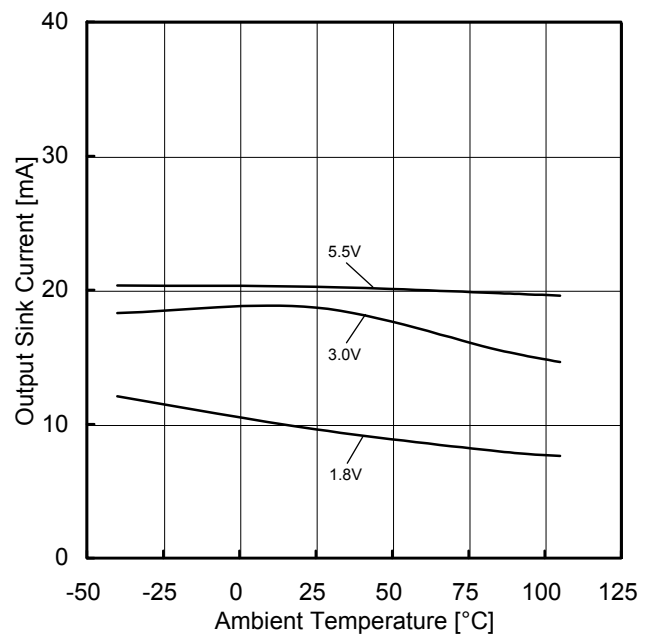
Figure 59. 出力シンク電流－温度特性 (OUT=VSS+0.4V)
