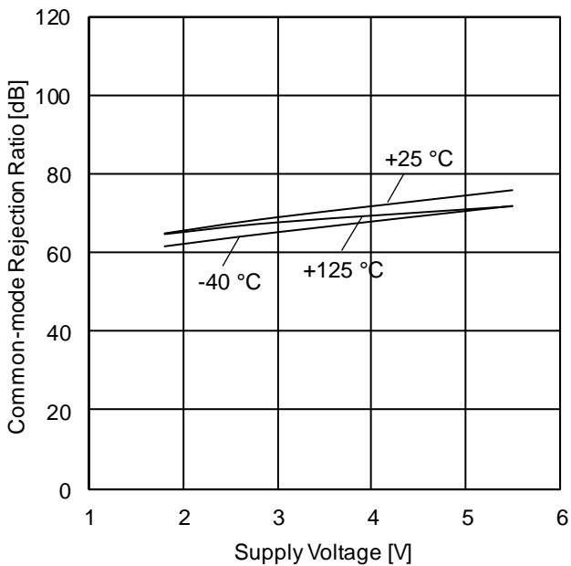
Figure 24. 同相信号除去比 vs 電源電圧特性
