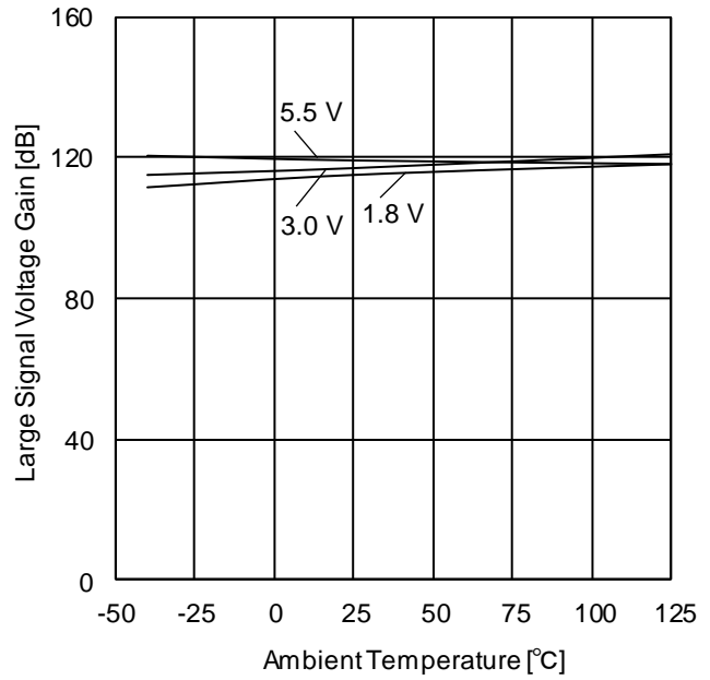
Figure 23. 大振幅電圧利得 vs 温度特性
