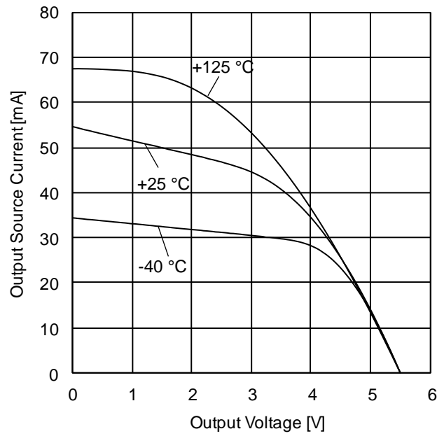
Figure 11. 出カソース電流 vs 出力電圧特性 ( V_{DD}=5.5\text{ V} )
