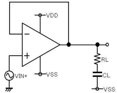
Figure 39. 周波数特性改善回路例 2
