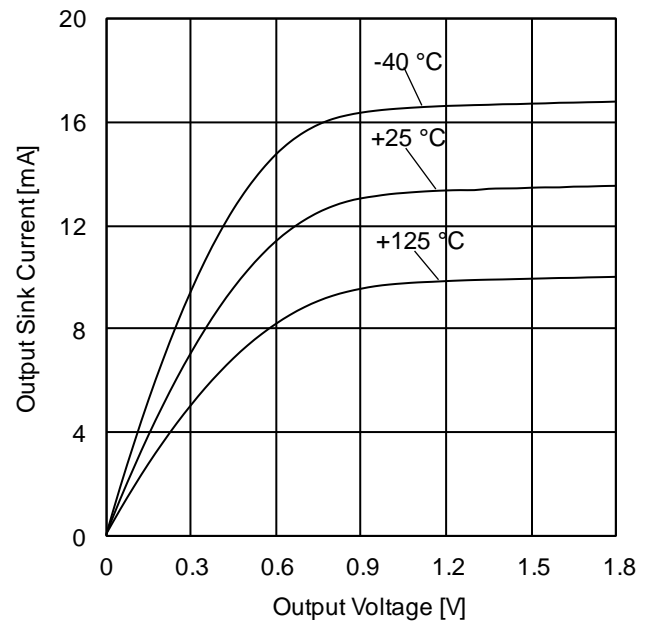
Figure 13. 出カシンク電流 vs 出力電圧特性 ( V_{DD}=1.8\text{ V} )
