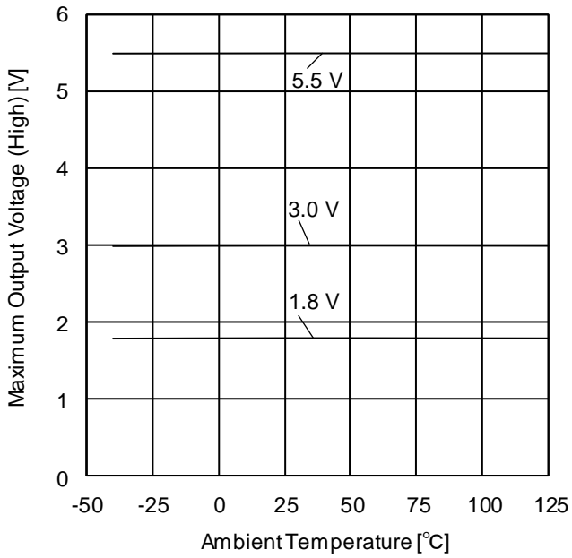
Figure 6. 最大出力電圧(High) vs 温度特性 (R L =10 kΩ)
