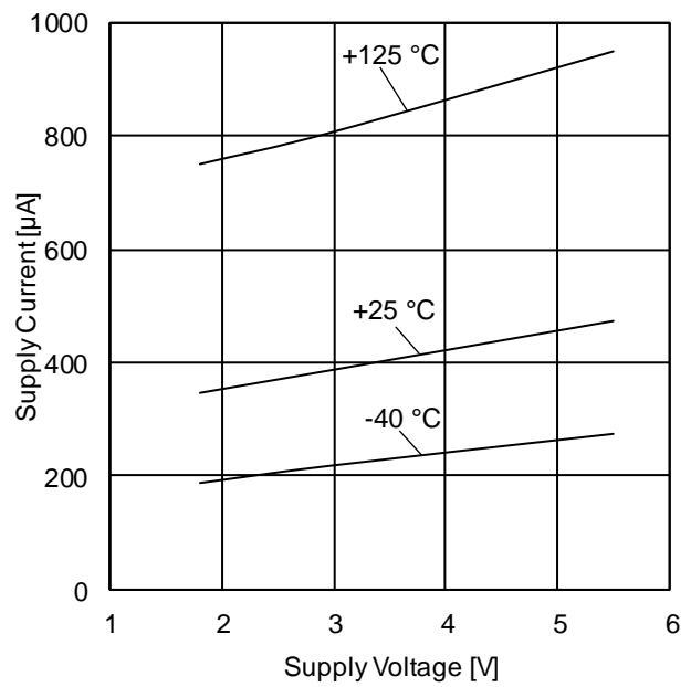
Figure 3. 回路電流 vs 電源電圧特性
