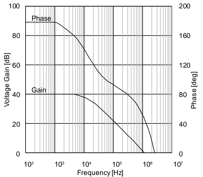
Figure 29. 電圧利得・位相 vs 周波数特性 (V DD =3.0 V)
