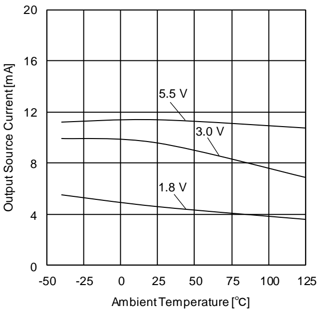
Figure 12. 出カソース電流 vs 温度特性 ( V_{OUT}=V_{DD}-0.4\text{ V} )
