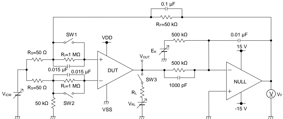
Figure 30. 測定回路 1
