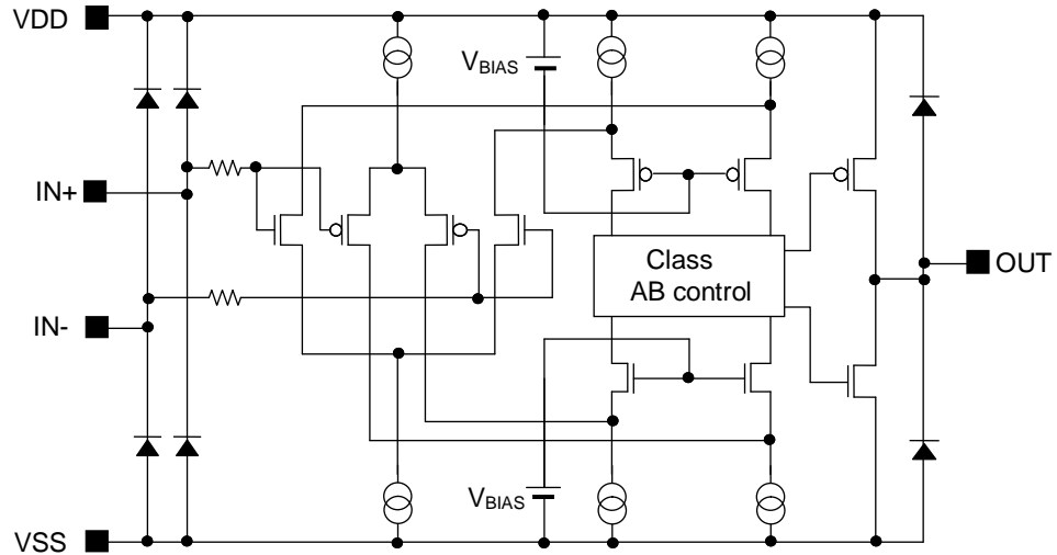
Figure 1. ブロック図
