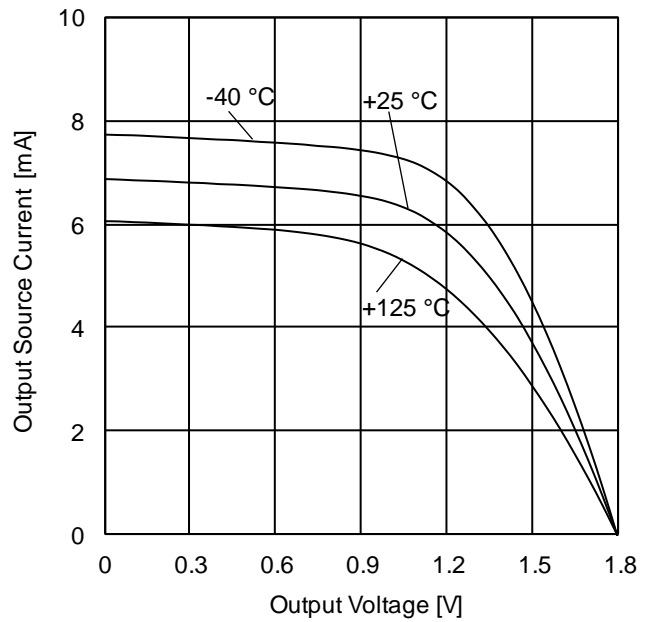
Figure 9. 出力ソース電流 vs 出力電圧特性 (V DD =1.8 V)
