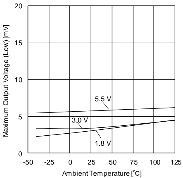
Figure 8. 最大出力電圧(Low) vs 温度特性 (R L =10 kΩ)
