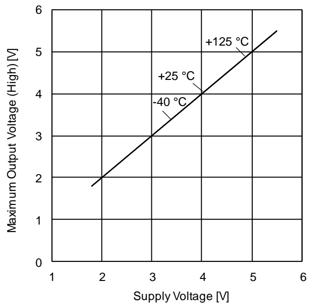
Figure 5. 最大出力電圧(High) vs 電源電圧特性 (R L =10 kΩ)
