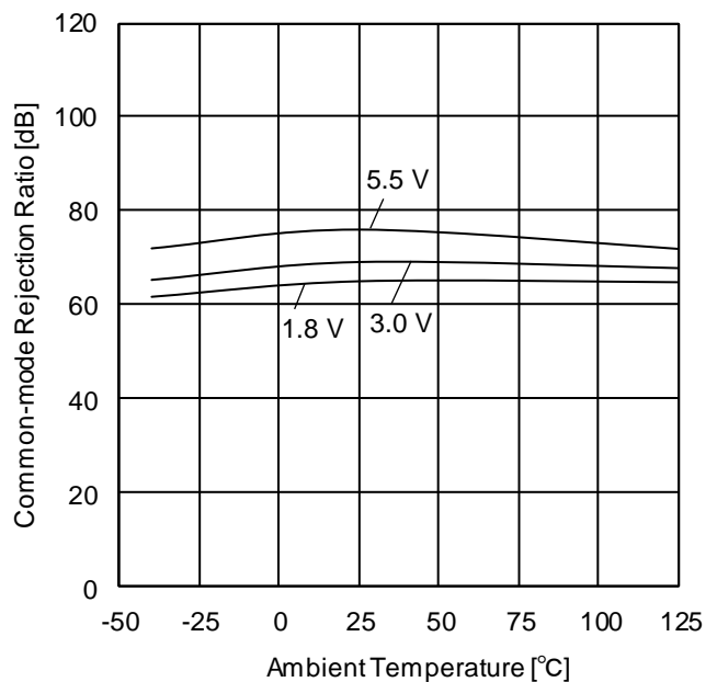
Figure 25. 同相信号除去比 vs 温度特性
