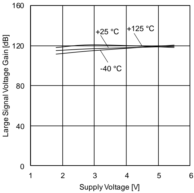
Figure 22. 大振幅電圧利得 vs 電源電圧特性
