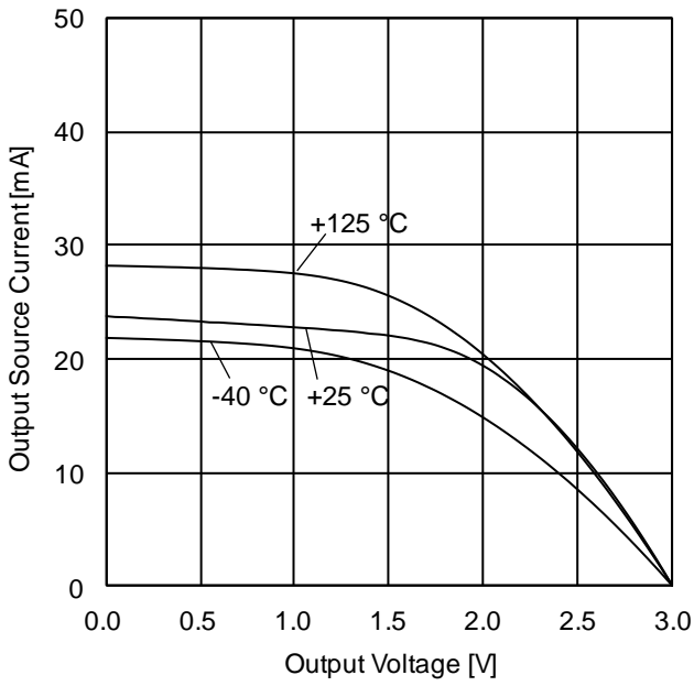
Figure 10. 出カソース電流 vs 出力電圧特性 ( V_{DD}=3.0\text{ V} )
