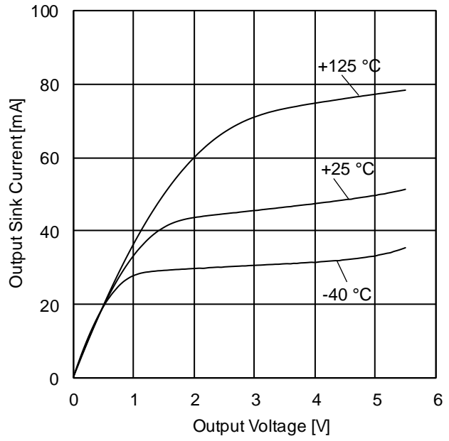
Figure 15. 出力シンク電流 vs 出力電圧特性 ( V_{DD}=5.5\text{ V} )
