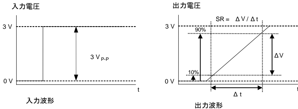
Figure 32. スルーレート
