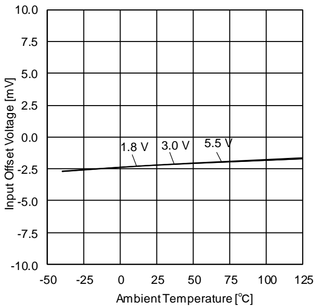
Figure 18. 入力オフセット電圧 vs 温度特性 ( V_{ICM}=V_{DD} , E_K=-V_{DD}/2 )
