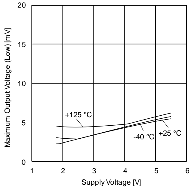
Figure 7. 最大出力電圧(Low) vs 電源電圧特性 (R L =10 kΩ)
