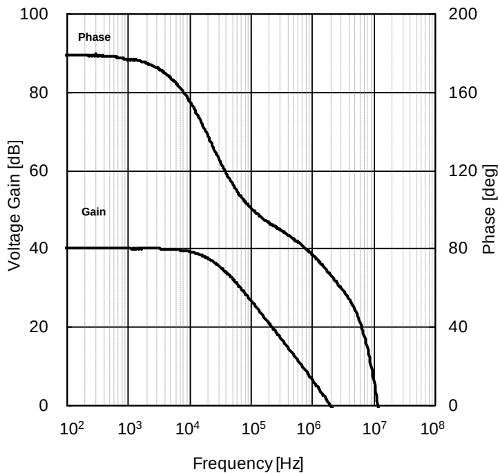
Figure 47. 電圧利得・位相一周波数特性
