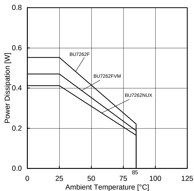
Figure 25. ディレーティングカーブ
