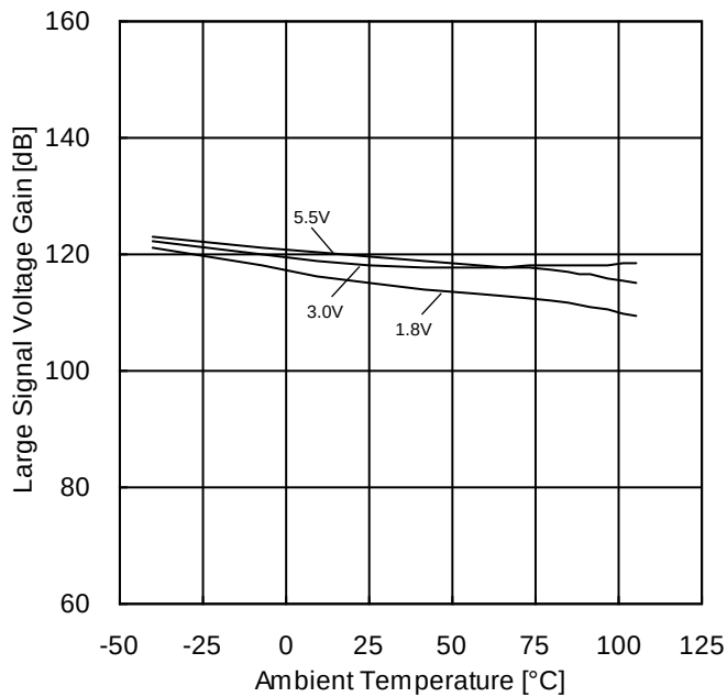
Figure 64. 大振幅電圧利得－温度特性
