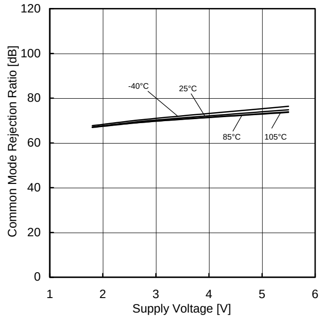
Figure 65. 同相信号除去比－電源電圧特性
