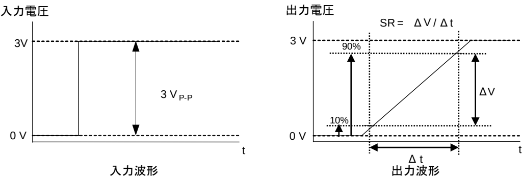
Figure 73. スルーレート測定時
