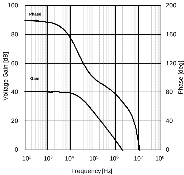
Figure 70. 電圧利得・位相一周波数特性
