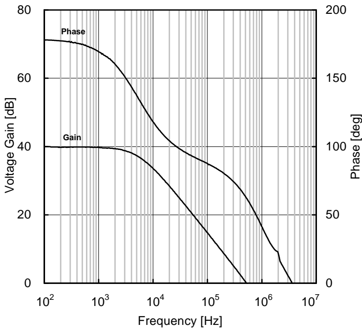
Figure 23. 電圧利得・位相一周波数特性
