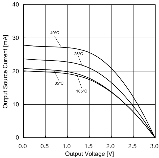
Figure 9. 出力ソース電流－出力電圧特性 (VDD=3V)
