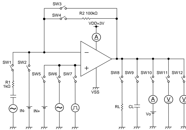
Figure 25. 測定回路 2
