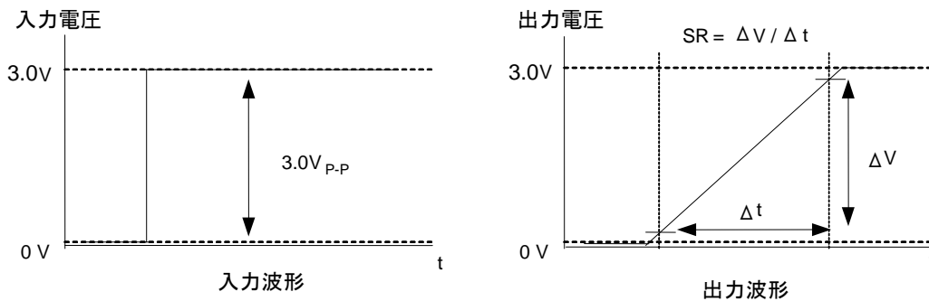
Figure 26. スルーレート測定時 入出力波形
