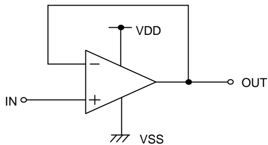
Figure 27. ボルテージフォロワ回路
