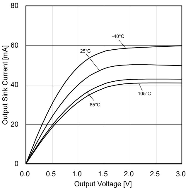
Figure 58. 出カシンク電流-出力電圧特性 (VDD=3V)
