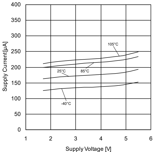
Figure 50. 回路電流-電源電圧特性
