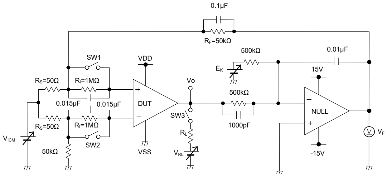
Figure 71. 測定回路 1(1チャンネルのみ)
