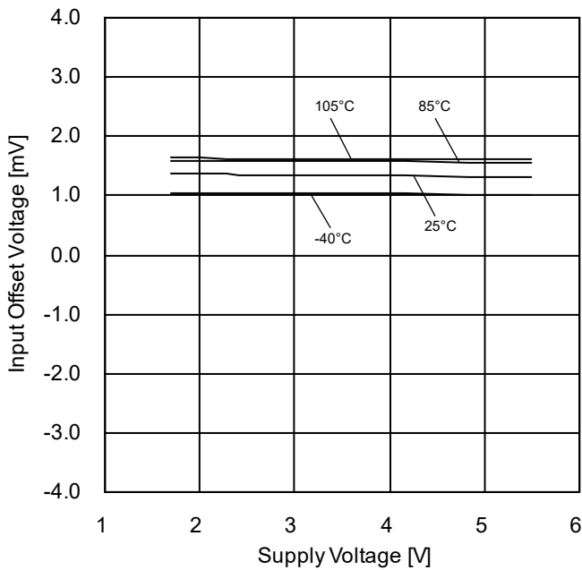
Figure 37. 入力オフセット電圧-電源電圧特性 ( V_{ICM}=V_{DD}-1.2V , E_k = -V_{DD}/2 )
