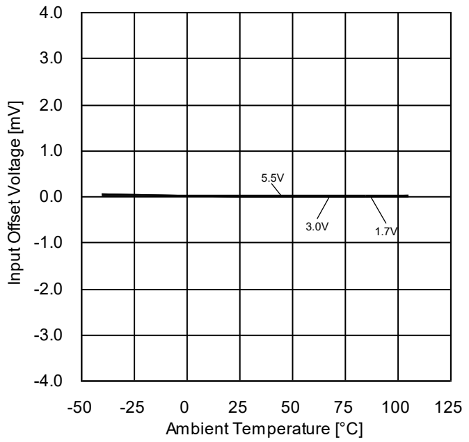
Figure 61. 入力オフセット電圧-温度特性 ( V_{ICM}=V_{DD}-1.2V , E_k = -V_{DD}/2 )
