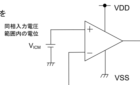
Figure 79. 未使用回路処理例
