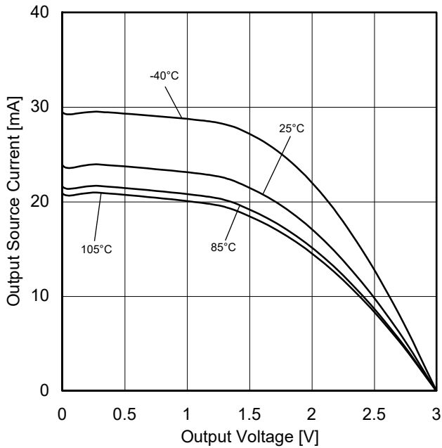
Figure 56. 出カソース電流-出力電圧特性 (VDD=3 V)
