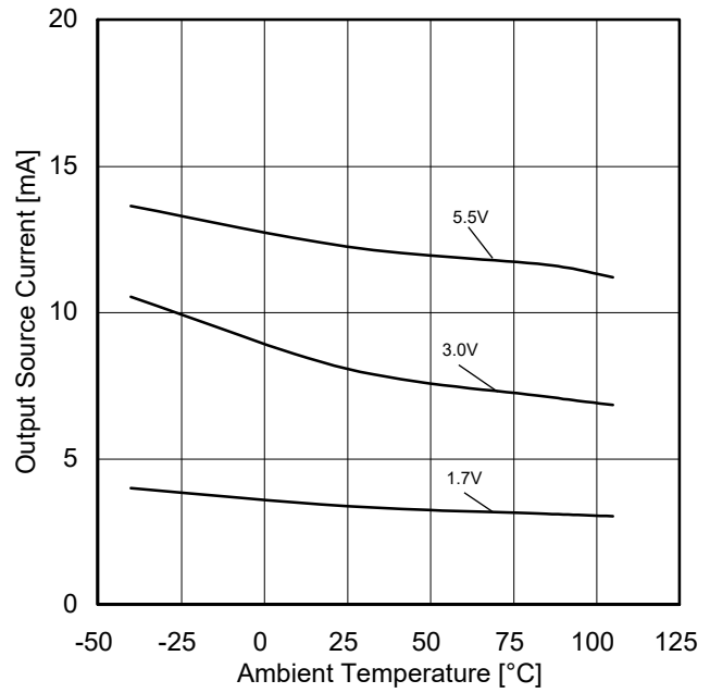
Figure 57. 出カソース電流-温度特性 (OUT=VDD-0.4V)
