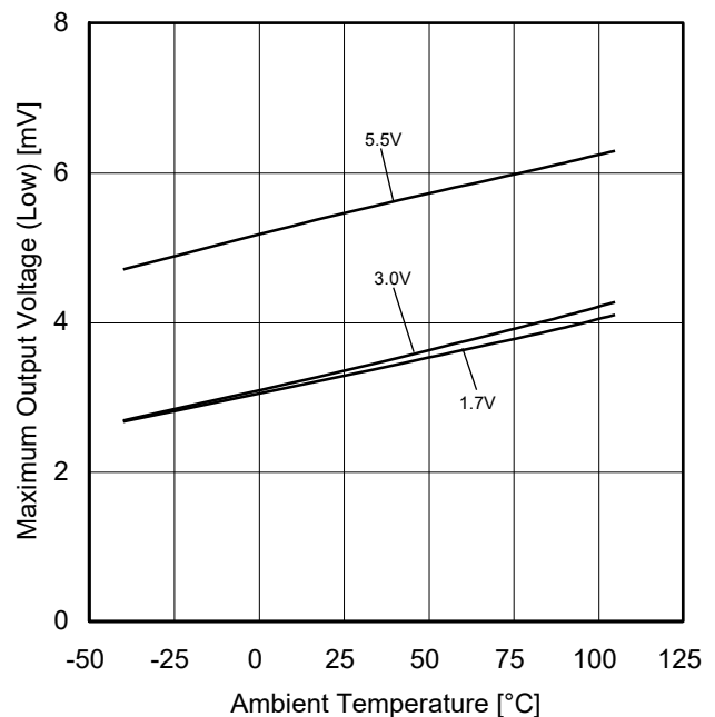
Figure 55. 最大出力電圧(Low)－温度特性 ( R_L=10k\Omega )
