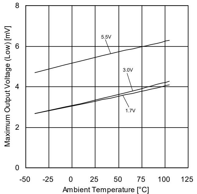
Figure 32. 最大出力電圧(Low)－温度特性 ( R_L=10k\Omega )
