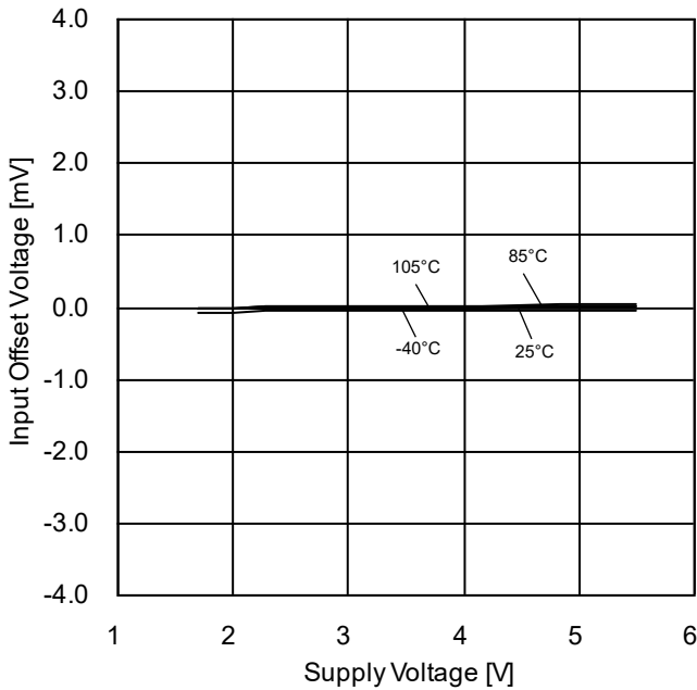
Figure 60. 入力オフセット電圧-電源電圧特性 ( V_{ICM}=V_{DD}-1.2V , E_k = -V_{DD}/2 )
