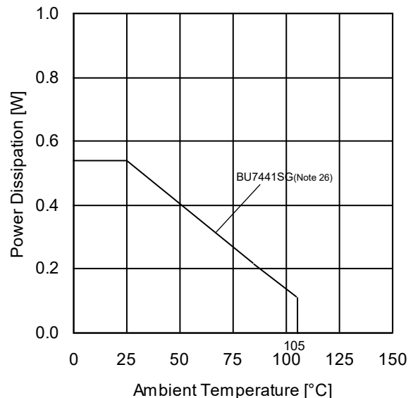
(d) BU7441SG
