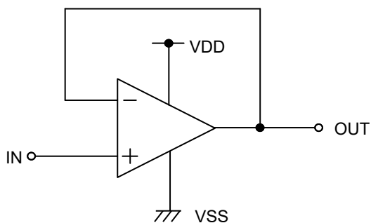
Figure 75. ボルテージフォロア回路
