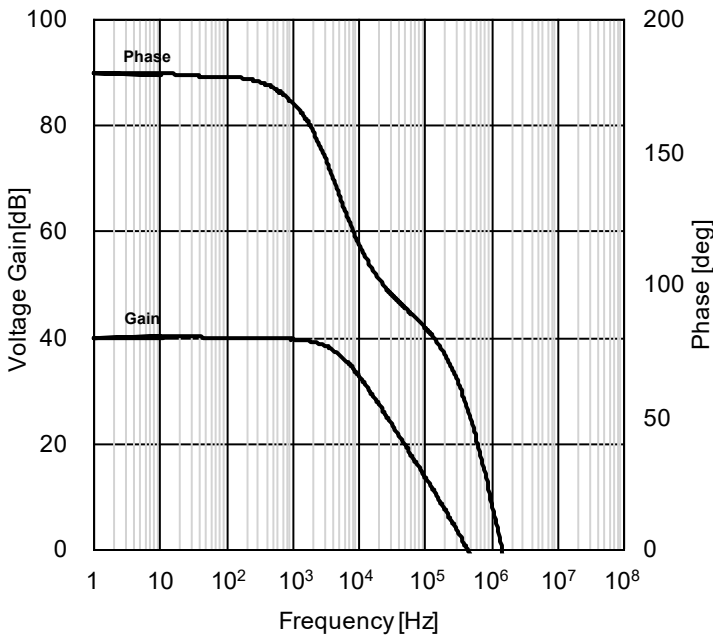
Figure 47. 電圧利得・位相一周波数特性 (VDD=+3V, VSS=0V, T A =25°C)
