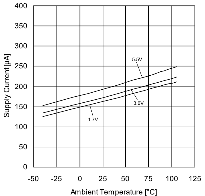
Figure 51. 回路電流-温度特性
