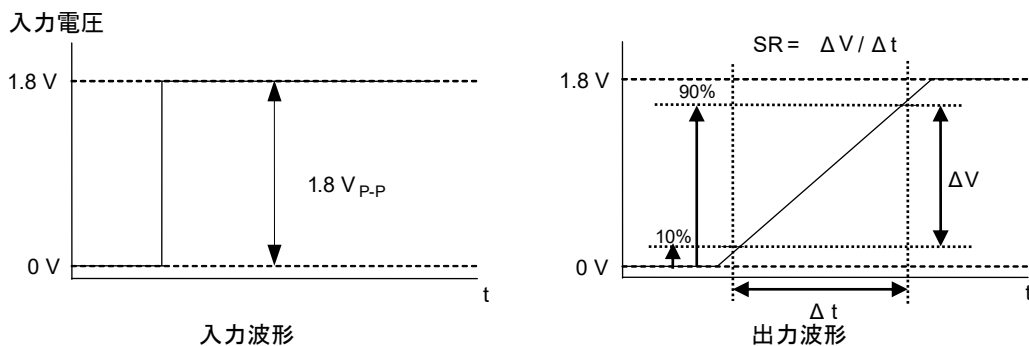
Figure 73. スルーレート測定時 入出力波形
