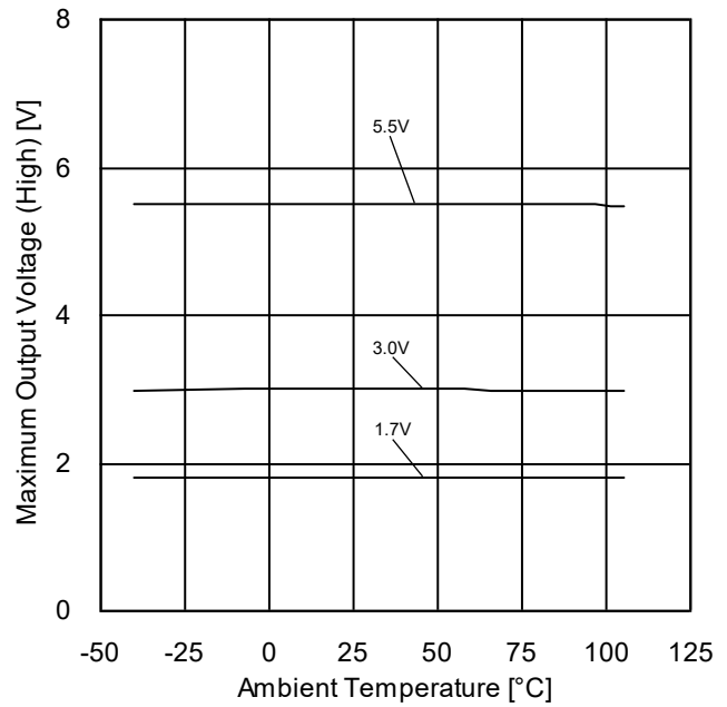
Figure 30. 最大出力電圧(High)－温度特性 ( R_L=10k\Omega )
