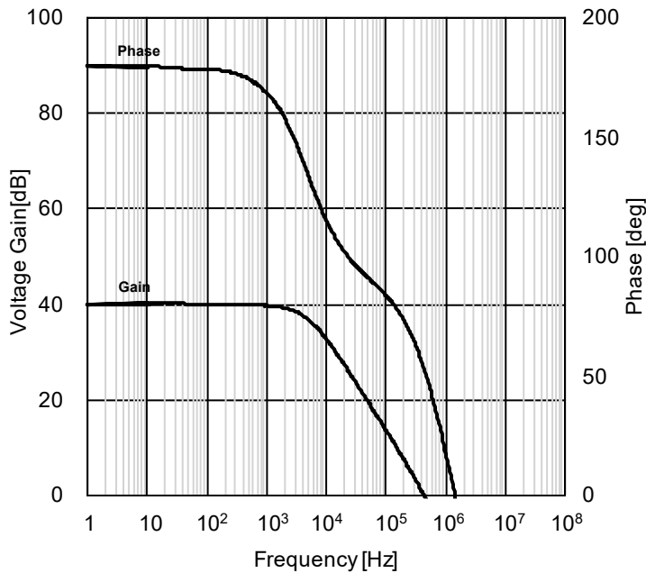
Figure 70. 電圧利得・位相-周波数特性 (VDD=+3V, VSS=0V, T A =25°C)
