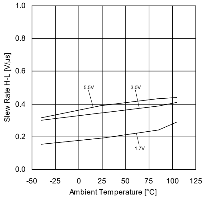
Figure 69. スルーレート(H-L)-温度特性
