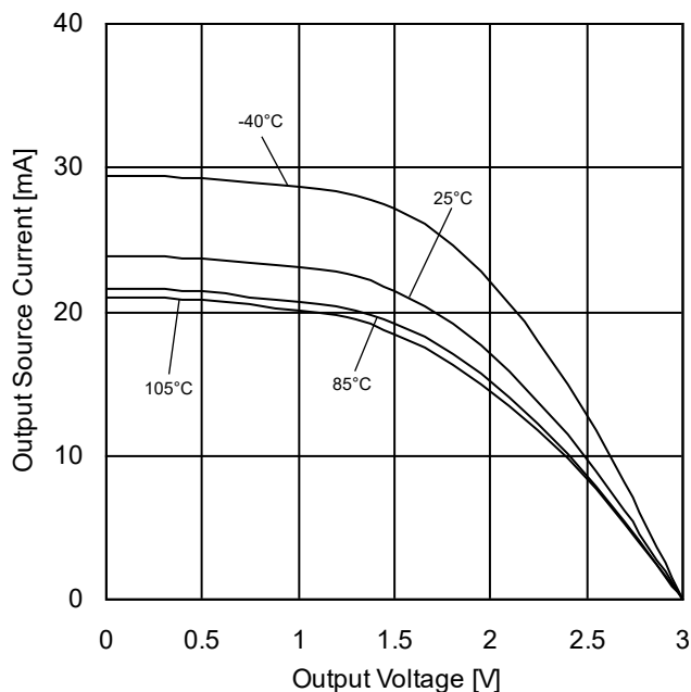
Figure 33. 出力ソース電流-出力電圧特性 (VDD=3V)
