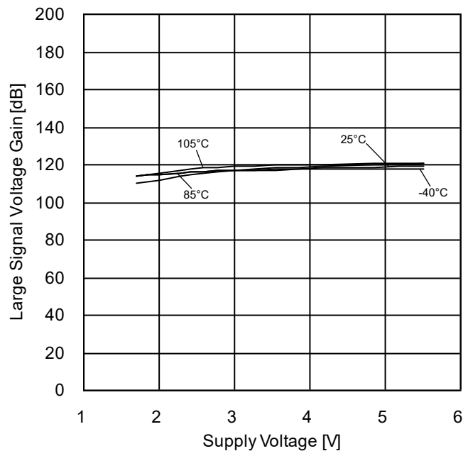
Figure 63. 大振幅電圧利得-電源電圧特性
