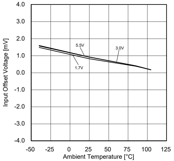
Figure 15. 入力オフセット電圧-温度特性 ( V_{ICM}=V_{DD}-1.2V , E_k = -V_{DD}/2 )
