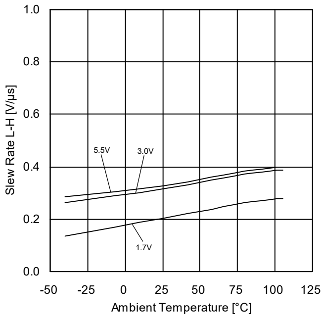
Figure 68. スルーレート(L-H)-温度特性
