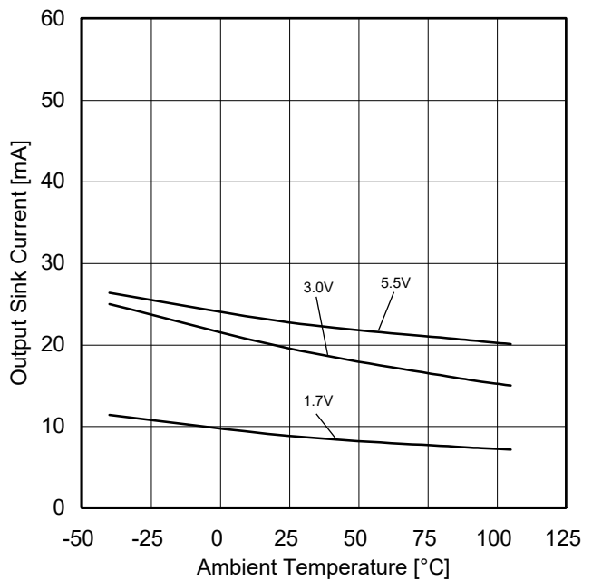
Figure 59. 出カシンク電流-温度特性 (OUT=VSS+0.4V)
