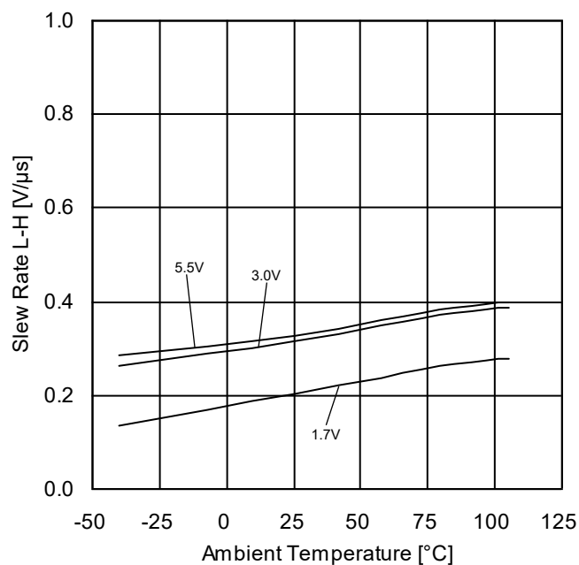
Figure 22. スルーレート(L-H)-温度特性
