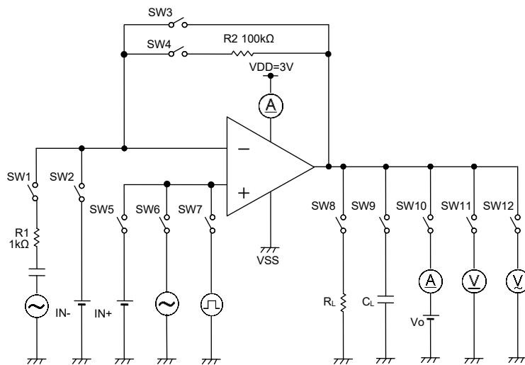
Figure 72. 測定回路例 2 (片チャンネルのみ)
