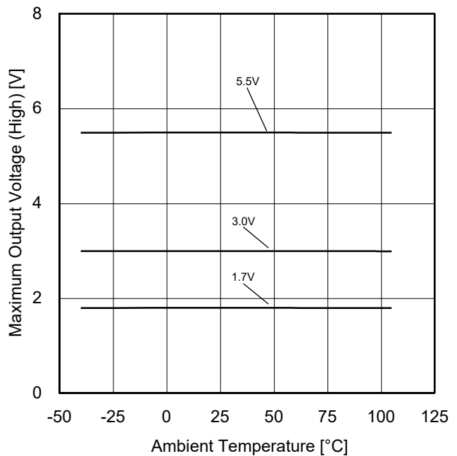
Figure 53. 最大出力電圧(High)－温度特性 ( R_L=10k\Omega )
