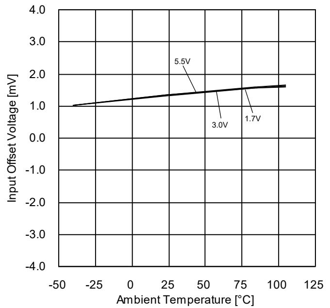
Figure 38. 入力オフセット電圧-温度特性 ( V_{ICM}=V_{DD}-1.2V , E_k = -V_{DD}/2 )
