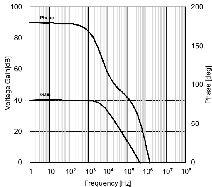
Figure 24. 電圧利得・位相一周波数特性 (VDD=+3V, VSS=0V, TA=25°C)
