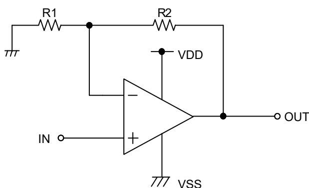
Figure 77. 非反転増幅回路
