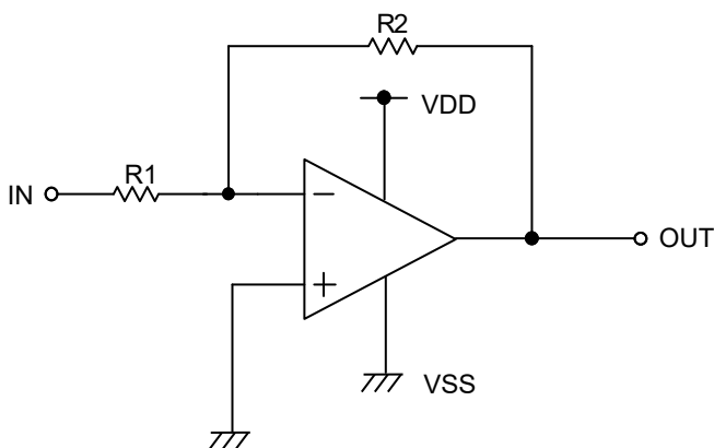
Figure 76. 反転増幅回路
