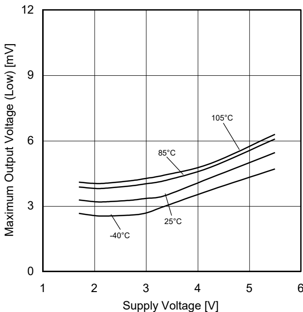
Figure 54. 最大出力電圧(Low)－電源電圧特性 ( R_L=10k\Omega )
