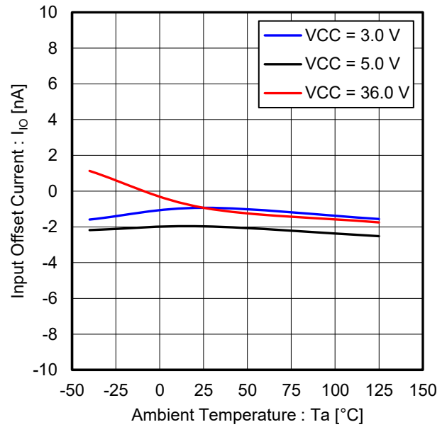
Figure 18. 入力オフセット電流 vs 温度 ( V_{ICM} = V_{CC}/2 )
