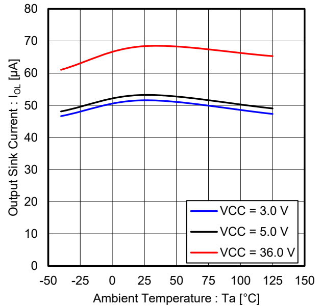
Figure 10. 出力シンク電流 vs 温度 ( V_{OUT} = 0.2\text{ V} )
