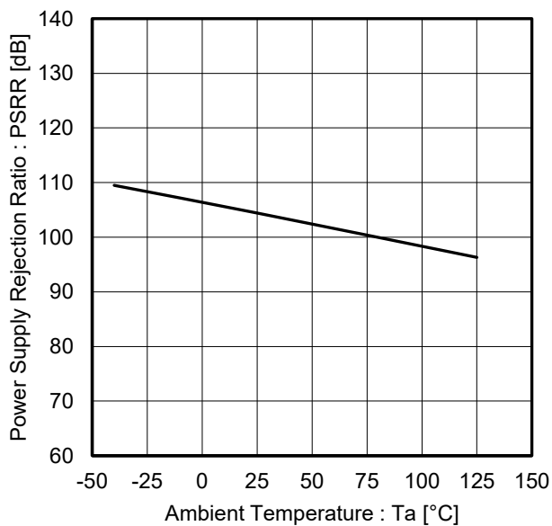
Figure 23. 電源電圧除去比 vs 温度 ( V_{CC} = 5\text{ V} )
