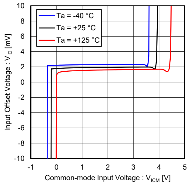
Figure 16. 入力オフセット電圧 vs 同相入力電圧 ( V_{CC} = 5\text{ V} )
