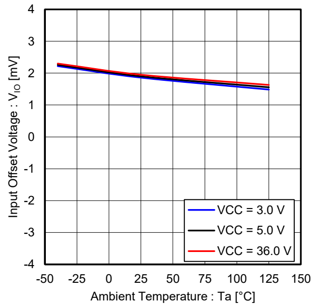
Figure 12. 入力オフセット電圧 vs 温度 ( V_{ICM} = V_{CC}/2 )
