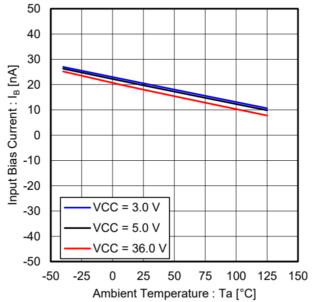
Figure 14. 入力バイアス電流 vs 温度 ( V_{ICM} = V_{CC}/2 )
