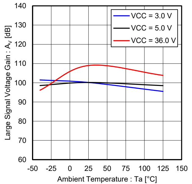
Figure 20. 大振幅電圧利得 vs 温度 ( R_L = 2\text{ k}\Omega )
