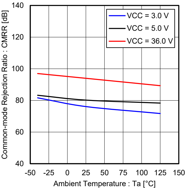
Figure 22. 同相信号除去比 vs 温度 ( V_{OUT} = 1.4\text{ V} )
