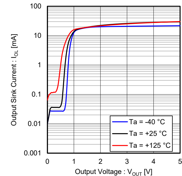
Figure 7. 出力シンク電流 vs 出力電圧 ( V_{CC} = 5\text{ V} )
