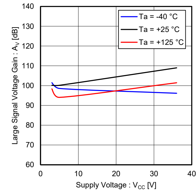
Figure 19. 大振幅電圧利得 vs 電源電圧 ( R_L = 2\text{ k}\Omega )
