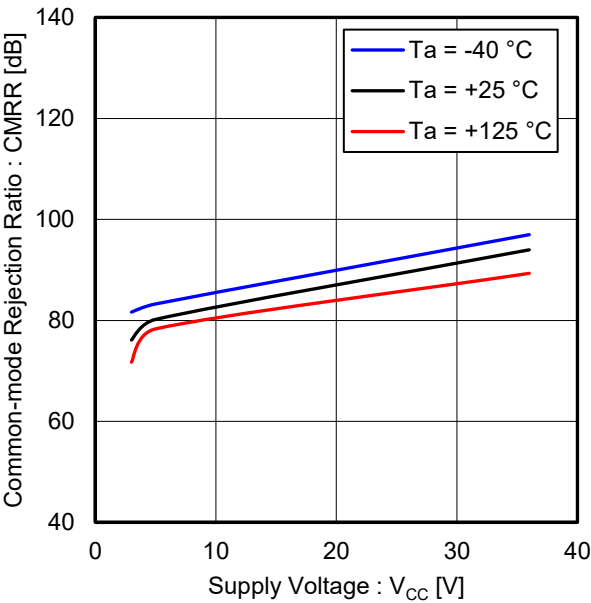
Figure 21. 同相信号除去比 vs 電源電圧 ( V_{OUT} = 1.4\text{ V} )
