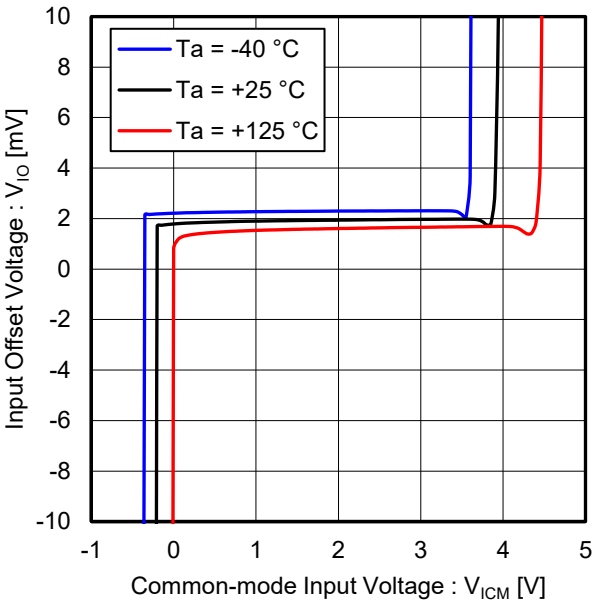
Figure 16. 入力オフセット電圧 vs 同相入力電圧 ( V_{CC} = 5\text{ V} )
