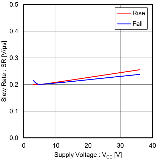
Figure 24. スルーレート vs 電源電圧 ( T_a = 25\text{ }^{\circ}\text{C} , R_L = 2\text{ k}\Omega )
