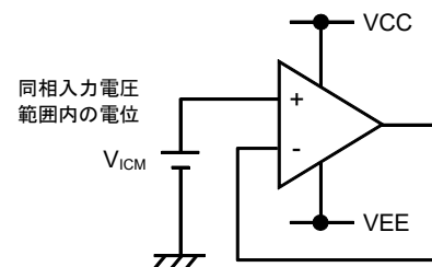
Figure 26. 未使用回路の処理例
