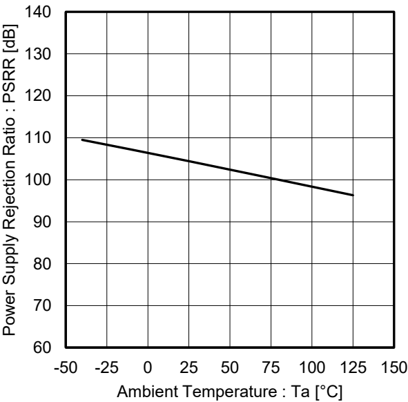
Figure 23. 電源電圧除去比 vs 温度 ( V_{CC} = 5\text{ V} )
