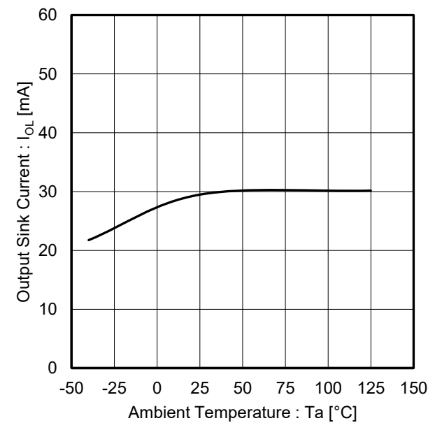
Figure 8. 出力シンク電流 vs 温度 ( V_{CC} = 5\text{ V} , V_{OUT} = 5\text{ V} )
