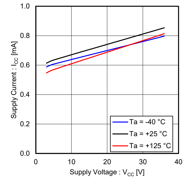
Figure 1. 回路電流 vs 電源電圧
