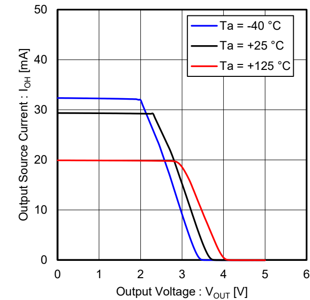
Figure 5. 出力ソース電流 vs 出力電圧 ( V_{CC} = 5\text{ V} )
