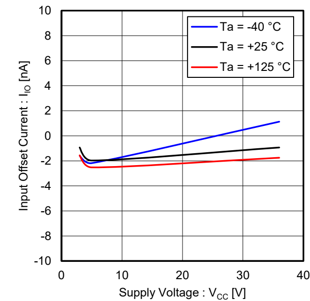
Figure 17. 入力オフセット電流 vs 電源電圧 ( V_{ICM} = V_{CC}/2 )
