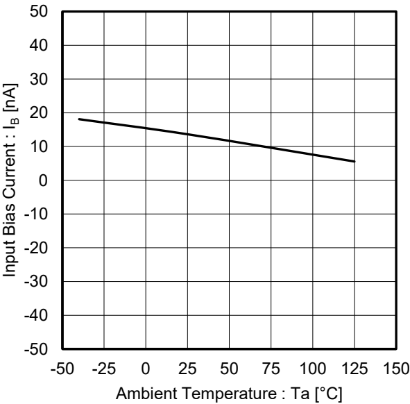
Figure 15. 入力バイアス電流 vs 温度 ( V_{CC} = 30\text{ V} , V_{ICM} = 28\text{ V} , V_{OUT} = 1.4\text{ V} )
