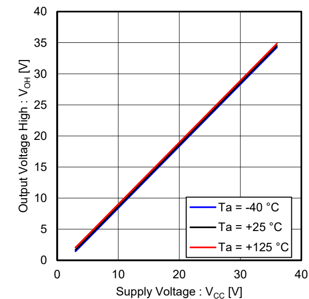
Figure 3. 出力電圧 High vs 電源電圧 ( R_L = 10\text{ k}\Omega )
