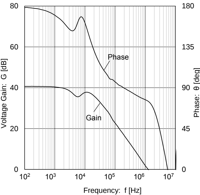
Figure 31. 電圧利得・位相 vs 周波数 ( V_S = 2.7\text{ V} )
