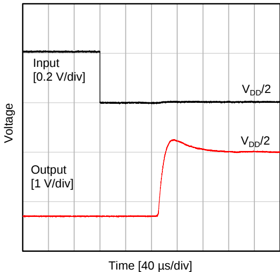
Figure 35. オーバーロードリカバリ ( V_S = 2.7\text{ V} , G = 40\text{ dB} , V_{IN} = (V_{DD}/2 + 0.2\text{ V}) to V_{DD}/2 )
