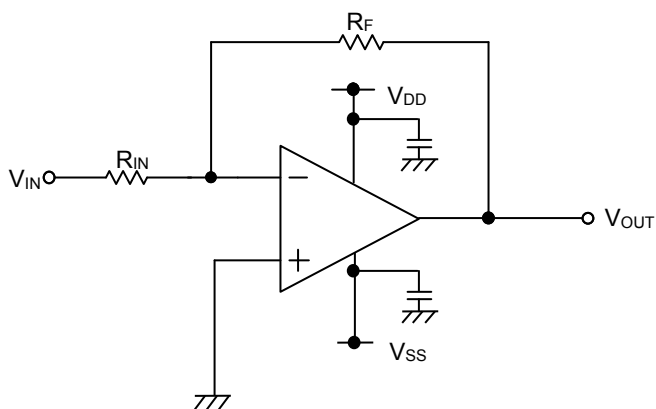
Figure 40. 反転増幅回路
