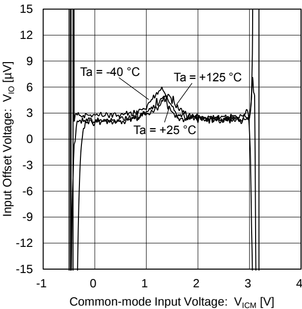
Figure 15. 入力オフセット電圧 vs 同相入力電圧 ( V_S = 2.7\text{ V} )
