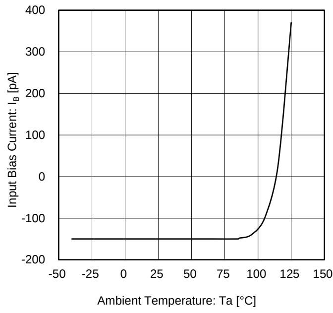
Figure 22. 入力バイアス電流 vs 温度
