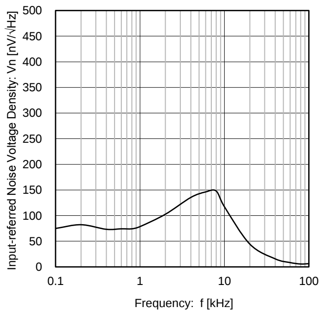
Figure 23. 入力換算雑音電圧密度 vs 周波数 ( V_s = 2.7\text{ V} )
