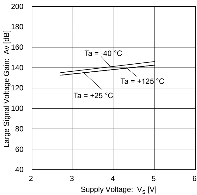
Figure 17. 大振幅電圧利得 vs 電源電圧
