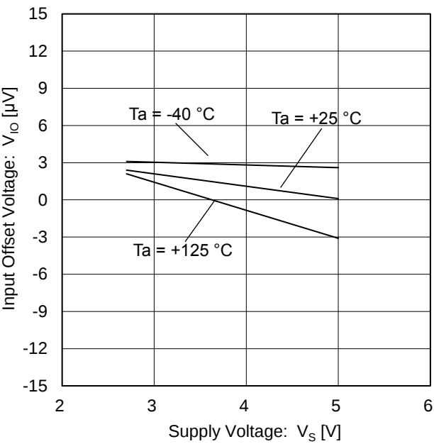
Figure 13. 入力オフセット電圧 vs 電源電圧 ( V_{ICM} = V_{DD} )
