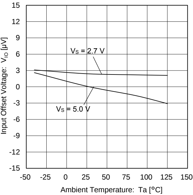
Figure 14. 入力オフセット電圧 vs 温度 ( V_{ICM} = V_{DD} )
