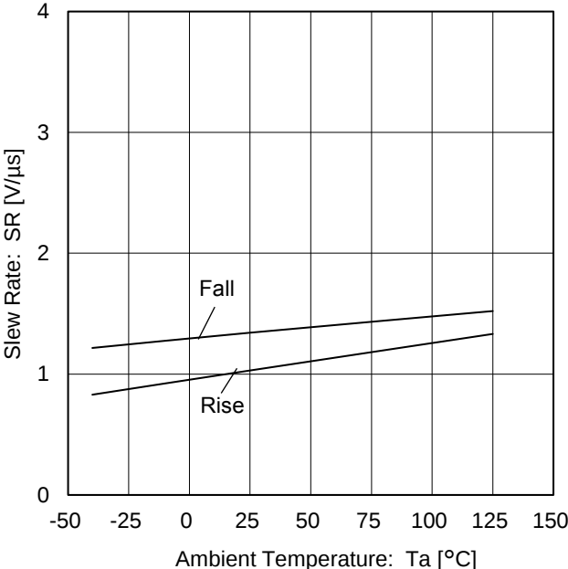
Figure 26. スルーレート vs 温度 ( V_S = 2.7\text{ V} )
