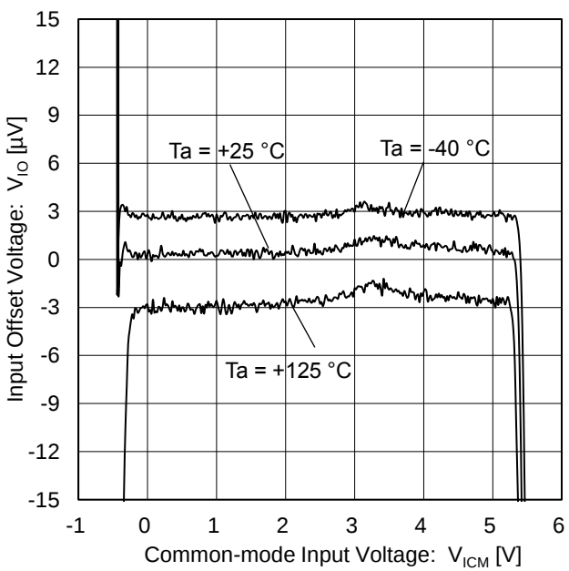
Figure 16. 入力オフセット電圧 vs 同相入力電圧 ( V_S = 5\text{ V} )
