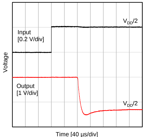
Figure 36. オーバーロードリカバリ ( V_S = 2.7\text{ V} , G = 40\text{ dB} , V_{IN} = (V_{DD}/2 - 0.2\text{ V}) to V_{DD}/2 )
