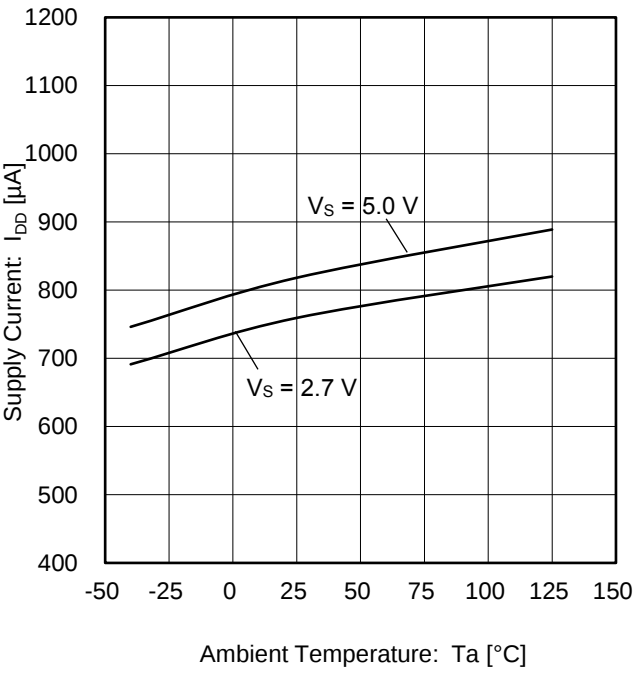
Figure 2. 回路電流 vs 温度
