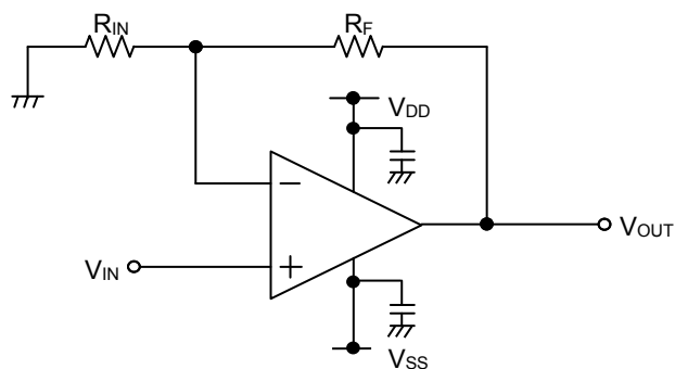
Figure 41. 非反転増幅回路
