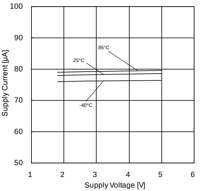
Figure 2. 回路電流－電源電圧特性
