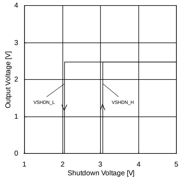
Figure 24. シャットダウン出力電圧 ( V_{DD}=5V , A_v=0dB , V_{IN}=2.5V )
