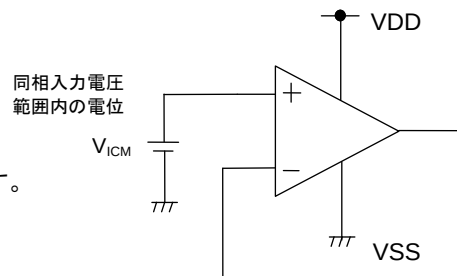
Figure 77. 未使用回路処理例
