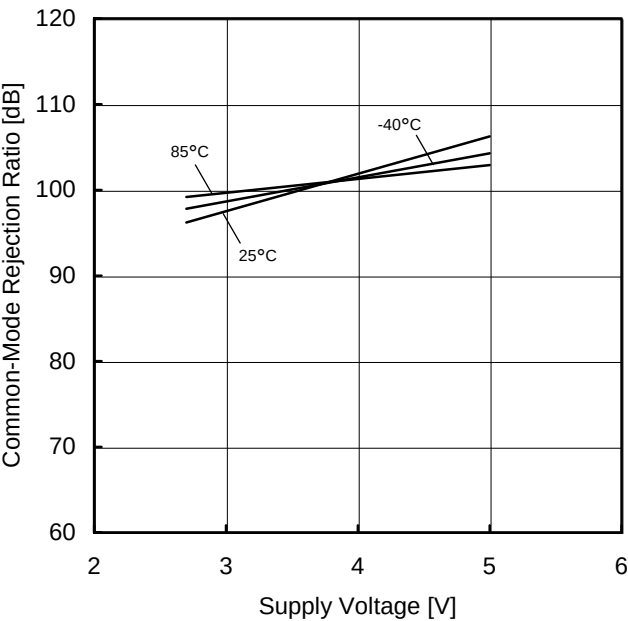
Figure 41. 同相信号除去比—電源電圧特性 (VDD=2.7V)
