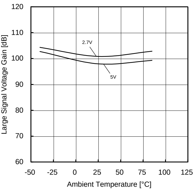
Figure 62. 大振幅電圧利得－温度特性
