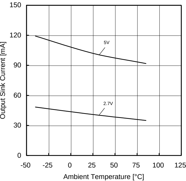
Figure 57. 出力シンク電流－温度特性 (OUT=2.7V)
