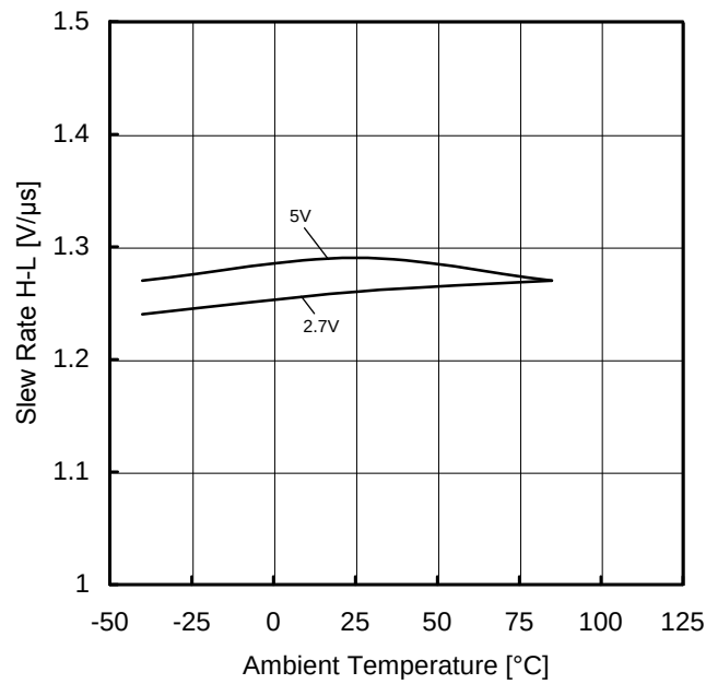
Figure 45. スルーレート(H-L)－温度特性 ( R_L=10k\Omega )
