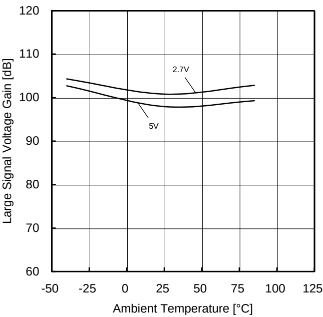
Figure 40. 大振幅電圧利得－温度特性
