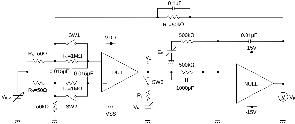
Figure 69. 測定回路(1 回路のみ)
