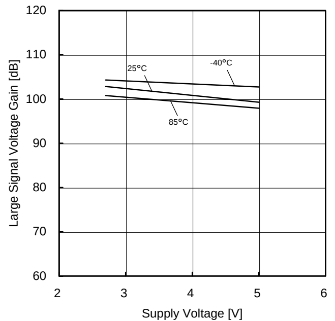
Figure 39. 大振幅電圧利得－電源電圧特性
