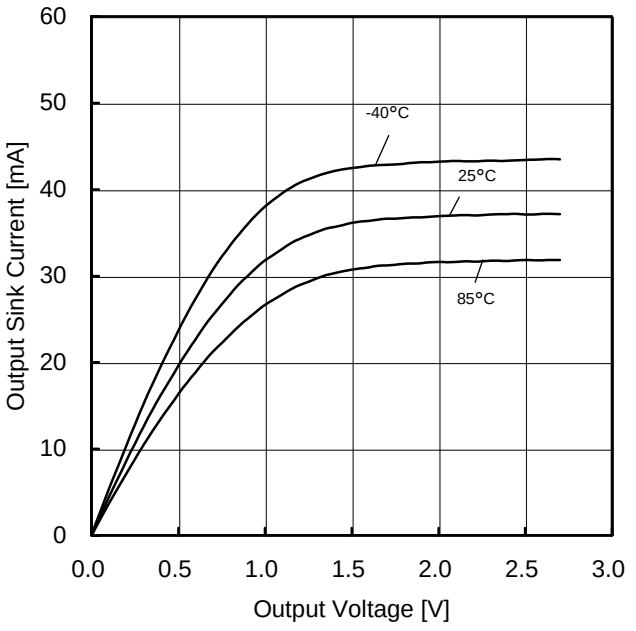
Figure 34. 出力シンク電流－出力電圧特性 (VDD=2.7V)
