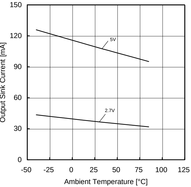
Figure 35. 出力シンク電流－温度特性 (OUT=2.7V)
