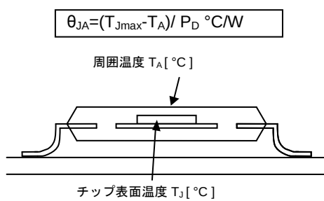
(a) 熱抵抗
