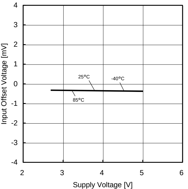
Figure 12. 入力オフセット電圧－電源電圧特性 ( V_{ICM}=VDD/2 , OUT=VDD/2 )
