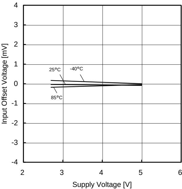
Figure 58. 入力オフセット電圧－電源電圧特性 ( V_{ICM}=VDD/2 , E_K=-VDD/2 )
