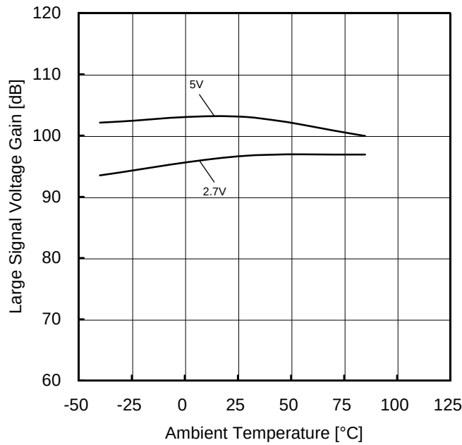
Figure 16. 大振幅電圧利得－温度特性
