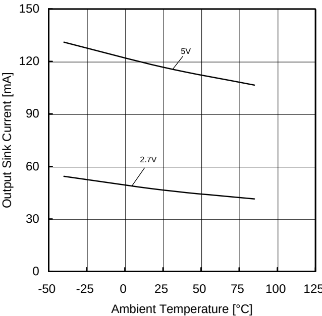
Figure 11. 出力シンク電流－温度特性 (OUT=VDD)
