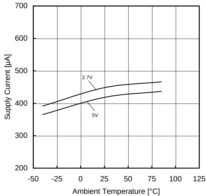
Figure 49. 回路電流－温度特性
