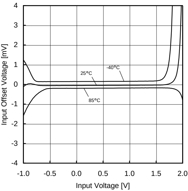
Figure 60. 入力オフセット電圧－入力電圧特性 ( V_{DD}=2.7V , E_K=-V_{DD}/2 )
