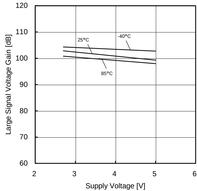
Figure 61. 大振幅電圧利得－電源電圧特性
