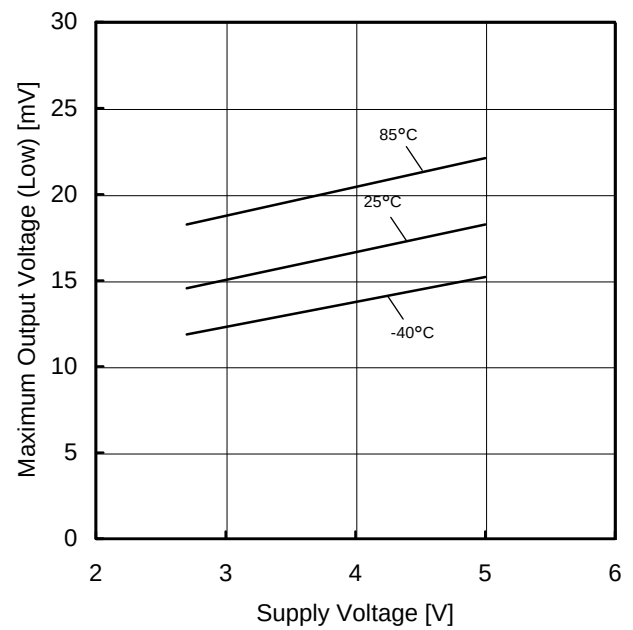
Figure 30. 最大出力電圧(Low)－電源電圧特性 ( R_L=2k\Omega )
