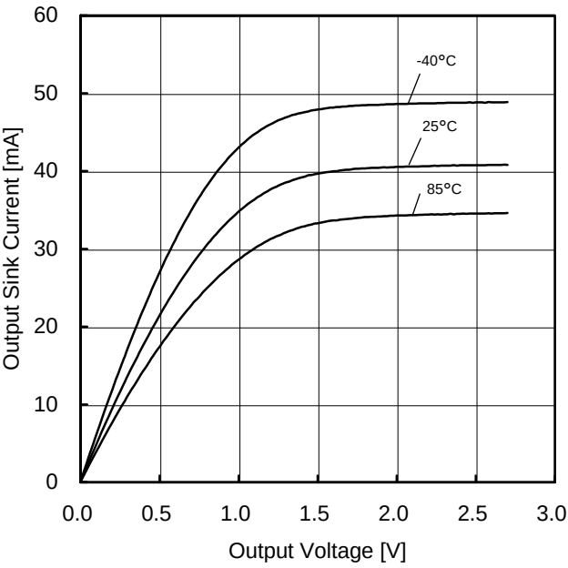
Figure 56. 出力シンク電流－出力電圧特性 (VDD=2.7V)
