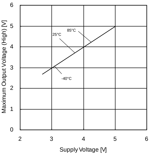
Figure 4. 最大出力電圧(High)－電源電圧特性 (RL=2kΩ)
