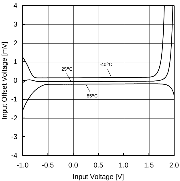
Figure 38. 入力オフセット電圧－入力電圧特性 ( V_{DD}=2.7V , E_K=-V_{DD}/2 )
