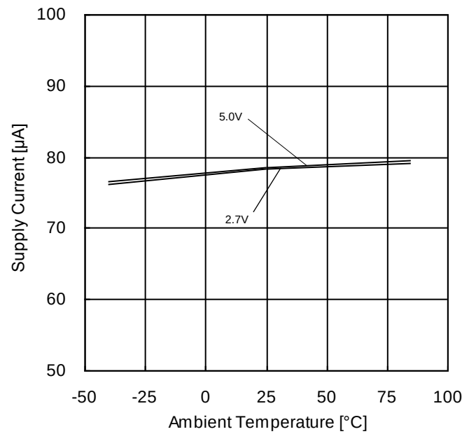
Figure 3. 回路電流－温度特性
