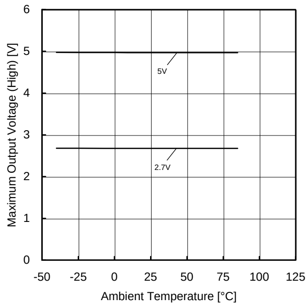
Figure 5. 最大出力電圧(High)－温度特性 ( R_L=2k\Omega )
