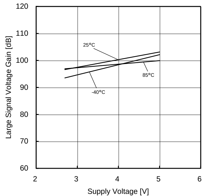
Figure 15. 大振幅電圧利得－電源電圧特性
