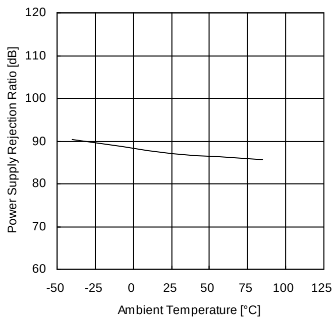
Figure 65. 電源電圧除去比－温度特性 (VDD=2.7V ~ 5.0V)
