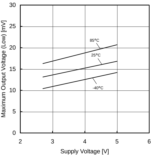
Figure 52. 最大出力電圧(Low)－電源電圧特性 ( R_L=2k\Omega )
