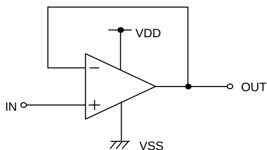
Figure 73. ボルテージフォロワ回路
