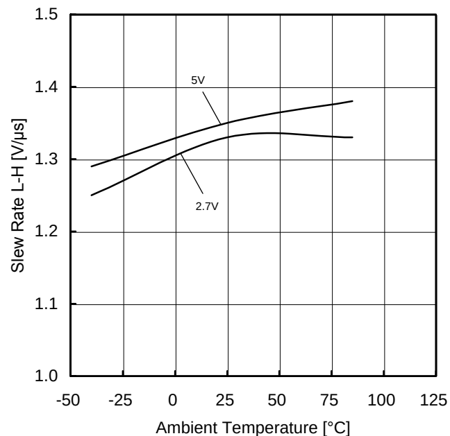
Figure 66. スルーレート(L-H)－温度特性 (RL=10kΩ)
