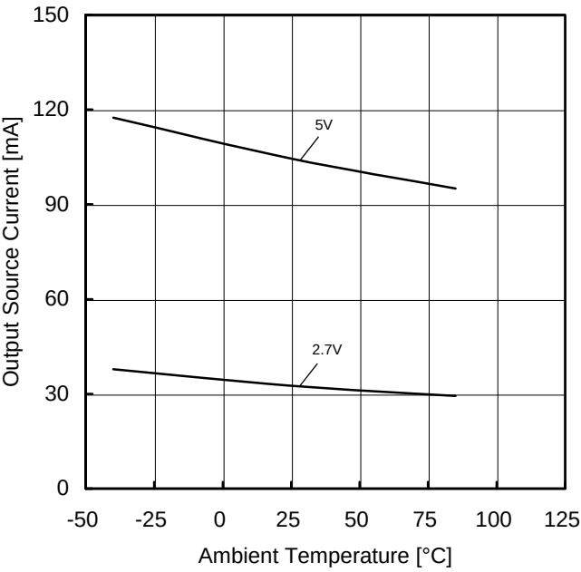
Figure 33. 出力ソース電流－温度特性 (OUT=0V)
