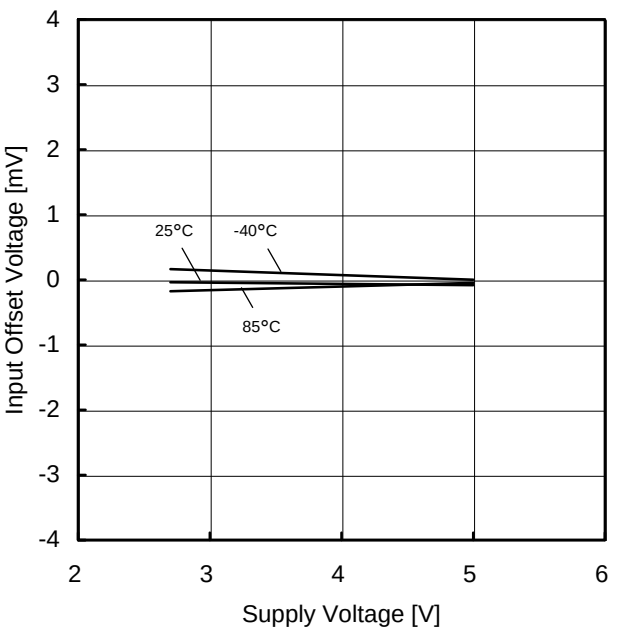
Figure 36. 入力オフセット電圧－電源電圧特性 (V ICM =VDD/2, OUT=VDD/2)
