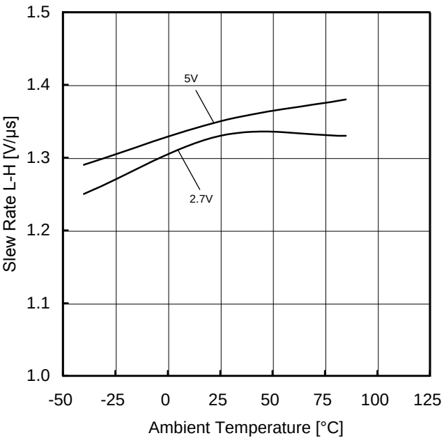
Figure 44. スルーレート(L-H)—温度特性 (RL=10kΩ)
