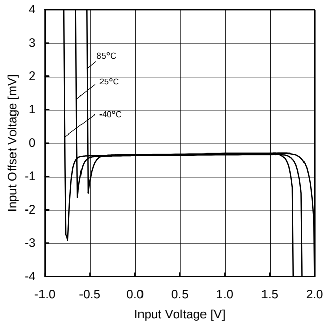
Figure 14. 入力オフセット電圧－入力電圧特性 ( V_{DD}=2.7V , E_K=-V_{DD}/2 )
