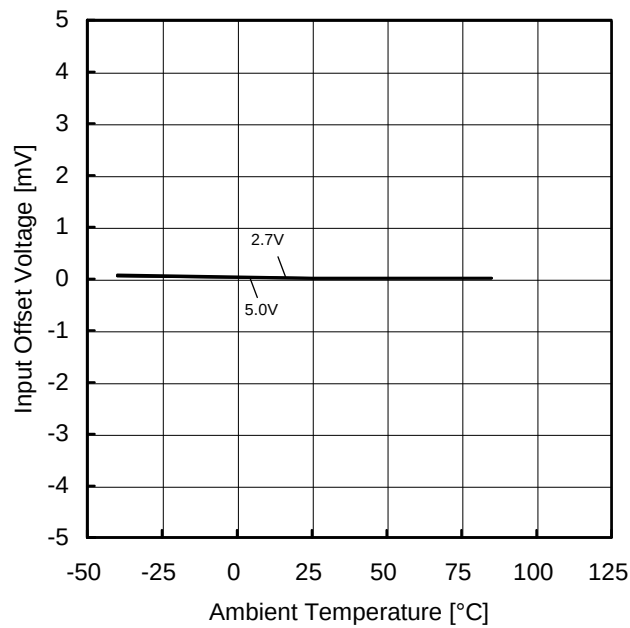
Figure 37. 入力オフセット電圧－温度特性 ( V_{ICM}=V_{DD}/2 , E_K=-V_{DD}/2 )
