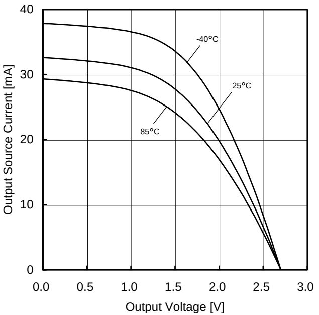
Figure 54. 出力ソース電流－出力電圧特性 ( V_{DD}=2.7V )
