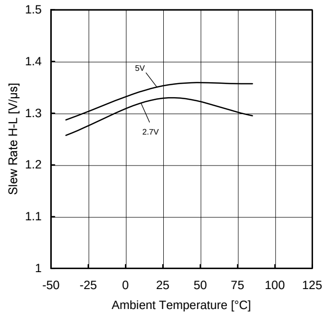
Figure 21. スルーレート(H-L)－温度特性 ( R_L=10k\Omega )
