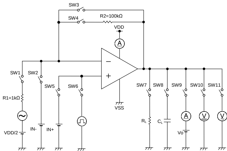
Figure 70. 測定回路 2 (1 回路のみ)
