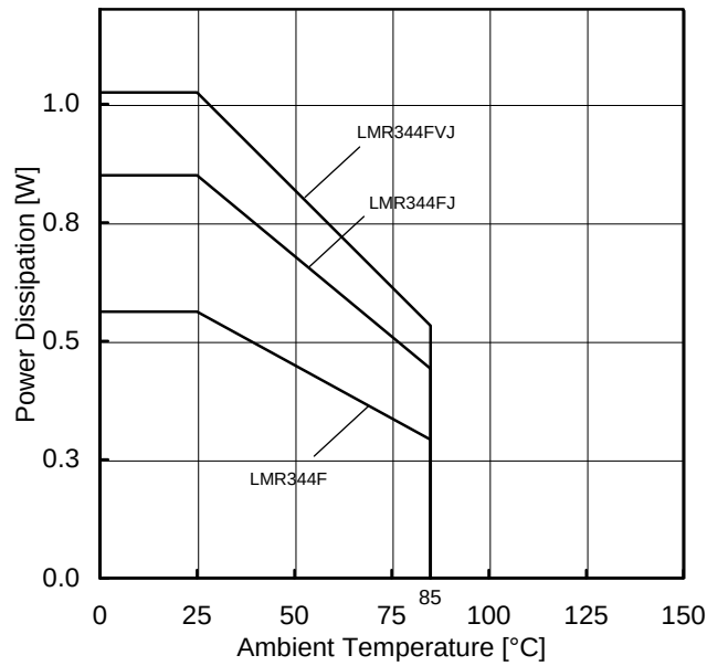
Figure 47. ディレーティングカーブ
