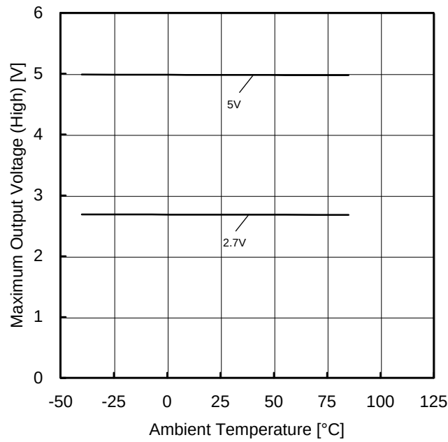
Figure 51. 最大出力電圧(High)－温度特性 ( R_L=2k\Omega )
