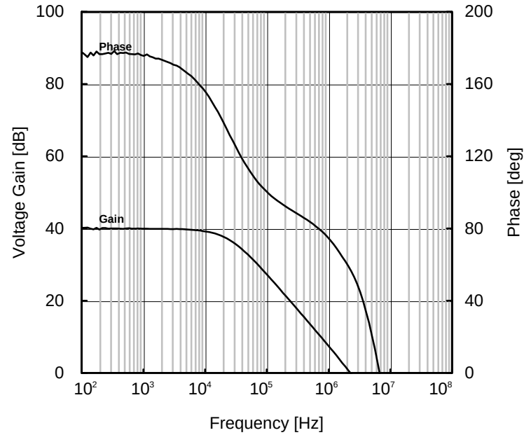
Figure 22. 電圧利得・位相－周波数特性 ( C=20pF )
