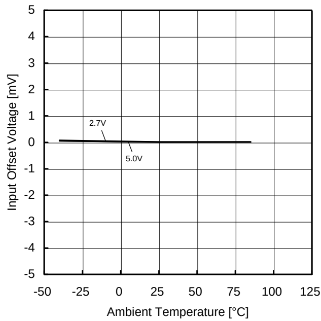
Figure 59. 入力オフセット電圧－温度特性 ( V_{ICM}=V_{DD}/2 , E_K=-V_{DD}/2 )
