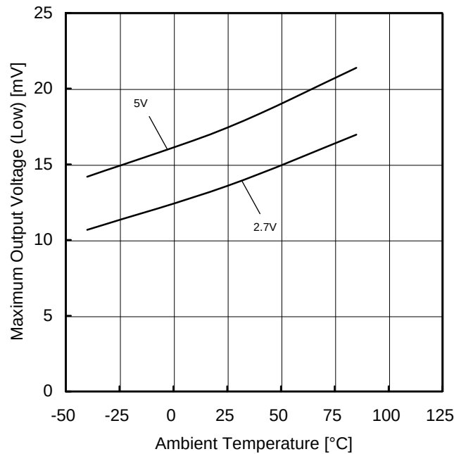
Figure 53. 最大出力電圧(Low)－温度特性 ( R_L=2k\Omega )
