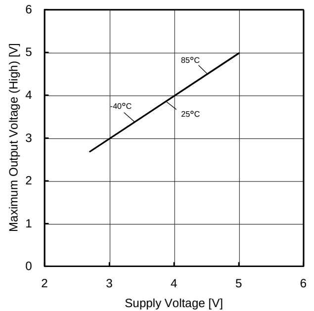
Figure 28. 最大出力電圧(High)－電源電圧特性 ( R_L=2k\Omega )
