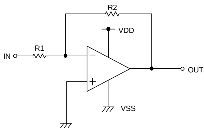
Figure 74. 反転増幅回路
