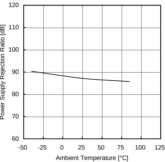
Figure 43. 電源電圧除去比—温度特性 (VDD=2.7V ~ 5.0V)
