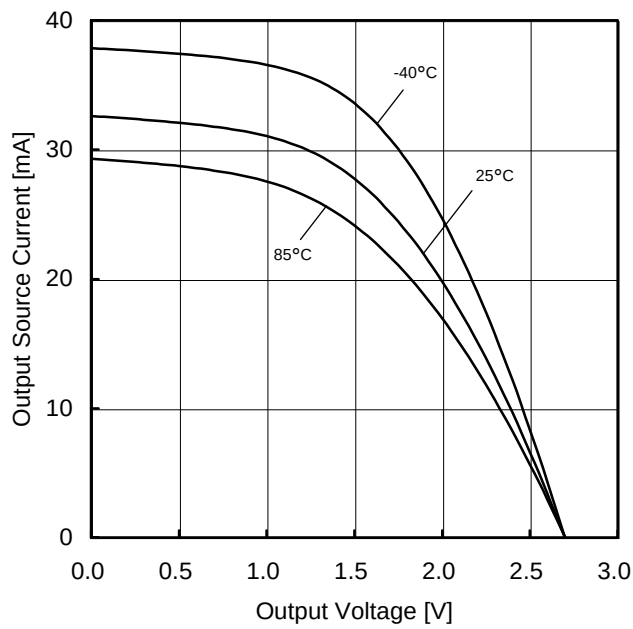
Figure 32. 出力ソース電流－出力電圧特性 ( V_{DD}=2.7V )
