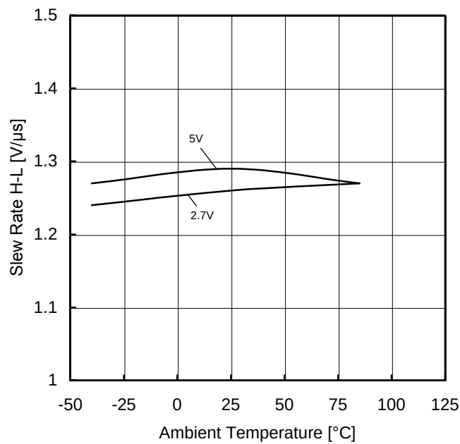
Figure 67. スルーレート(H-L)－温度特性 ( R_L=10k\Omega )
