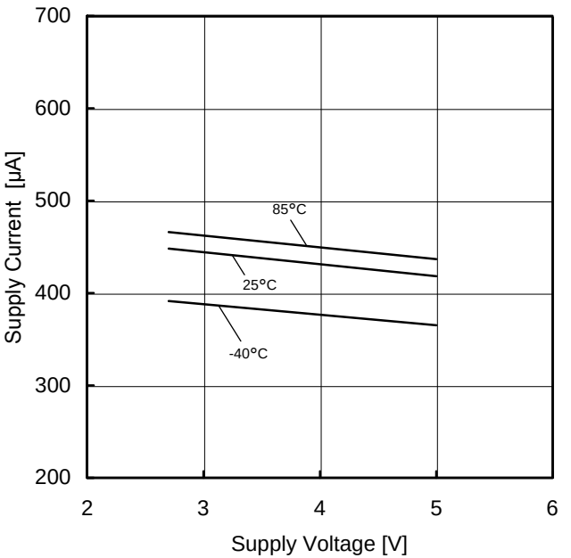
Figure 48. 回路電流－電源電圧特性
