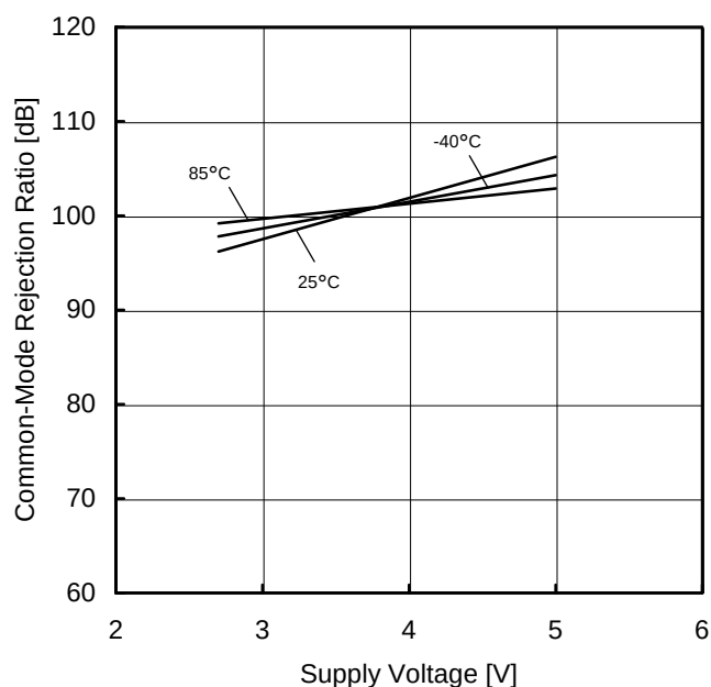
Figure 63. 同相信号除去比－電源電圧特性 (VDD=2.7V)
