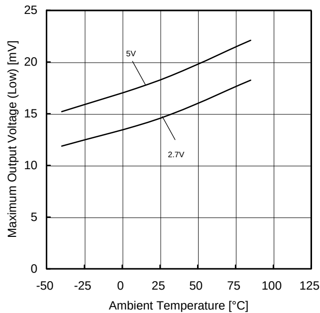
Figure 31. 最大出力電圧(Low)－温度特性 ( R_L=2k\Omega )
