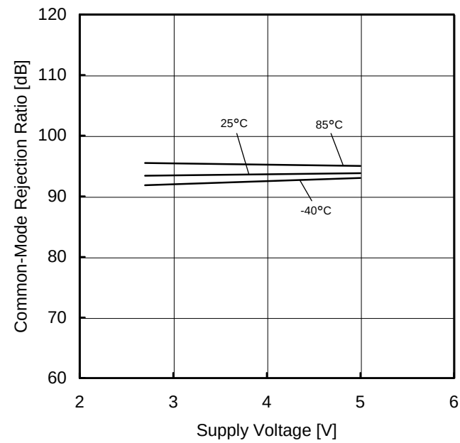
Figure 17. 同相信号除去比－電源電圧特性 (VDD=2.7V)
