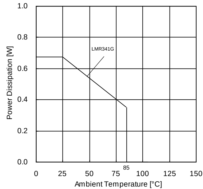
Figure 1. ディレーティングカーブ
