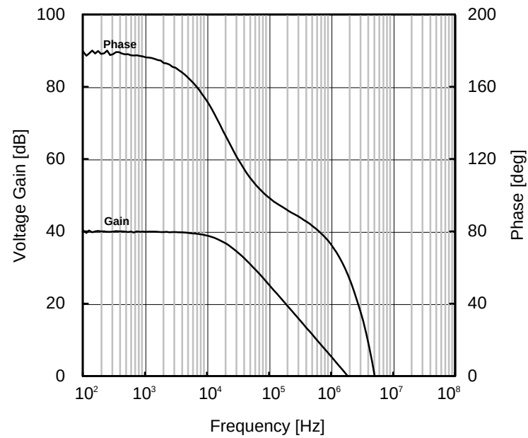
Figure 46. 電圧利得・位相－周波数特性 ( C=20pF )
