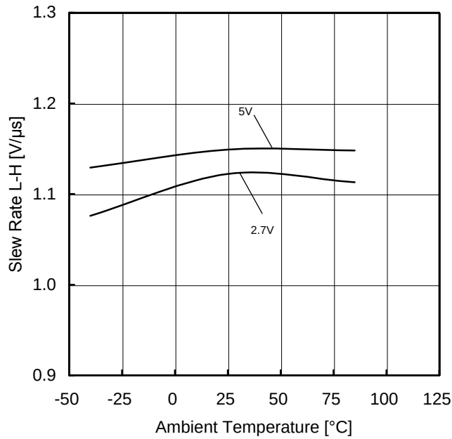
Figure 20. スルーレート(L-H)－温度特性 (RL=10kΩ)
