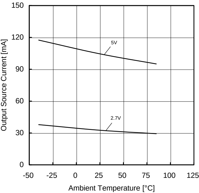
Figure 55. 出力ソース電流－温度特性 (OUT=0V)
