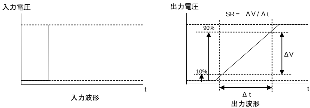
Figure 71. スルーレート測定時 入出力波形
