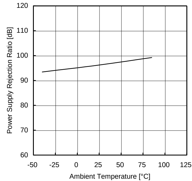
Figure 19. 電源電圧除去比－温度特性 (VDD=2.7V ~ 5.0V)
