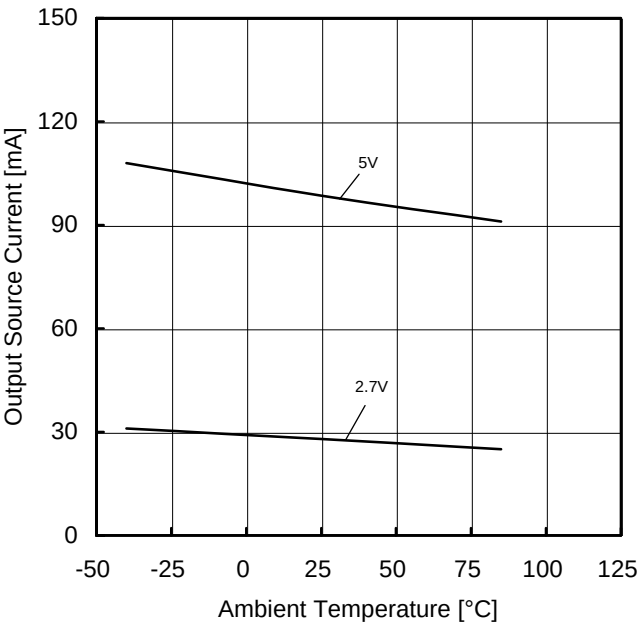
Figure 9. 出力ソース電流－温度特性 (OUT=0V)
