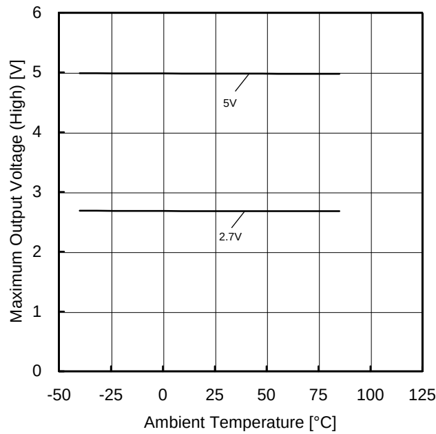
Figure 29. 最大出力電圧(High)－温度特性 ( R_L=2k\Omega )
