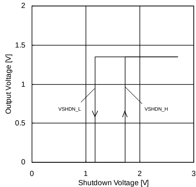
Figure 23. シャットダウン出力電圧 ( V_{DD}=2.7V , A_v=0dB , V_{IN}=1.35V )
