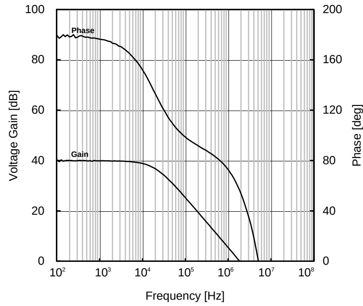
Figure 68. 電圧利得・位相－周波数特性 ( C=20pF )
