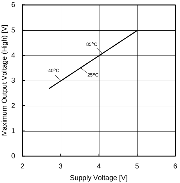
Figure 50. 最大出力電圧(High)－電源電圧特性 ( R_L=2k\Omega )
