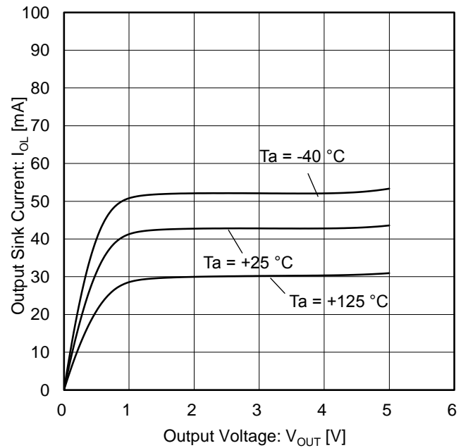
Figure 8. 出力シンク電流 vs 出力電圧 ( V_S = 5.0\text{ V} )
