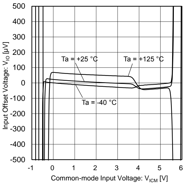
Figure 11. 入力オフセット電圧 vs 同相入力電圧 ( V_s = 5.0\text{ V} )
