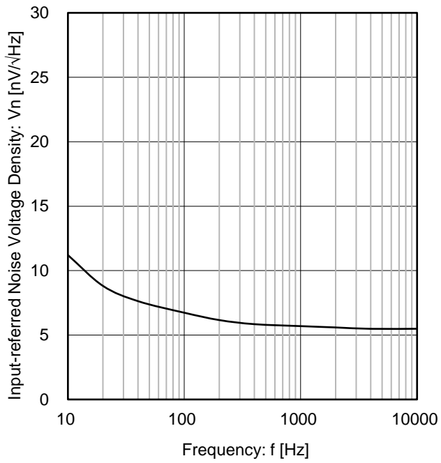
Figure 21. 入力換算雑音電圧密度 vs 周波数 ( V_s = 5.0 \text{ V} )
