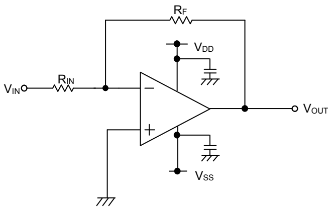
Figure 23. 反転増幅回路
