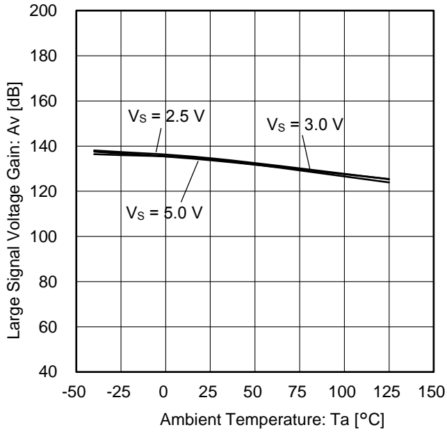
Figure 13. 大振幅電圧利得 vs 温度 ( R_L = 10 k \Omega )
