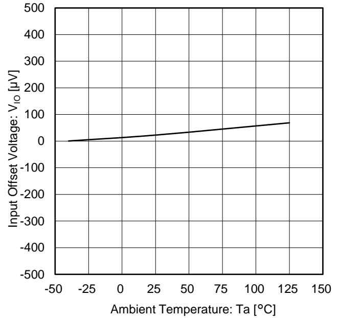
Figure 10. 入力オフセット電圧 vs 温度 ( V_s = 5.0\text{ V} )
