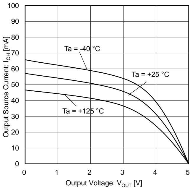
Figure 7. 出力ソース電流 vs 出力電圧 ( V_S = 5.0\text{ V} )
