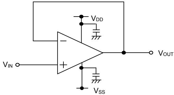
Figure 22. ボルテージフォロフ回路
