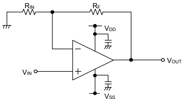
Figure 24. 非反転増幅回路
