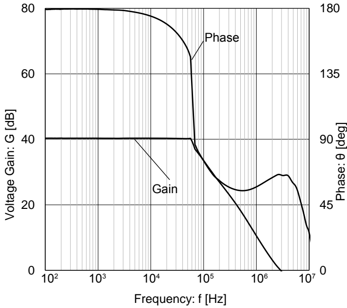
Figure 17. 電圧利得・位相 vs 周波数 ( V_S = 5.0\text{ V} )
