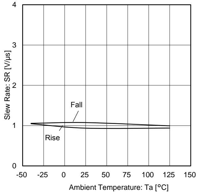
Figure 20. スルーレート vs 温度 ( V_S = 5.0\text{ V} )
