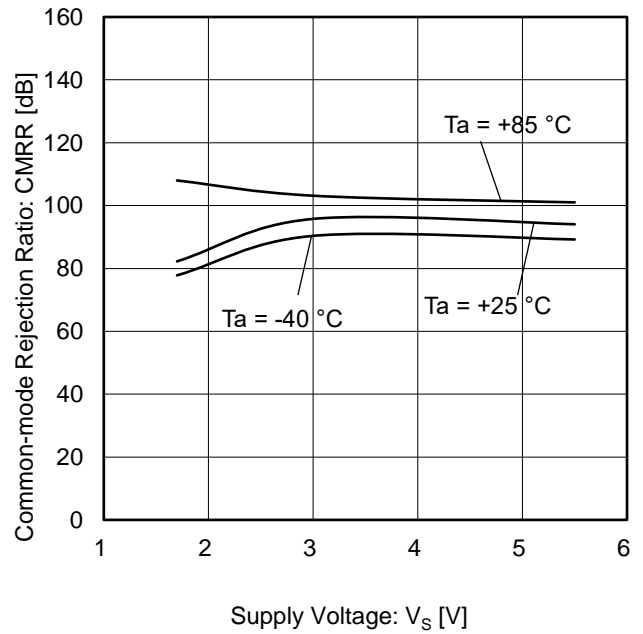
Figure 16. 同相信号除去比 vs 電源電圧
