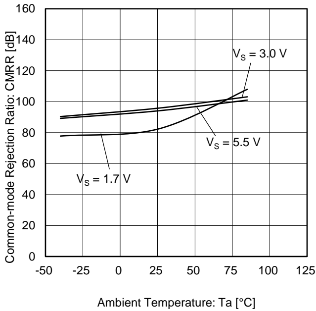
Figure 17. 同相信号除去比 vs 温度
