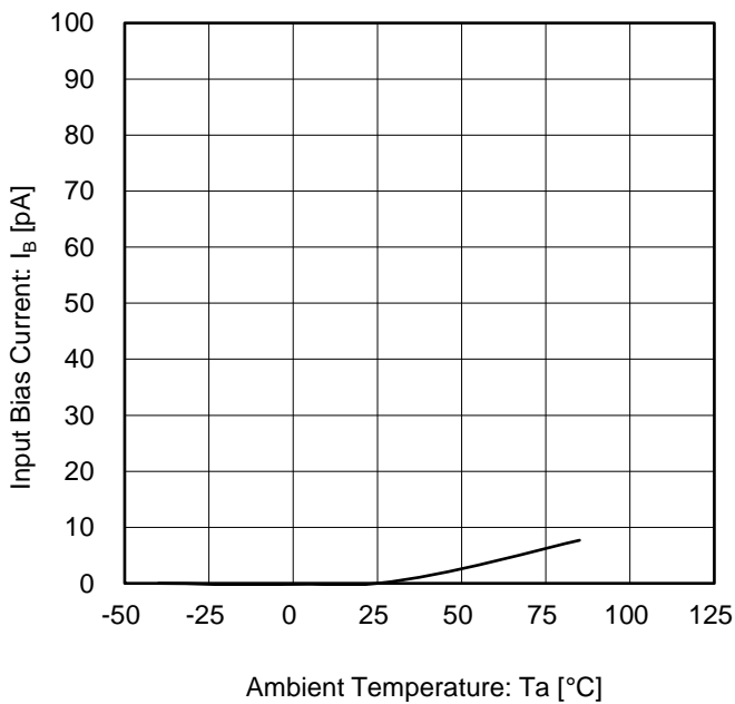
Figure 19. 入力バイアス電流 vs 温度
