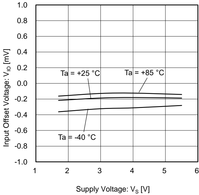
Figure 9. 入力オフセット電圧 vs 電源電圧 ( V_{ICM} = 0\text{ V} )
