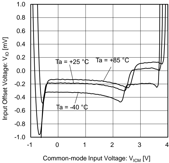
Figure 13. 入力オフセット電圧 vs 同相入力電圧 ( V_S = 3\text{ V} )
