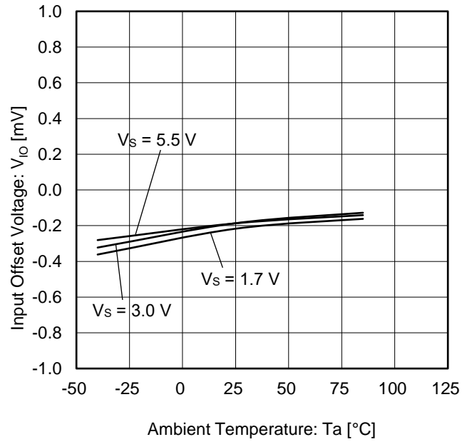
Figure 10. 入力オフセット電圧 vs 温度 ( V_{ICM} = 0\text{ V} )
