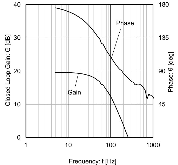
Figure 24. クローズドループゲイン・位相 vs 周波数 ( V_S = 3\text{ V} )
