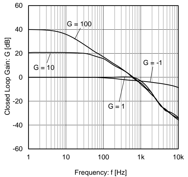
Figure 26. クローズドループゲイン vs 周波数 ( V_S = 3\text{ V} )
