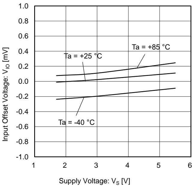
Figure 11. 入力オフセット電圧 vs 電源電圧 ( V_{ICM} = V_{DD} )
