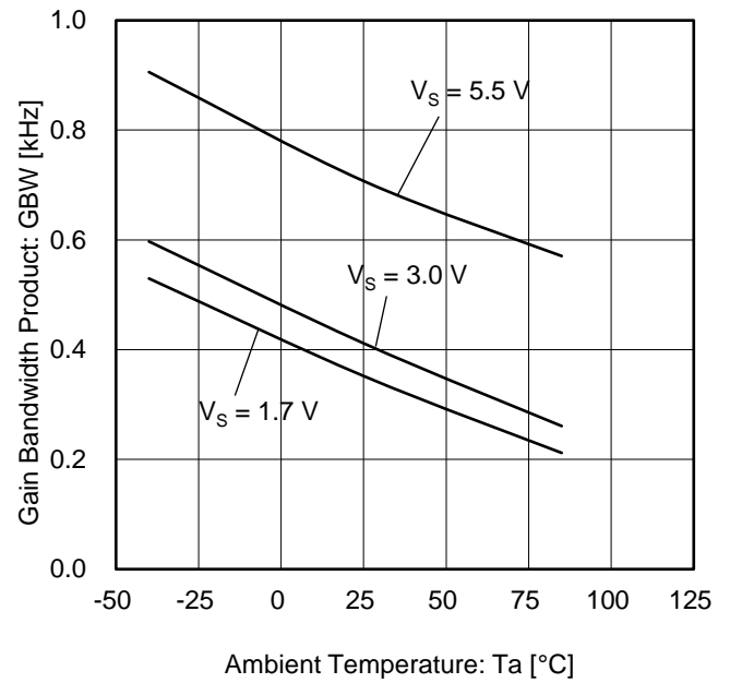
Figure 22. 利得帯域幅積 vs 温度
