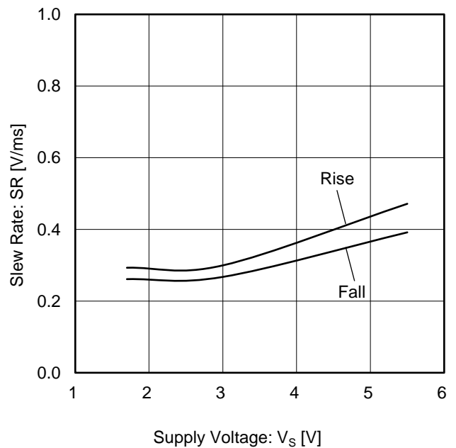
Figure 20. スルーレート vs 電源電圧
