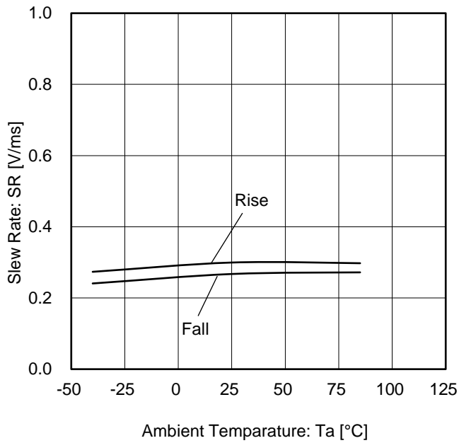
Figure 21. スルーレート vs 温度 ( V_S = 3\text{ V} )
