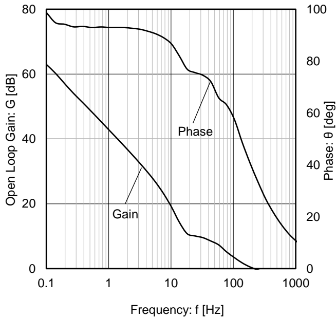
Figure 25. オープンループゲイン・位相 vs 周波数 ( V_S = 3\text{ V} )
