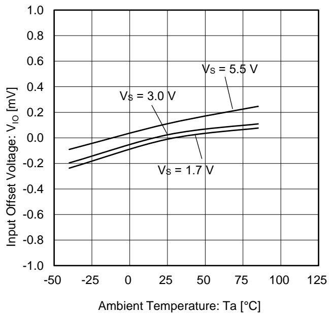
Figure 12. 入力オフセット電圧 vs 温度 ( V_{ICM} = V_{DD} )
