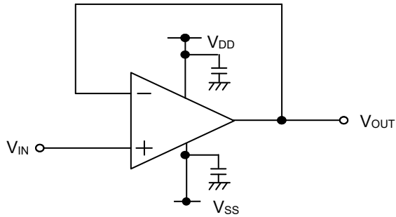
Figure 28. ボルテージフォロフ回路
