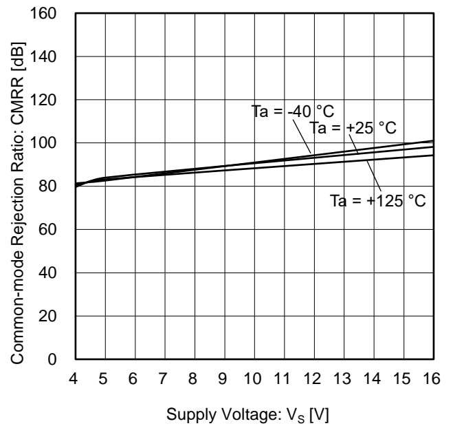
Figure 14. 同相信号除去比 vs 電源電圧
