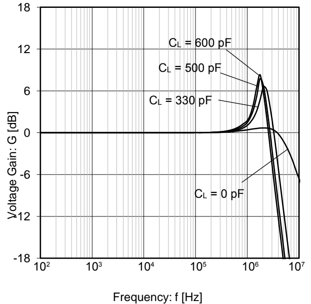
Figure 24. 電圧利得 vs 周波数 ( V_S = 5\text{ V} , G = 0\text{ dB} , V_{IN} = 180\text{ mV}_{P-P} )
