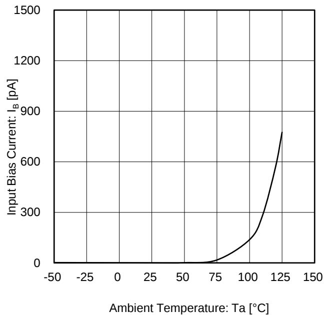
Figure 17. 入力バイアス電流 vs 温度 ( V_S = 5\text{ V} )
