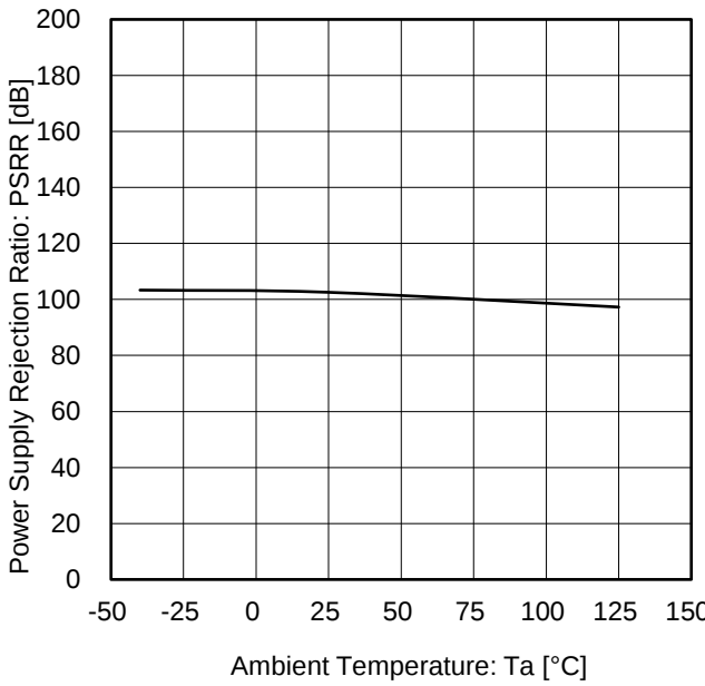
Figure 16. 電源電圧除去比 vs 温度
