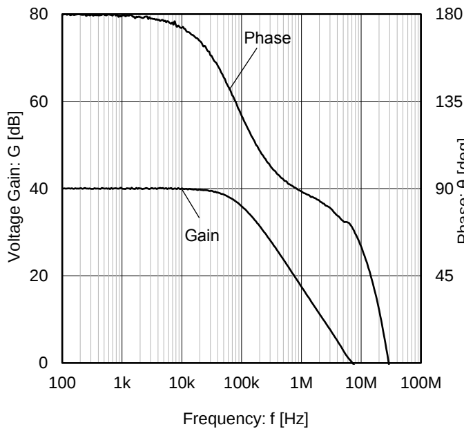
Figure 23. 電圧利得・位相 vs 周波数 ( V_S = 5\text{ V} )
