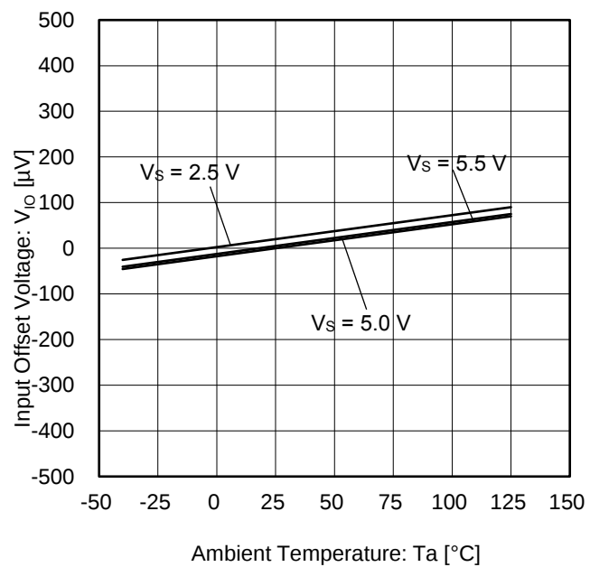
Figure 10. 入力オフセット電圧 vs 温度
