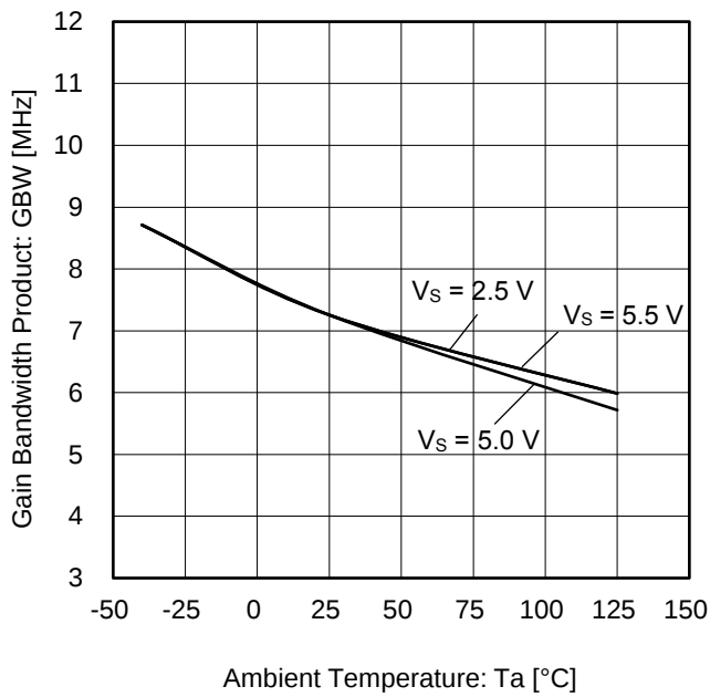
Figure 21. 利得帯域幅積 vs 温度
