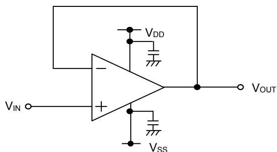
Figure 25. ボルテージフォロフ回路
