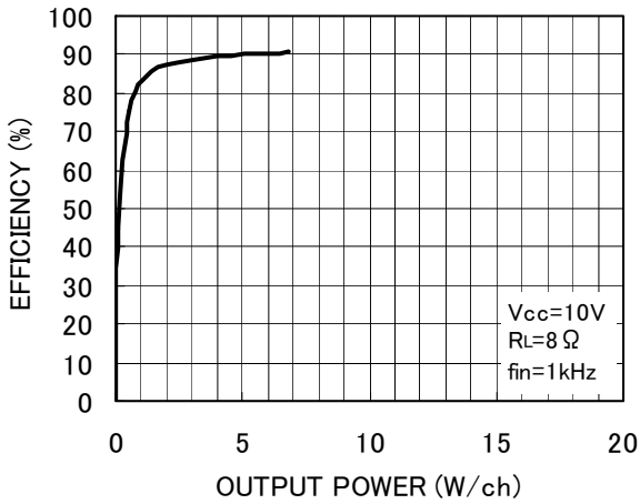
Fig.7 効率 - 出力電力
