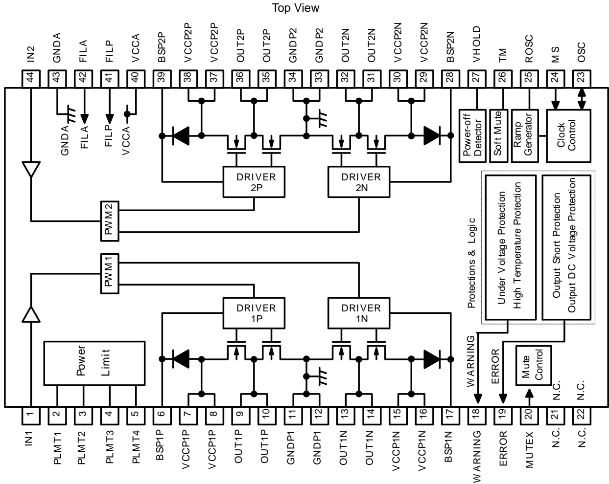
Fig.28 端子配置図
