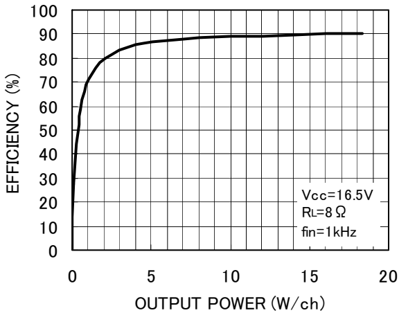
Fig.9 効率 - 出力電力
