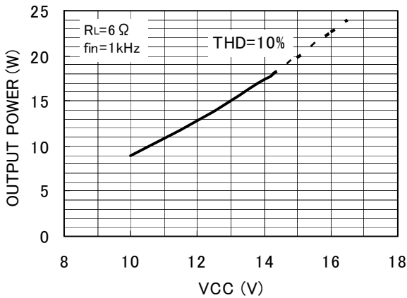
Fig.18 出力電力 - 電源電圧
