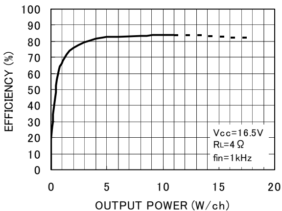
Fig.26 効率 - 出力電力
