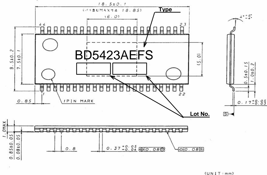
Fig.29 HTSSOP-A44 パッケージ 外形寸法図・標印図
