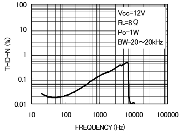
Fig.2 THD+N - 周波数
