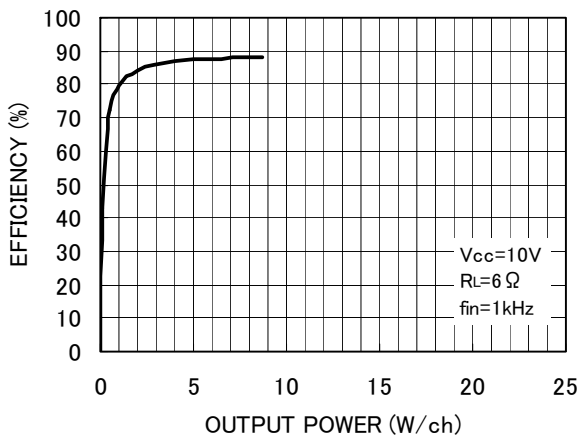
Fig.19 効率 - 出力電力
