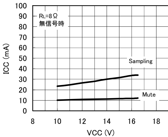
Fig.11 消費電流 - 電源電圧
