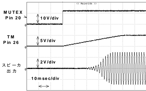
Fig.13 ソフトミュート解除時の波形
