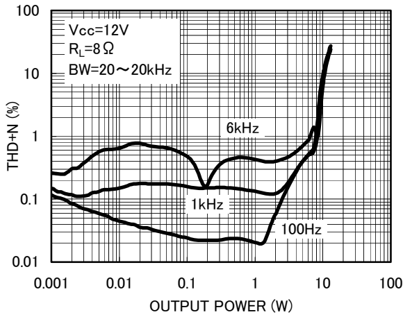
Fig.1 THD+N - 出力電力
