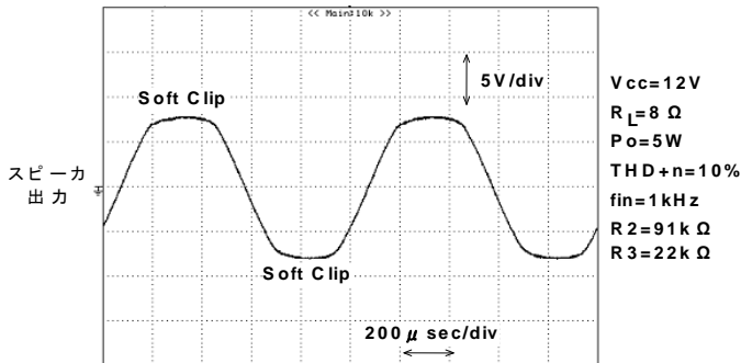
Fig.17 出力電力制限時の波形 (P o =5W)
