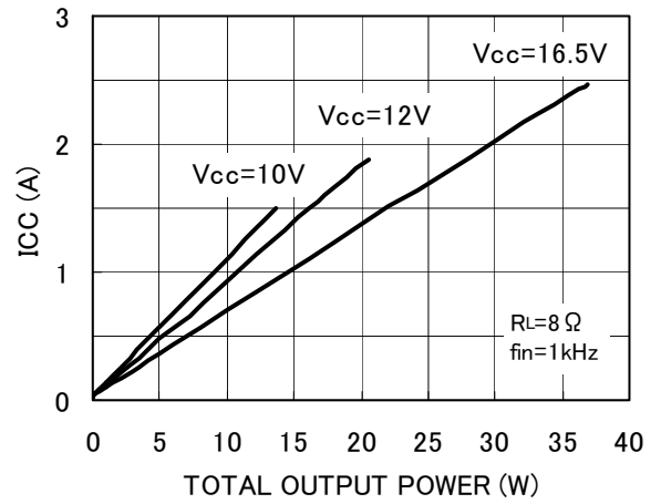
Fig.10 消費電流 - 出力電力
