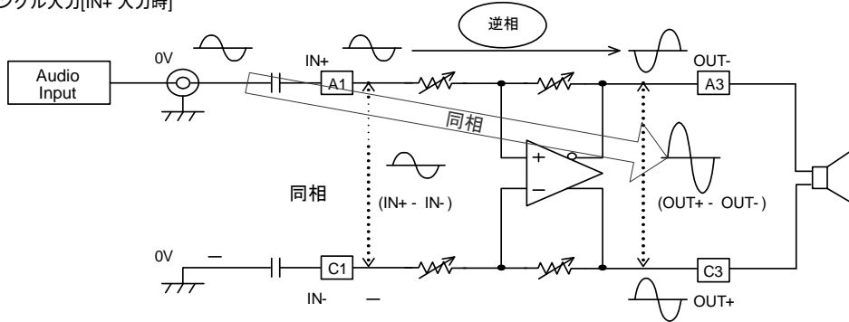
2) シングル入力[IN+ 入力時]
