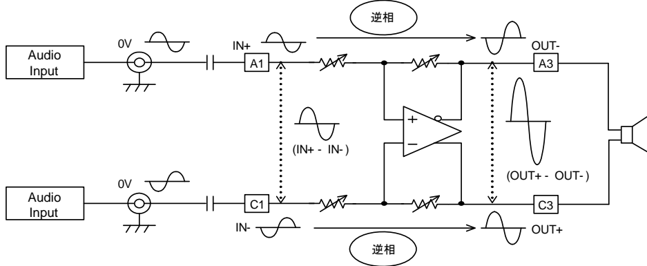
1) 差動入力
