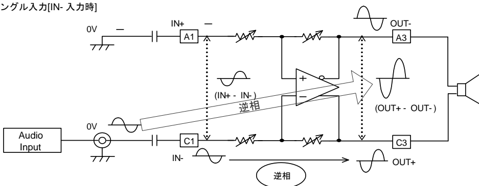
3) シングル入力[IN- 入力時]
