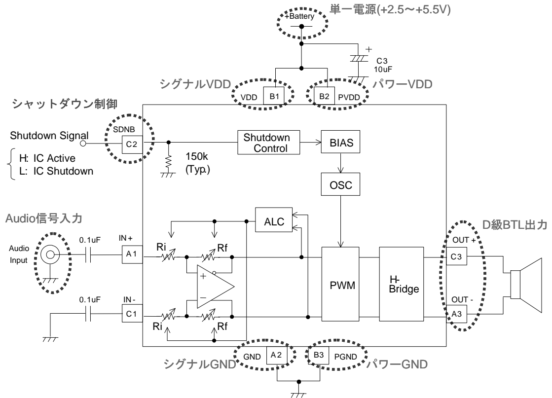
Fig3. シングルエンド入力(IN+入力時)
