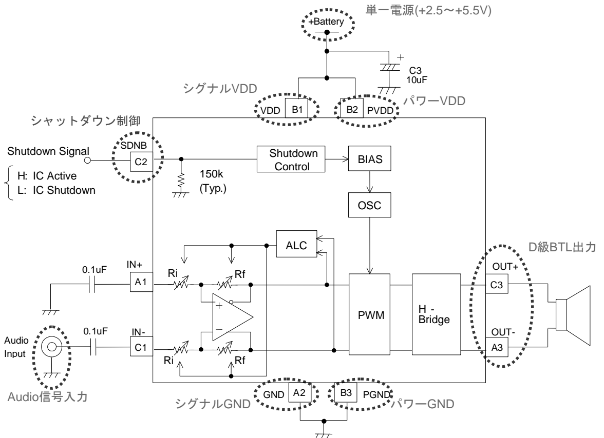
Fig4. シングルエンド入力(IN-入力時)
