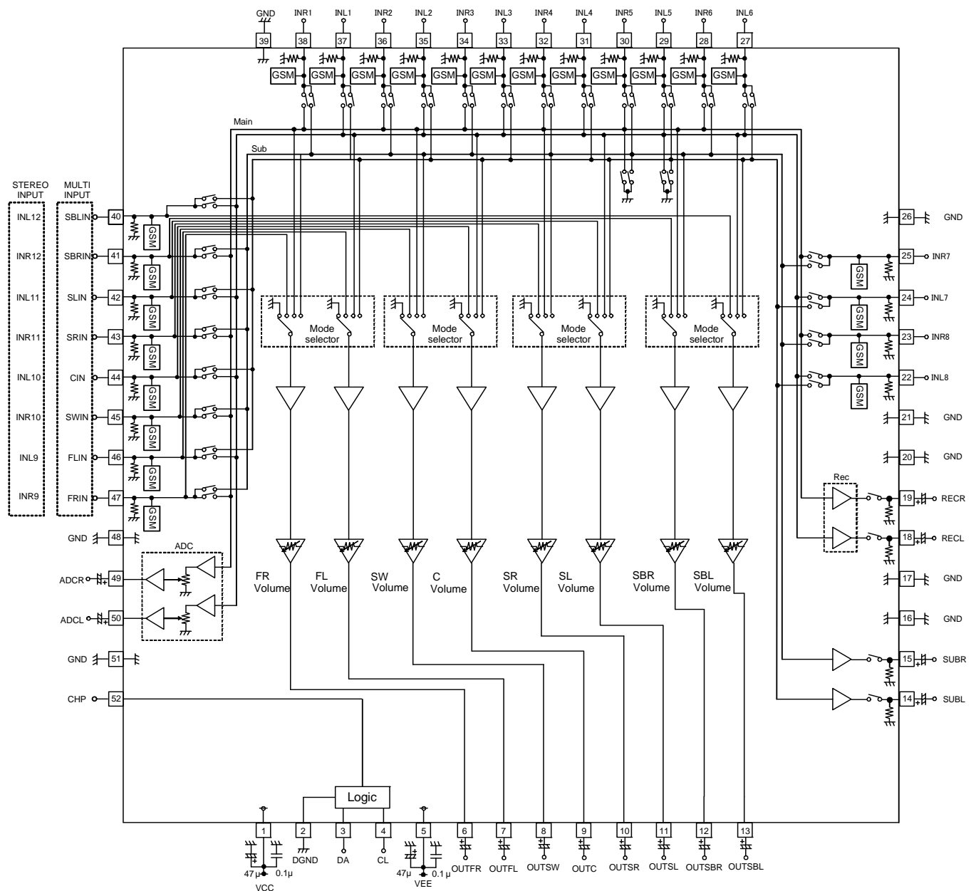
Figure 13. 応用回路例
