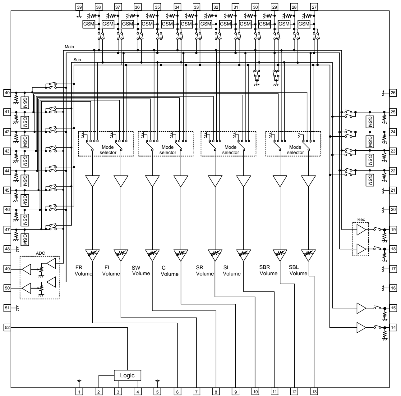
Figure 3. ブロック図
