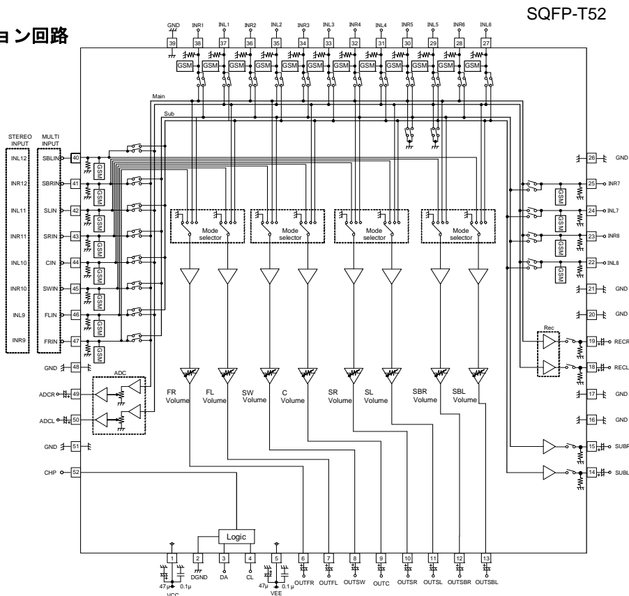
Figure 1. 応用回路例
