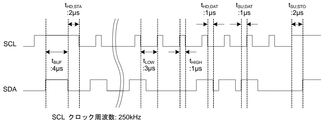
Figure 17. I 2 C データ送信におけるコマンドタイミング例
