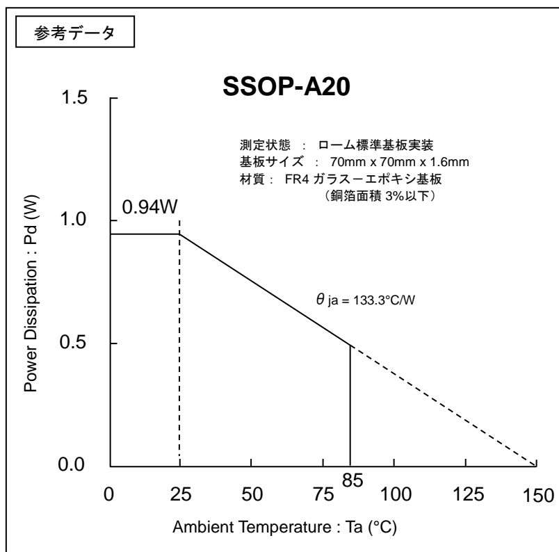
Figure 18. 熱軽減率曲線
