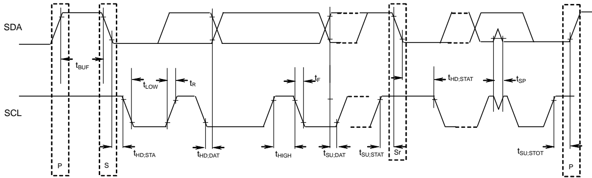
Figure 13. I 2 C バス上のタイミング定義
