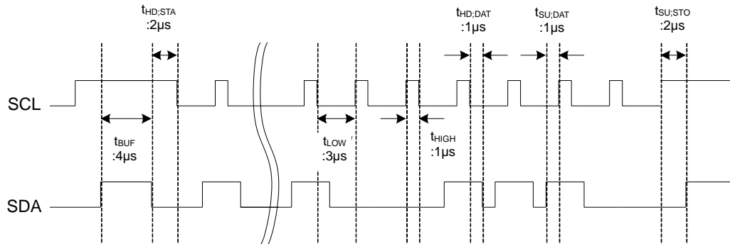
Figure 14. I 2 C データ送信におけるコマンドタイミング例
