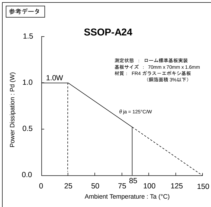
Figure 19. 熱軽減率曲線
