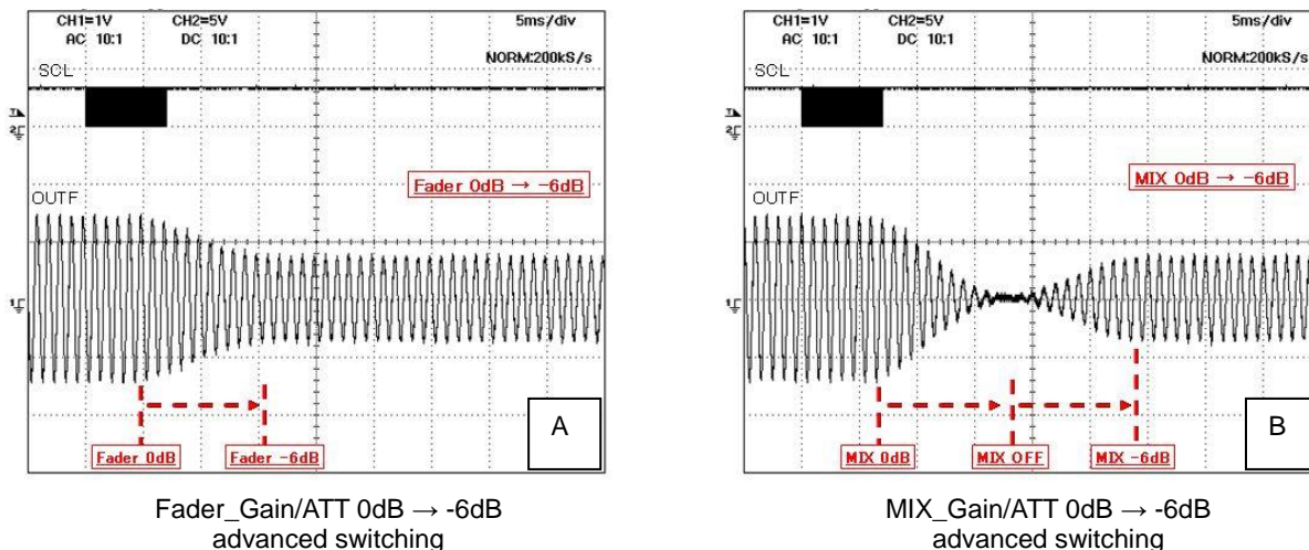
Figure 27. MIX のアドバンススイッチ動作
