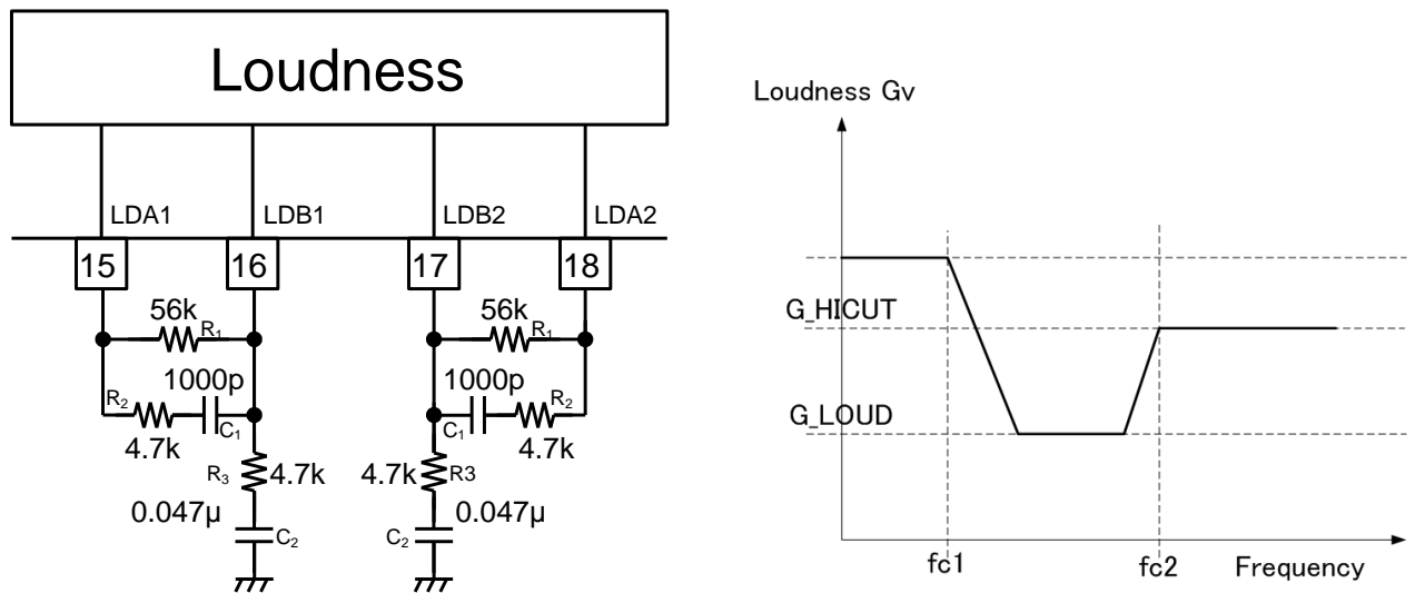
Figure 28. ラウドネス回路の外付け定数設定方法
