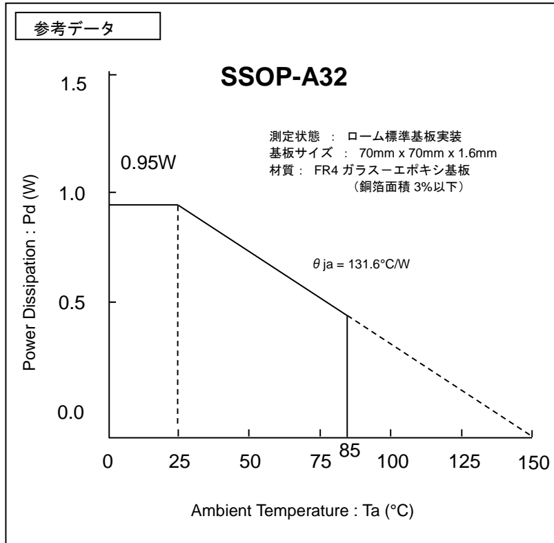
Figure 24. 熱軽減率曲線
