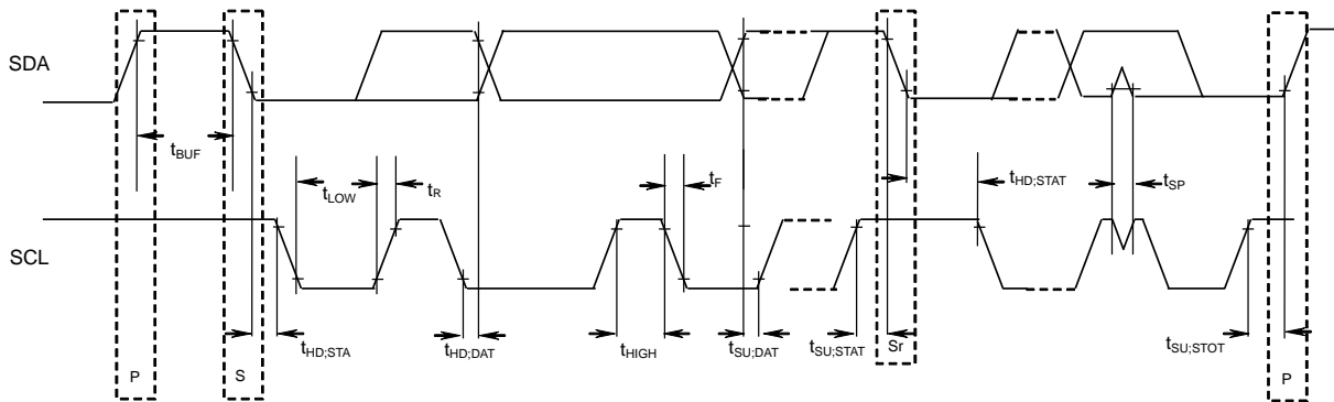
Figure 22. I 2 C バス上のタイミング定義
