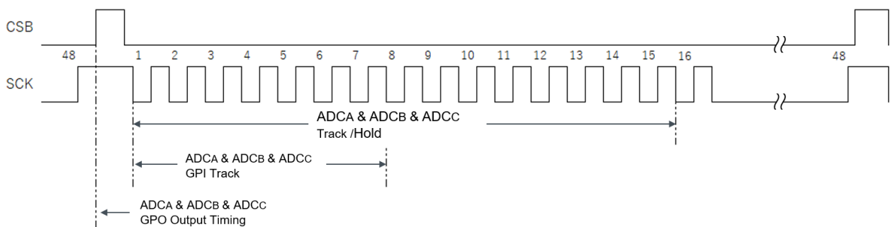
Figure 33. 3 個デイジーチェーン接続時 AGIO 端子更新タイミング
