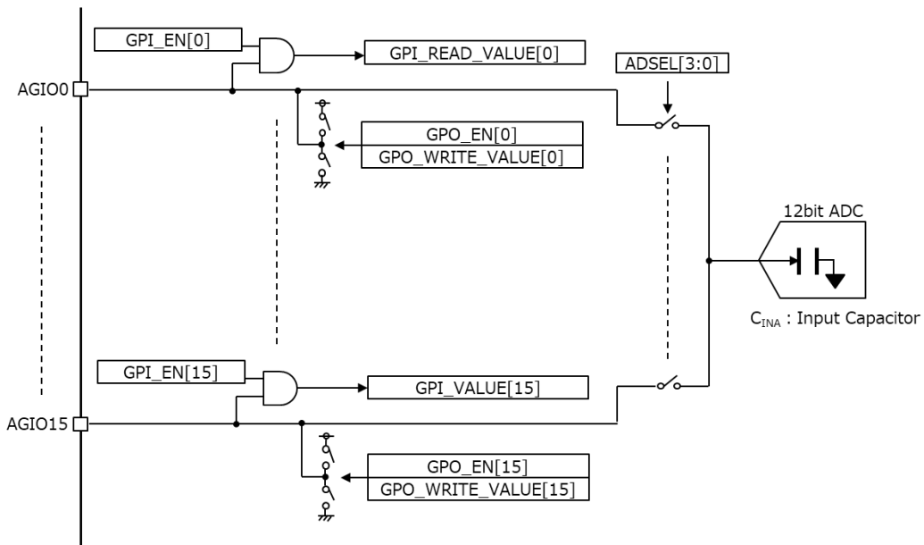
Figure 24. AGIO 端子接続図
