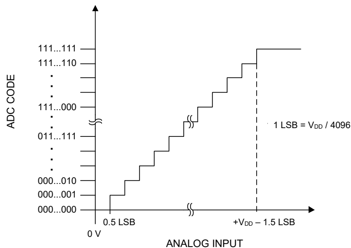
Figure 23. 理想変換特性
