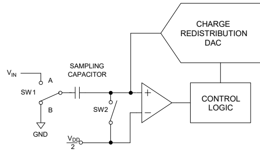
Figure 22. ホールドモード
