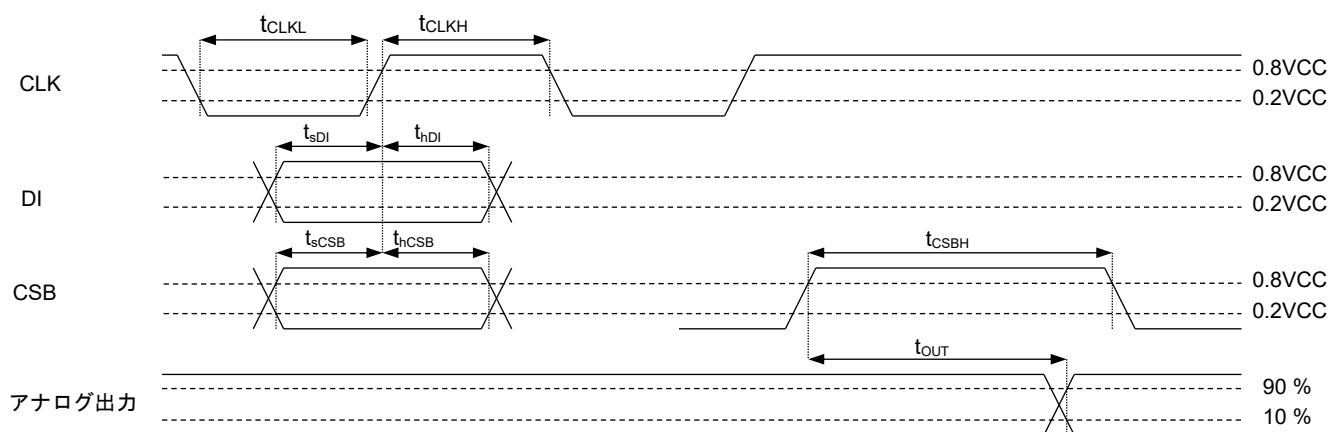
Figure 1. 3線シリアルバスとアナログ出力タイミングチャート
