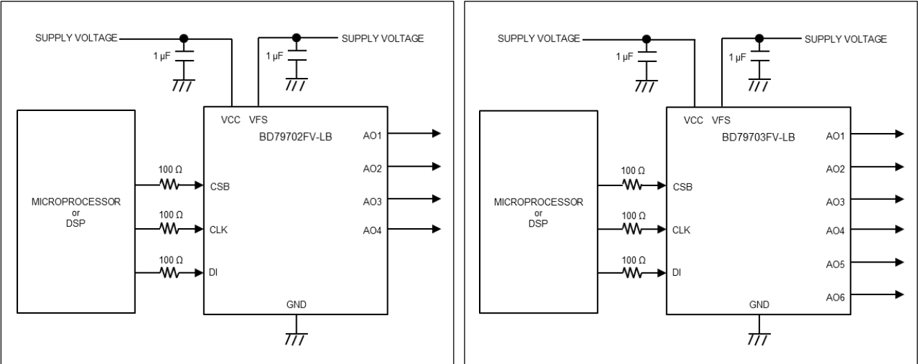
Figure 23. 応用回路図
