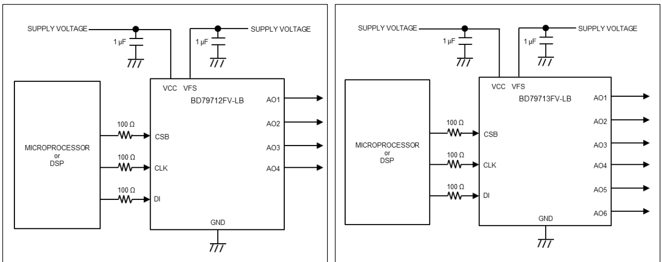
Figure 24. 応用回路図
