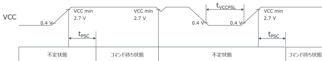
Figure 22. 電源投入時タイミングチャート
