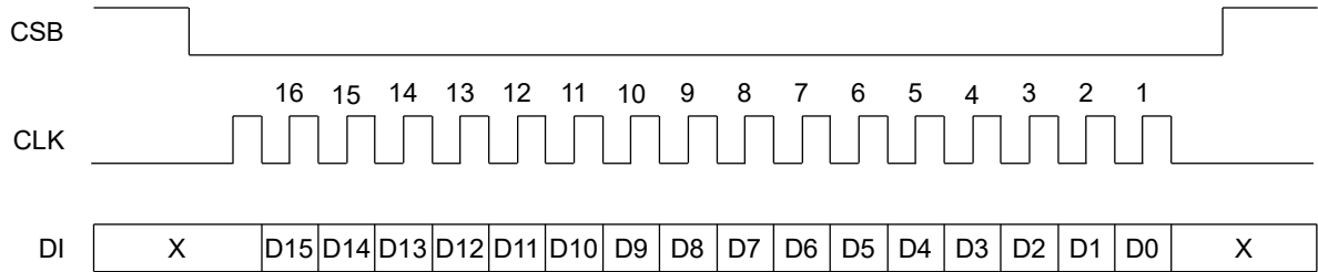
Figure 23. 通信フォーマット
