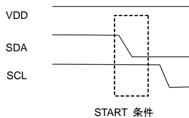
Figure 23. START 条件タイミング
