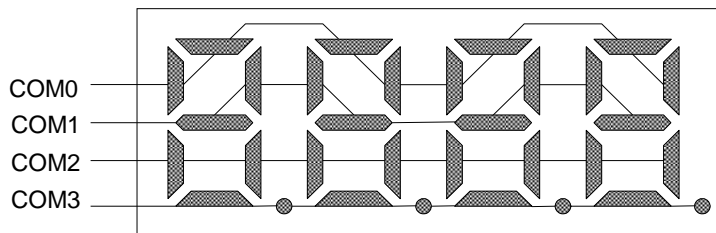
Figure 18. COM ラインパターン例
