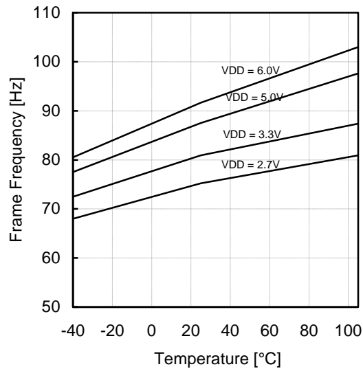
Figure 6. フレーム周波数温度特性(Typ)
