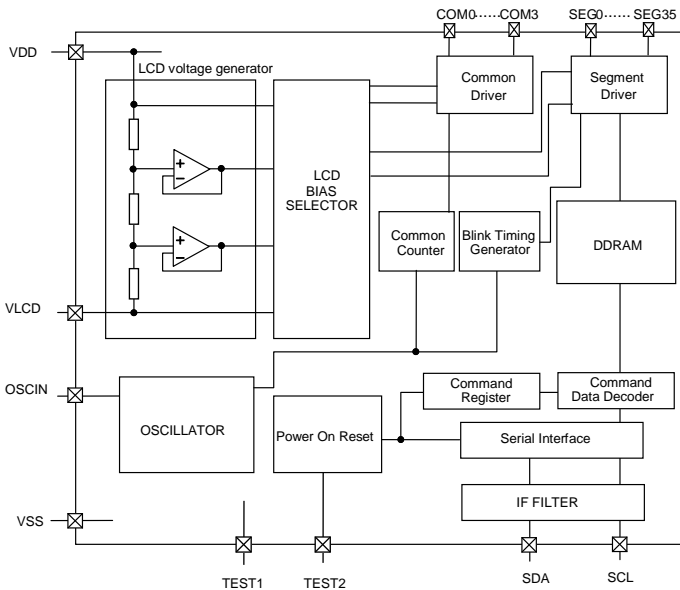
Figure 2. ブロック図
