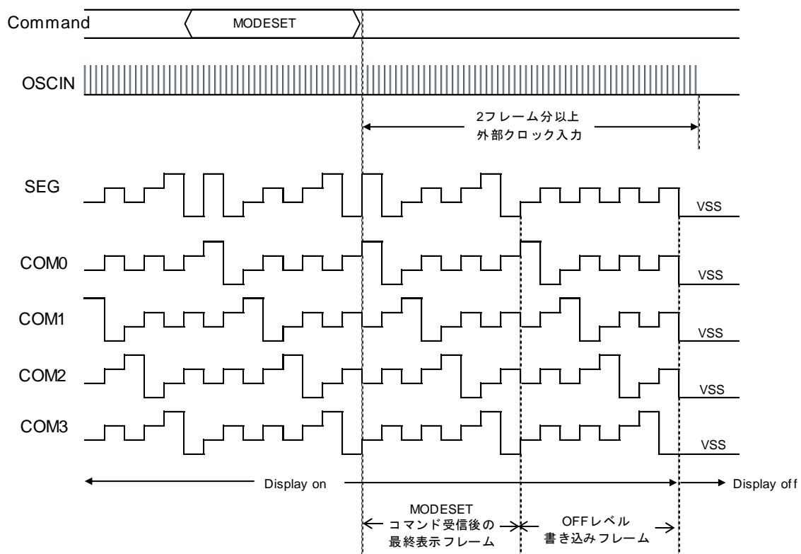
Figure 25. 外部クロック停止タイミング
