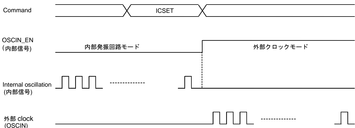
Figure 15. OSC MODE 切り替えタイミング
