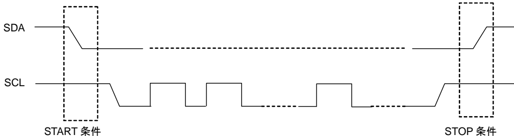
Figure 10. 2 線シリアルインタフェース Command / Data 転送フォーマット
