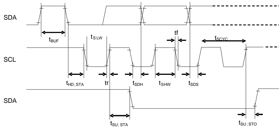
Figure 7. インタフェースタイミング
