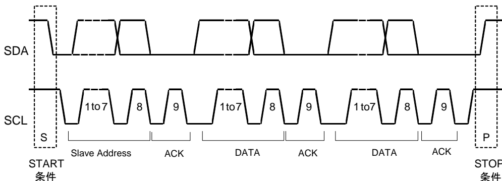
Figure 12. Acknowledge タイミング
