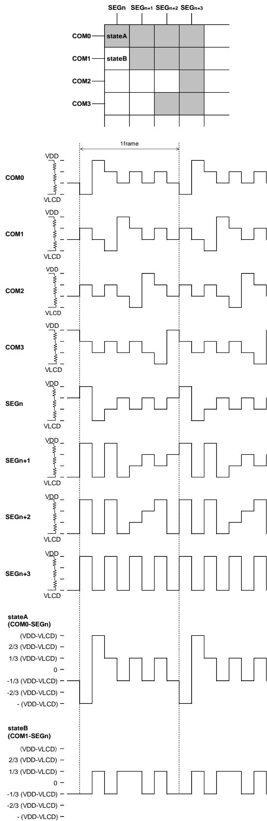
Figure 16. ライン反転時液晶駆動波形図(1/3bias)
