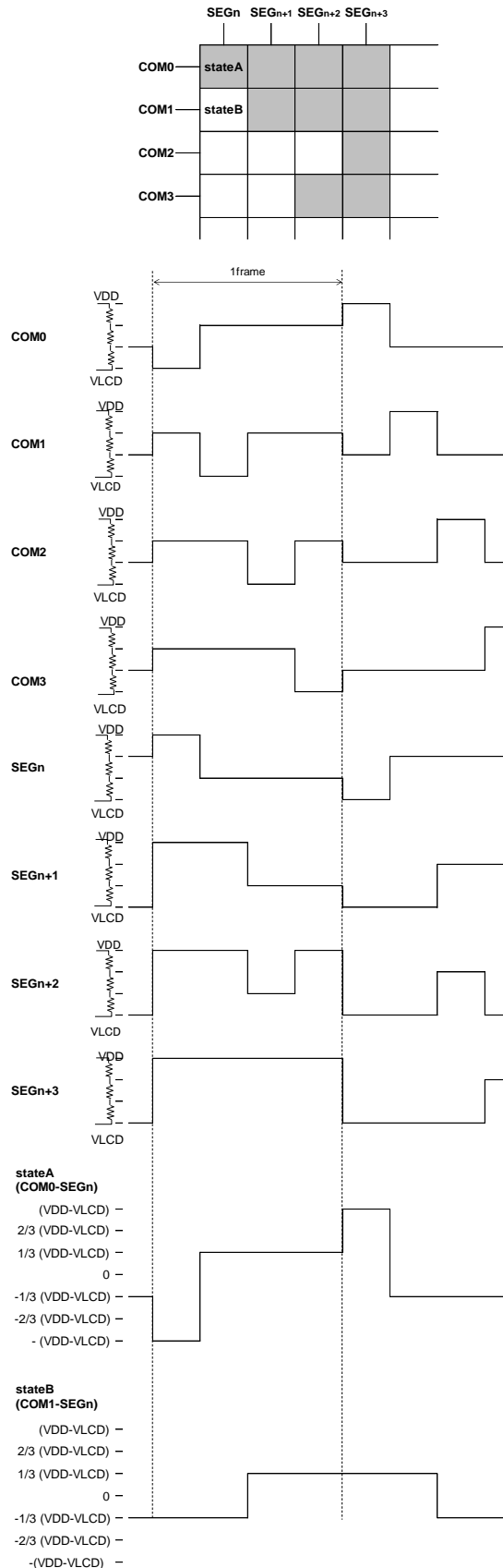
Figure 17. フレーム反転時液晶駆動波形図(1/3bias)
