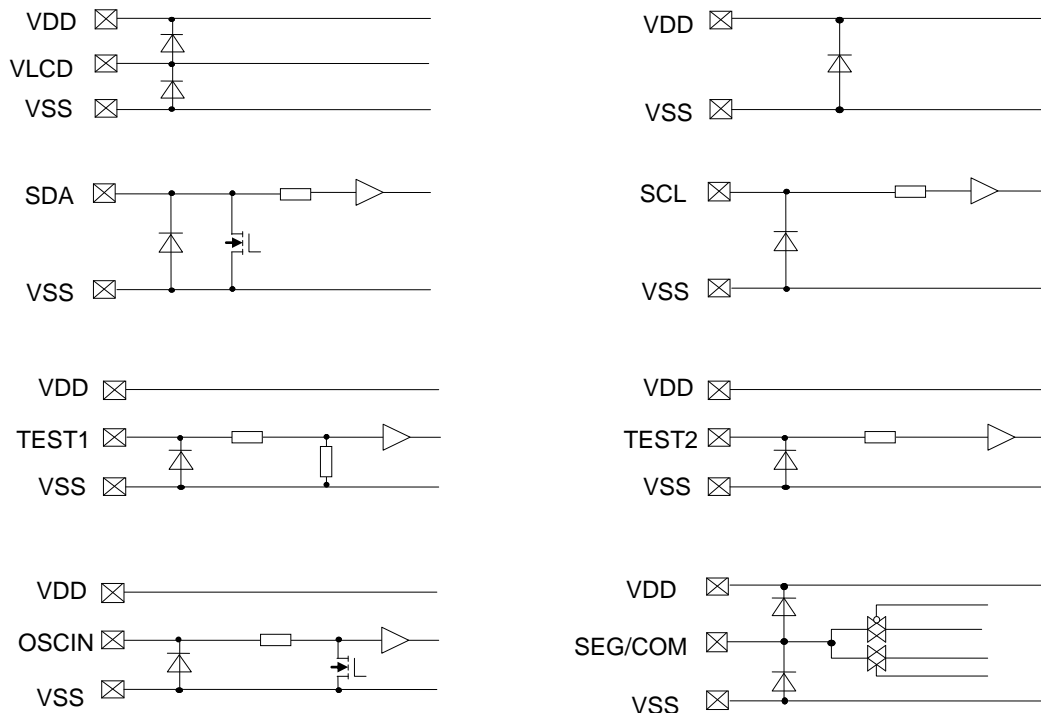
Figure 8 入出力等価回路図
