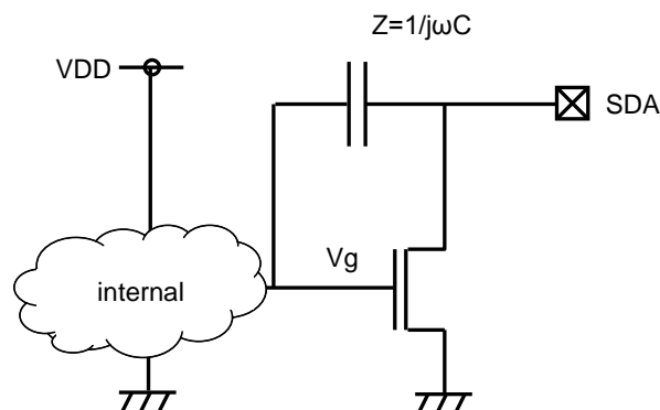
Figure 27. SDA 出力セル構造
