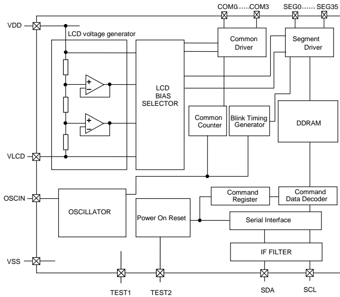
Figure 4. ブロック図
