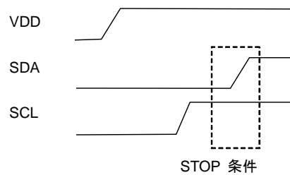
Figure 22. STOP 条件タイミング
