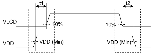
Figure 21. 電源 on/off 波形
