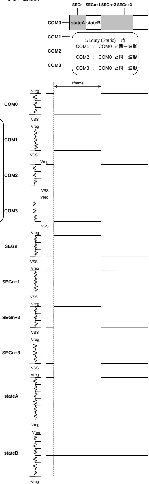
Figure 16. フレーム反転時液晶駆動波形図
