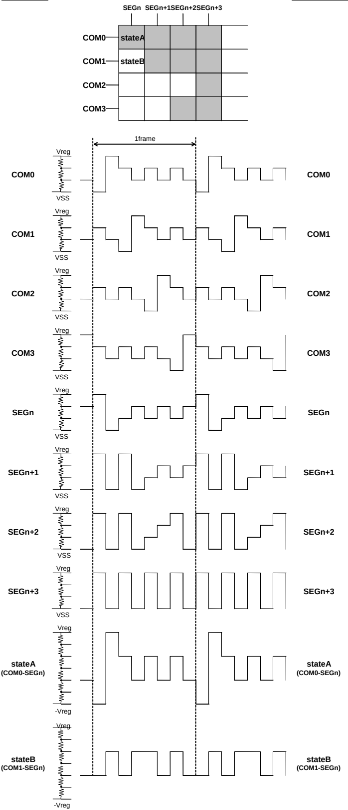
Figure 11. ライン反転時液晶駆動波形図
