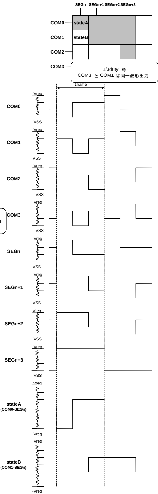
Figure 14. フレーム反転時液晶駆動波形図
