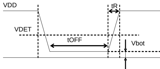
Figure 17. 立ち上がり波形
