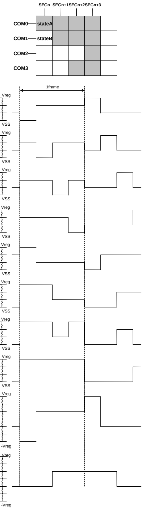
Figure 12. フレーム反転時液晶駆動波形図
