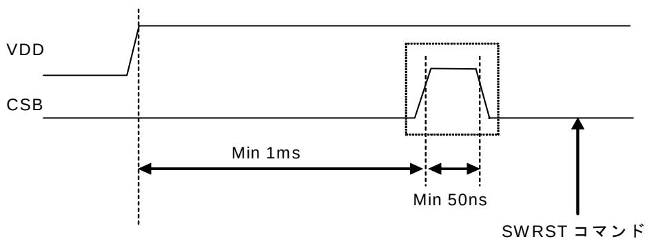
Figure 18. SWRST コマンド Sequence
