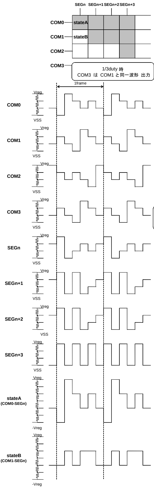
Figure 13. ライン反転時液晶駆動波形図
