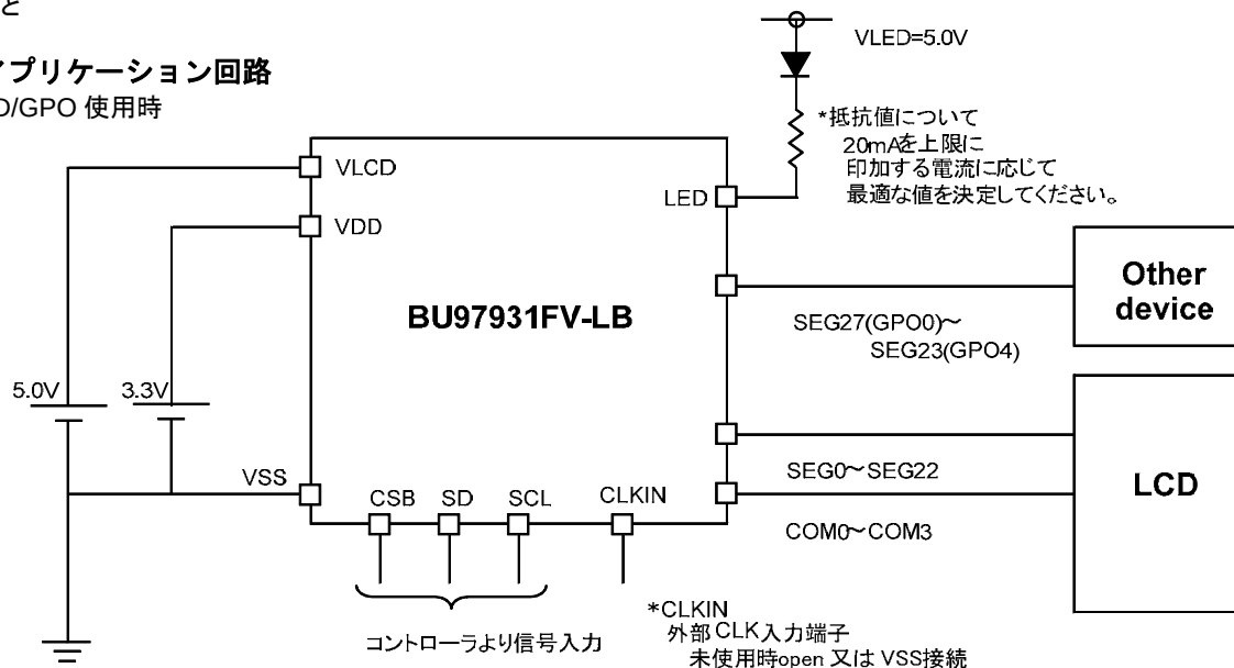
Figure 1. 基本アプリケーション回路
