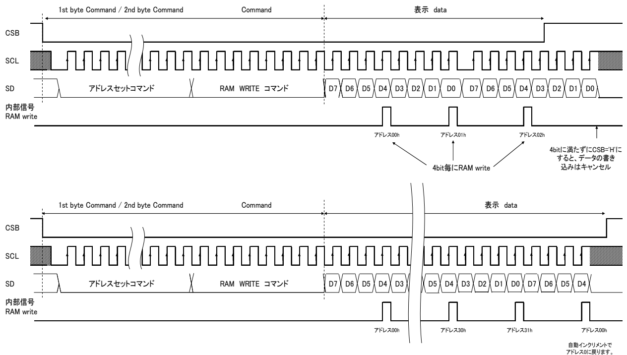
Figure 8. 表示 Data 転送方法
