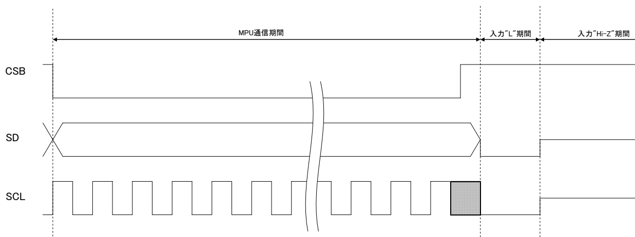
Figure 19. 入力端子 Pull down 時推奨シーケンス
