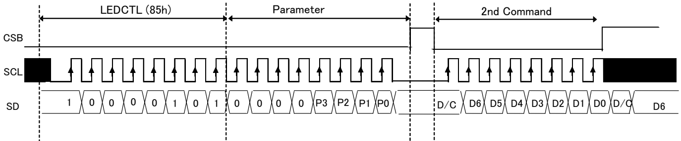
Figure 18. LEDCTL コマンド入力推奨シーケンス
