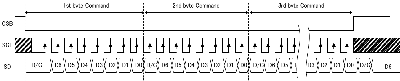
Figure 7. 3-SPI Data 転送 Format
