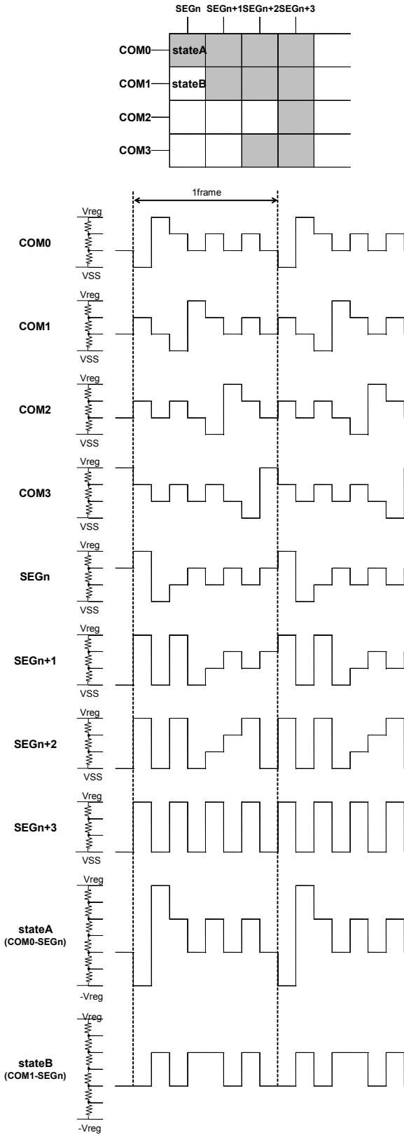
Figure 9. ライン反転時液晶駆動波形図
