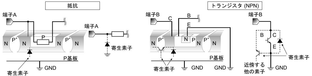
Figure 8. IC 構造例
