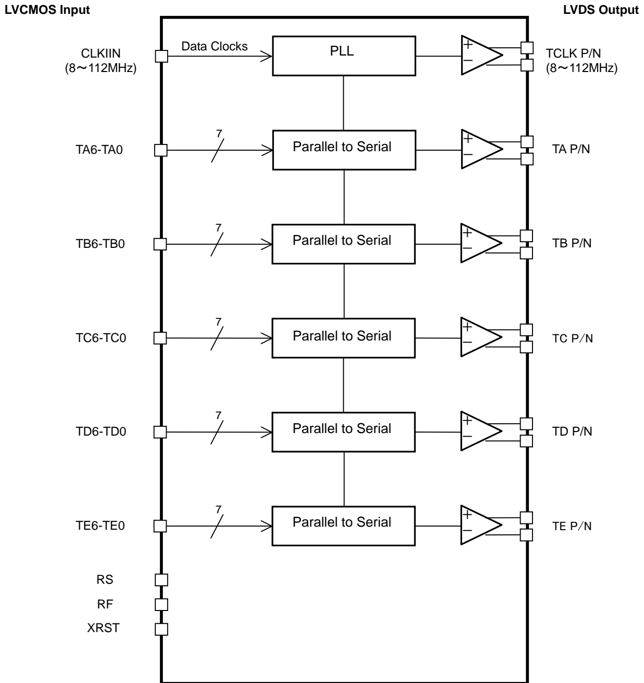
Fig.1 ブロック図
