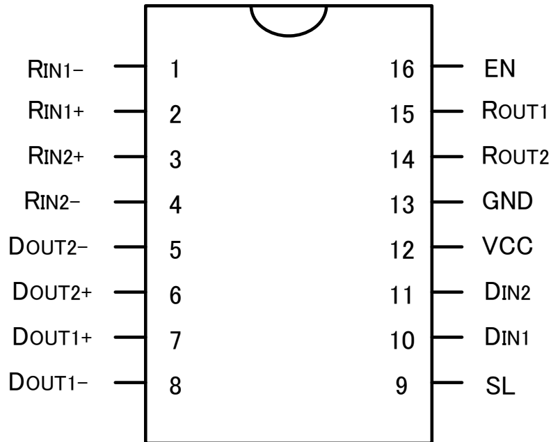
図-3 端子配置図 (Top View)
