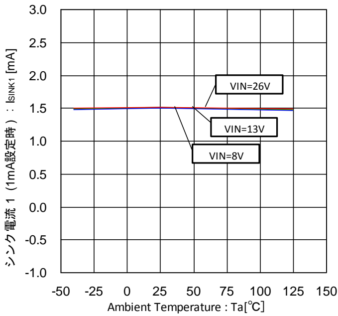
Figure 37. シンク電流 1-温度特性 (1mA 設定時)
