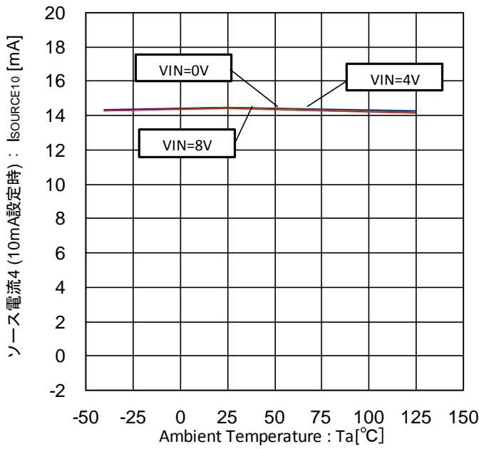
Figure 57. ソース電流 4 -温度特性 (10mA 設定時)
