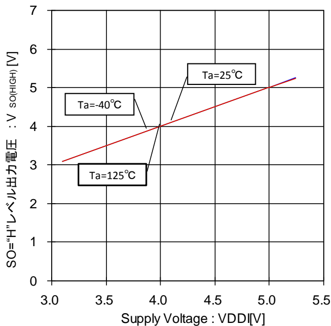
Figure 90. SO="H"レベル出力電圧-電圧特性 (Isource=200 \mu A)
