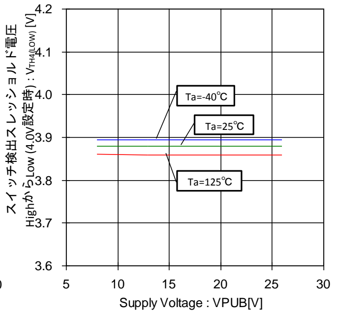
Figure 78. スイッチ検出スレッシュヨルド電圧 High から Low-電圧特性(4.0V 設定時)
