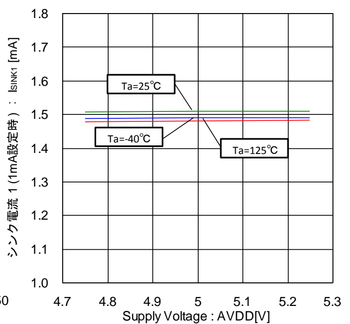
Figure 36. シンク電流 1 -電圧特性 (1mA 設定時、外部から 8V 印加)
