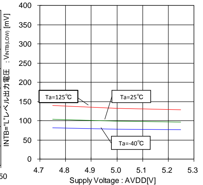
Figure 104. INTB="L"レベル出力電圧-電圧特性 (I SINK =1.0mA)
