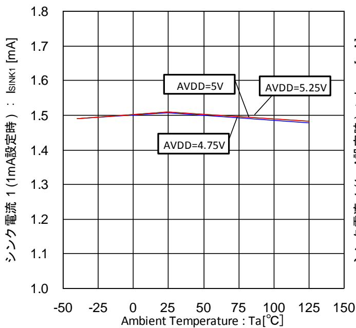
Figure 35. シンク電流 1-温度特性 (1mA 設定時、外部から 8V 印加)
