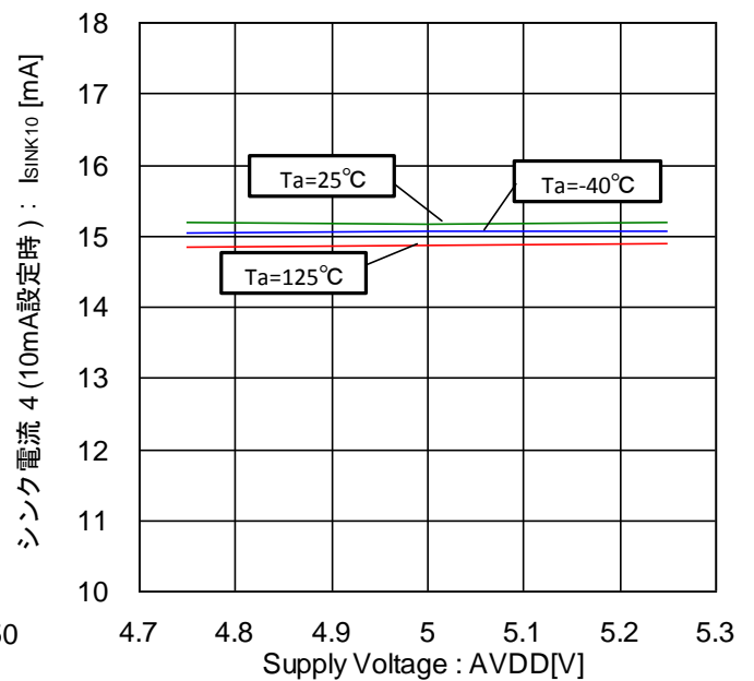
Figure 60. シンク電流 4 -電圧特性 (10mA 設定時、外部から 8V 印加)
