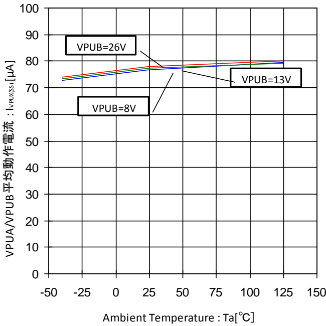
Figure 25. VPUA/VPUB 平均動作電流-温度特性 (監視周期 : 50ms、ストロープ時間 : 125 \mu\text{s} 、 ソース電流設定 : 1mA)
