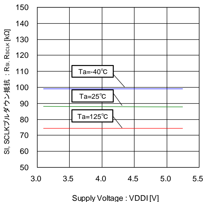
Figure 86. SI, SCLK プルダウン抵抗-電圧特性
