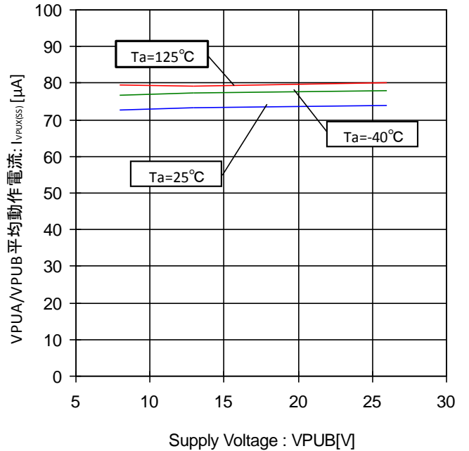
Figure 26. VPUA/VPUB 平均動作電流-電圧特性 (監視周期 : 50ms、ストロープ時間 : 125 \mu\text{s} 、 ソース電流設定 : 1mA)
