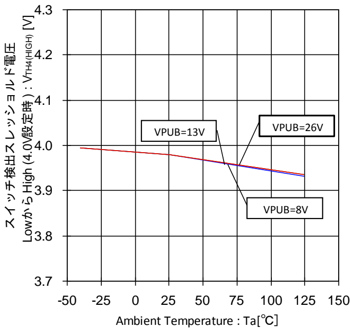
Figure 75. スイッチ検出スレッシュヨルド電圧 Low から High-温度特性(4.0V 設定時)
