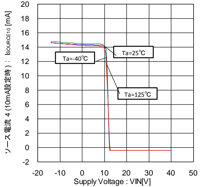
Figure 58. ソース電流 4 -電圧特性 (10mA 設定時)
