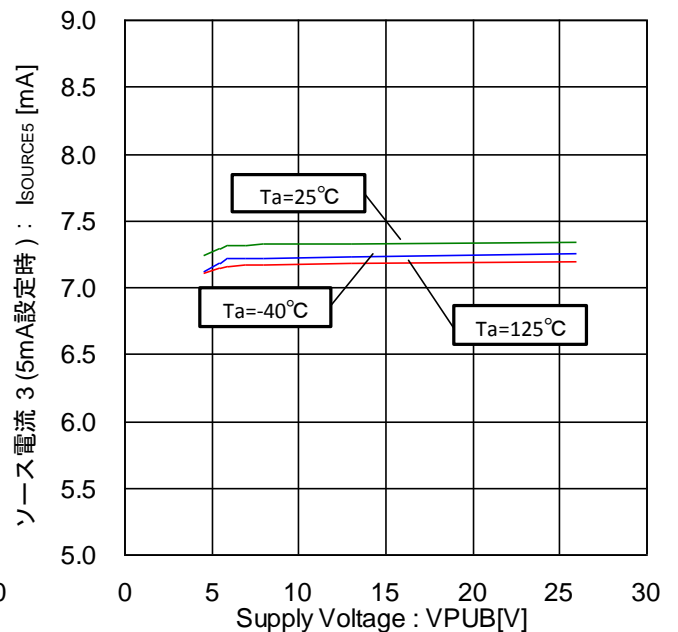
Figure 48. ソース電流 3 -電圧特性 (5mA 設定時、外部から 0V 印加)
