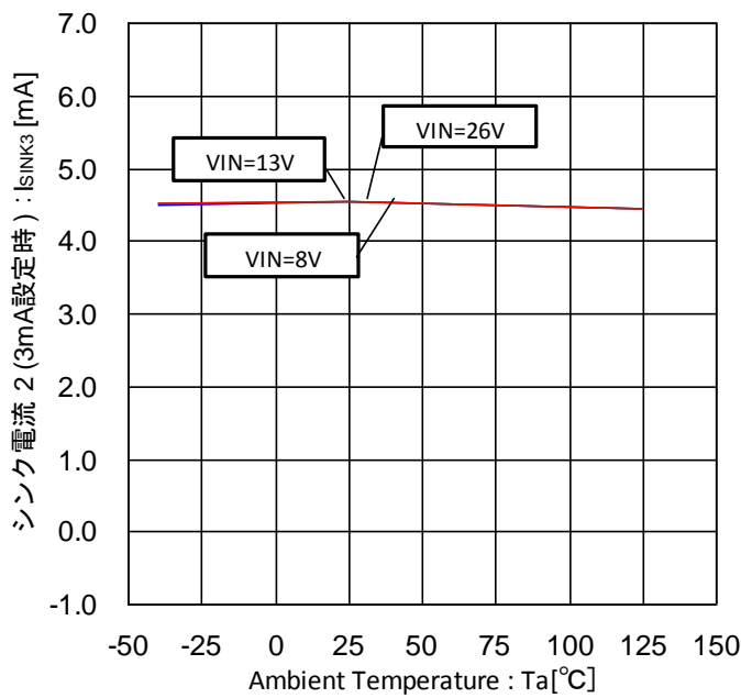
Figure 45. シンク電流 2 -温度特性 (3mA 設定時)
