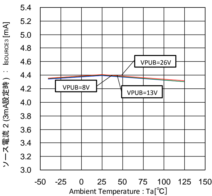
Figure 39. ソース電流 2 -温度特性 (3mA 設定時、外部から 0V 印加)
