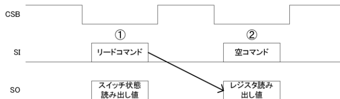
Figure 11. 単独読み出し
