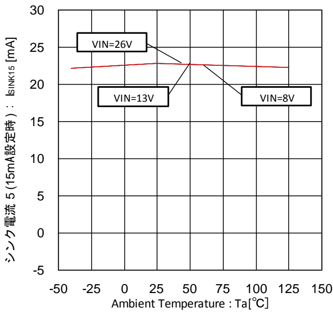
Figure 69. シンク電流 5 -温度特性 (15mA 設定時)
