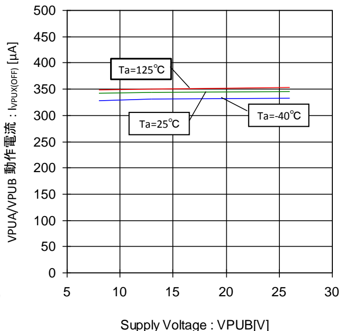
Figure 24. V_{PUA}/V_{PUB} 動作電流-電圧特性 (常時監視設定、電流源無効、“Hi-Z”状態)
