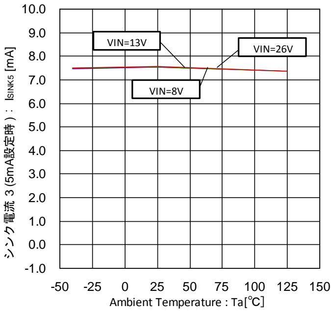
Figure 53. シンク電流 3-温度特性 (5mA 設定時)
