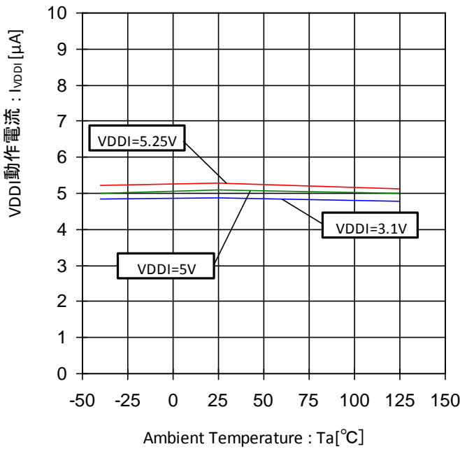
Figure 27. VDDI 動作電流-温度特性 (INTB="H", CSB="H"時)
