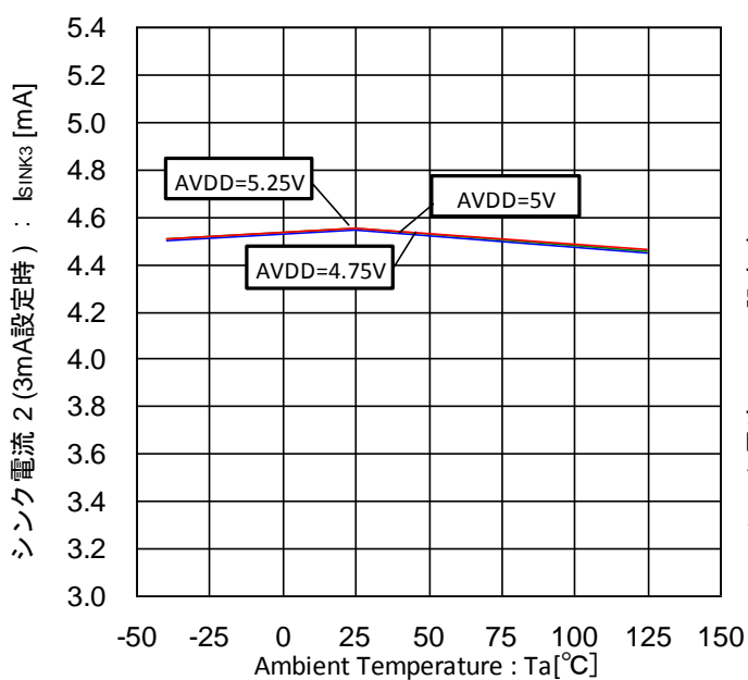
Figure 43. シンク電流 2-温度特性 (3mA 設定時、外部から 8V 印加)
