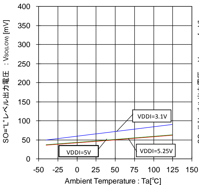
Figure 91. SO="L"レベル出力電圧-温度特性 (ISINK=1.6mA)
