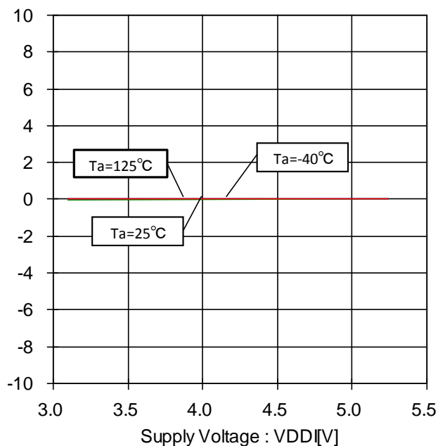
Figure 94. SO("Hi-Z"時)入力電流-電圧特性
