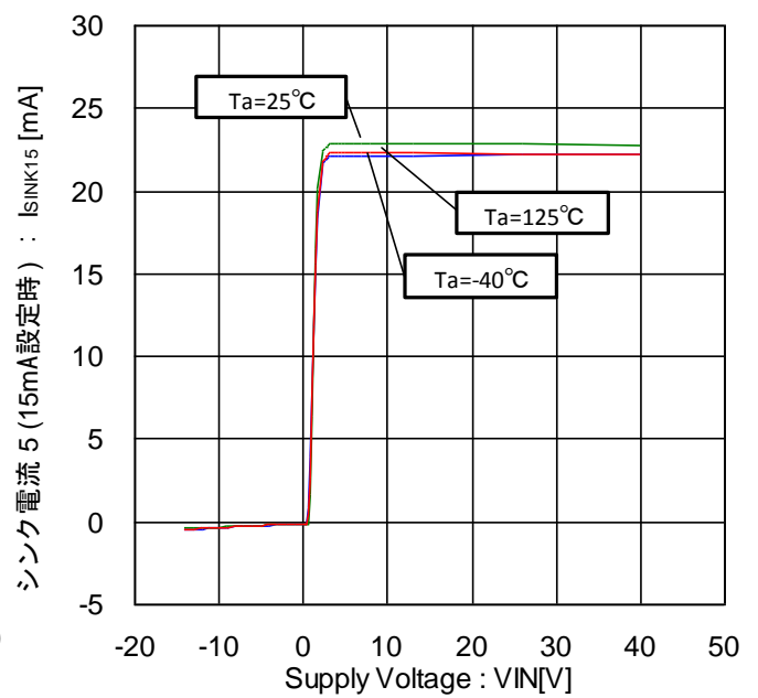
Figure 70. シンク電流 5 -電圧特性 (15mA 設定時)
