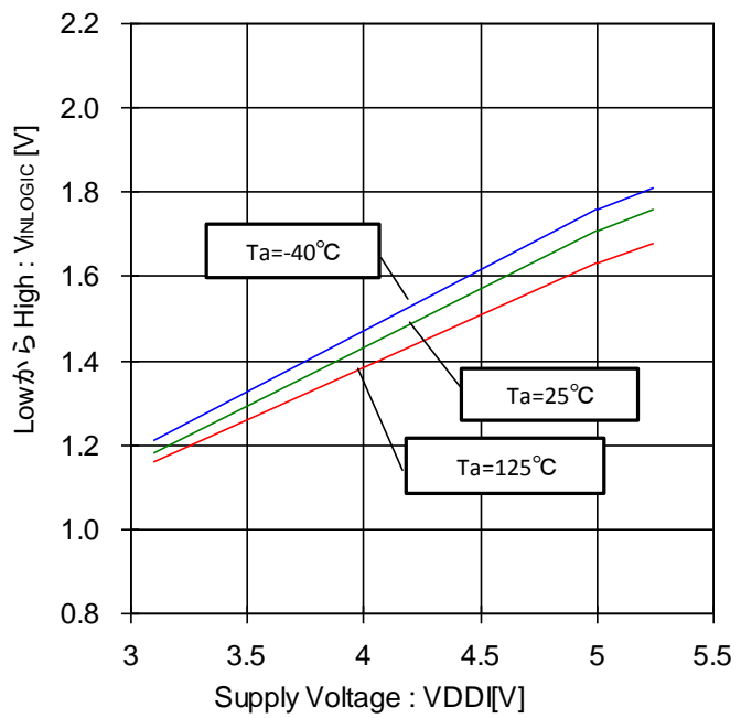
Figure 80. シリアルインタフェーススレッシュヨルド電圧 Low から High-電圧特性
