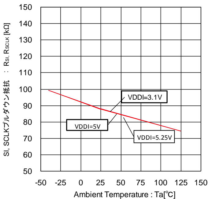
Figure 85. SI, SCLK プルダウン抵抗-温度特性
