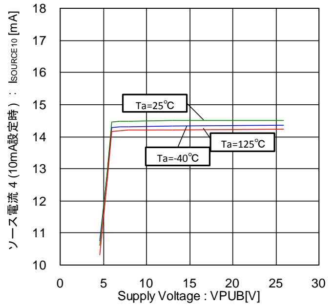
Figure 56. ソース電流 4-電圧特性 (10mA 設定時、外部から 0V 印加)
