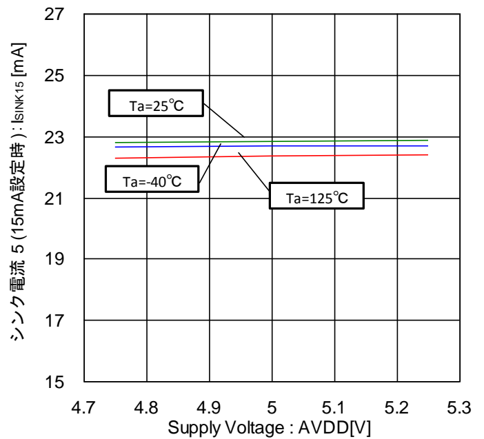
Figure 68. シンク電流 5 -電圧特性 (15mA 設定時、外部から 8V 印加)
