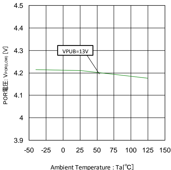
Figure 21. POR(パワーオンリセット)電圧-温度特性
