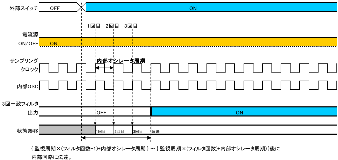
Figure 19. 常時監視設定時の 3 回一致フィルタ動作例
