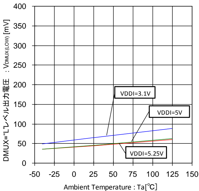
Figure 97. DMUX="L" レベル出力電圧-温度特性 (ISINK=1.6mA)
