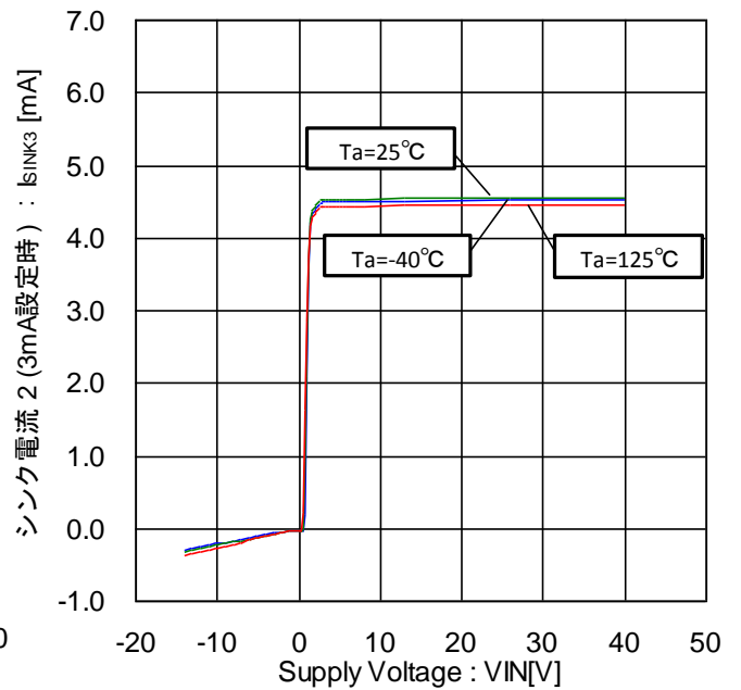
Figure 46. シンク電流 2 -電圧特性 (3mA 設定時)
