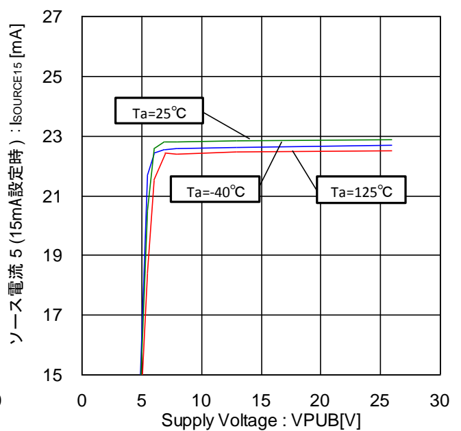
Figure 64. ソース電流 5-電圧特性 (15mA 設定時、外部から 0V 印加)
