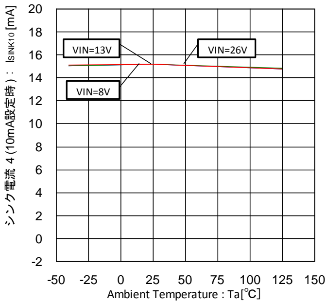
Figure 61. シンク電流 4-温度特性 (10mA 設定時)
