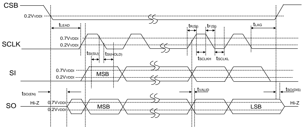
Figure 4. シリアルアクセスタイミング
