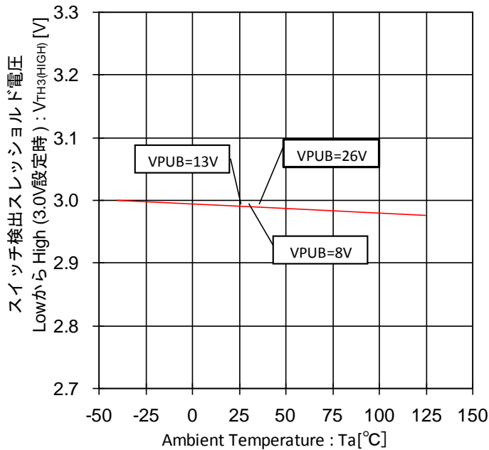
Figure 71. スイッチ検出スレッシュホールド電圧 Low から High -温度特性(3.0V 設定時)
