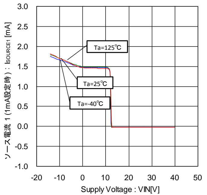
Figure 34. ソース電流 1 -電圧特性 (1mA 設定時)
