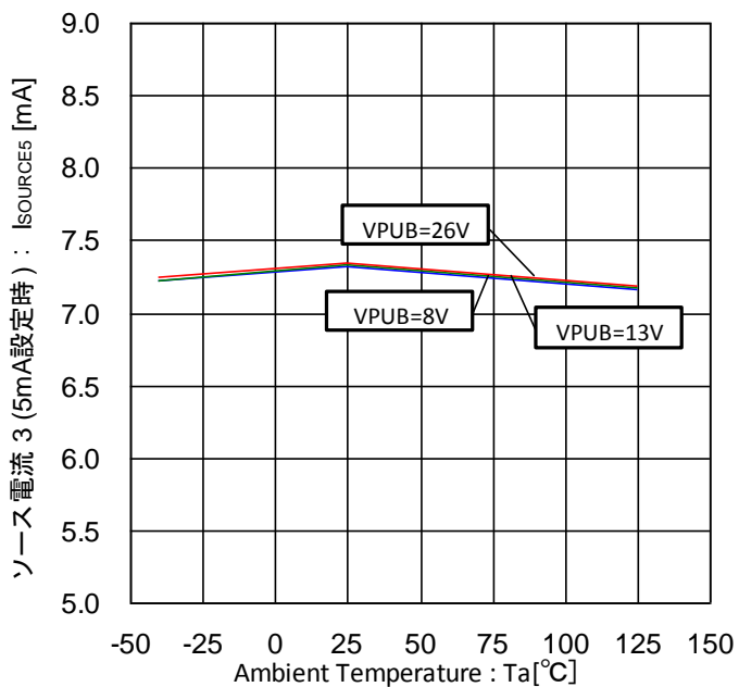
Figure 47. ソース電流 3 -温度特性 (5mA 設定時、外部から 0V 印加)
