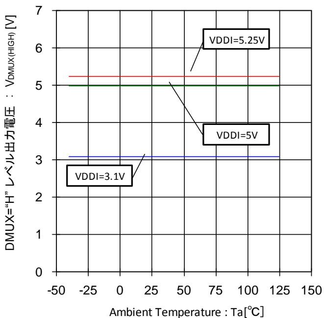
Figure 95. DMUX="H"レベル出力電圧-温度特性 (Isource=200μA)
