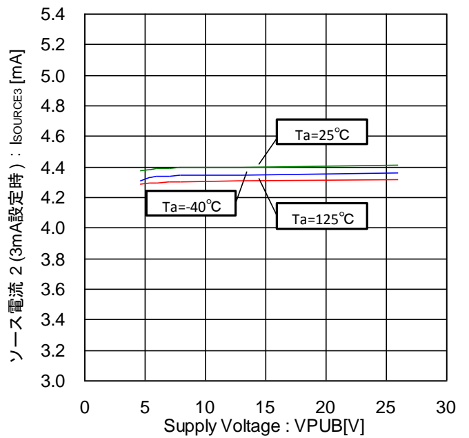
Figure 40. ソース電流 2 -電圧特性 (3mA 設定時、外部から 0V 印加)
