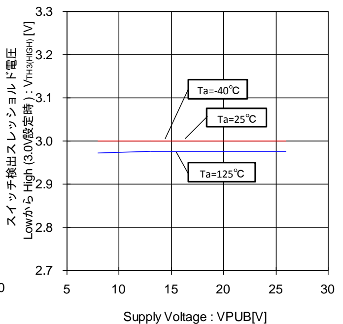
Figure 72. スイッチ検出スレッシュホールド電圧 Low から High -電圧特性(3.0V 設定時)
