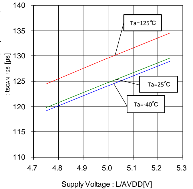
Figure 112. スイッチストロープ時間-電圧特性 (125µs 設定時)
