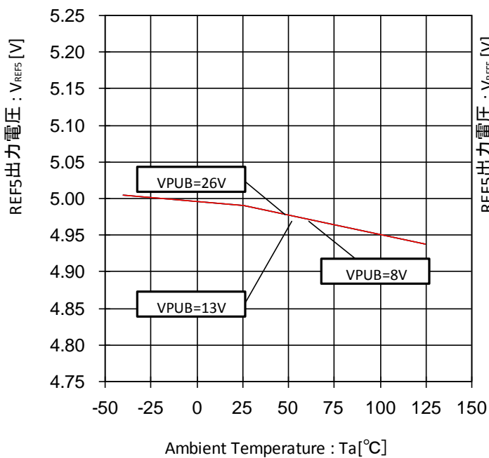
Figure 29. REF5 出力電圧-温度特性
