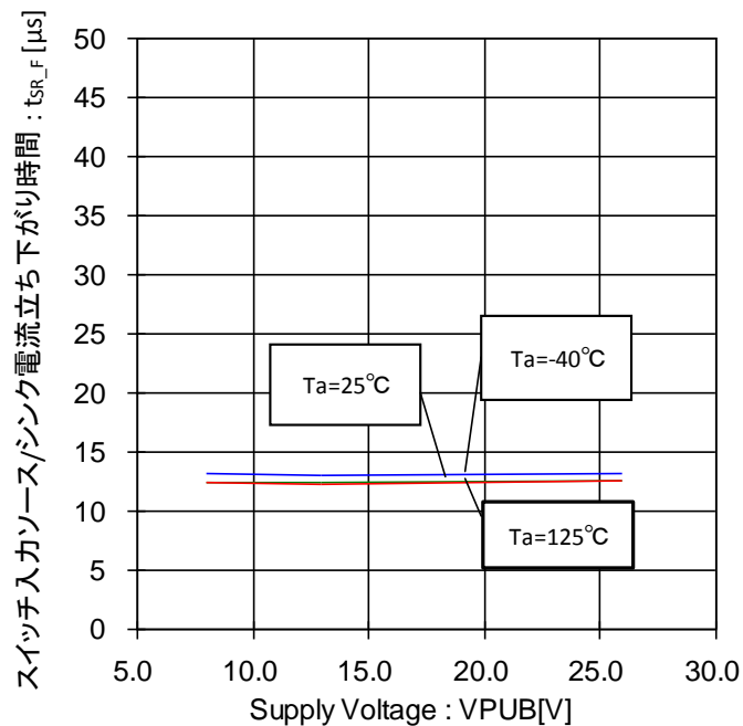
Figure 120. スイッチ入力ソース/シンク電流 立ち下がり時間-電圧特性 (FSQ="0", FSQZ/A/B="0", 10mA 設定時 負荷抵抗 100Ω)
