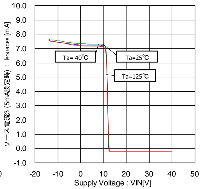
Figure 50. ソース電流 3-電圧特性 (5mA 設定時)
