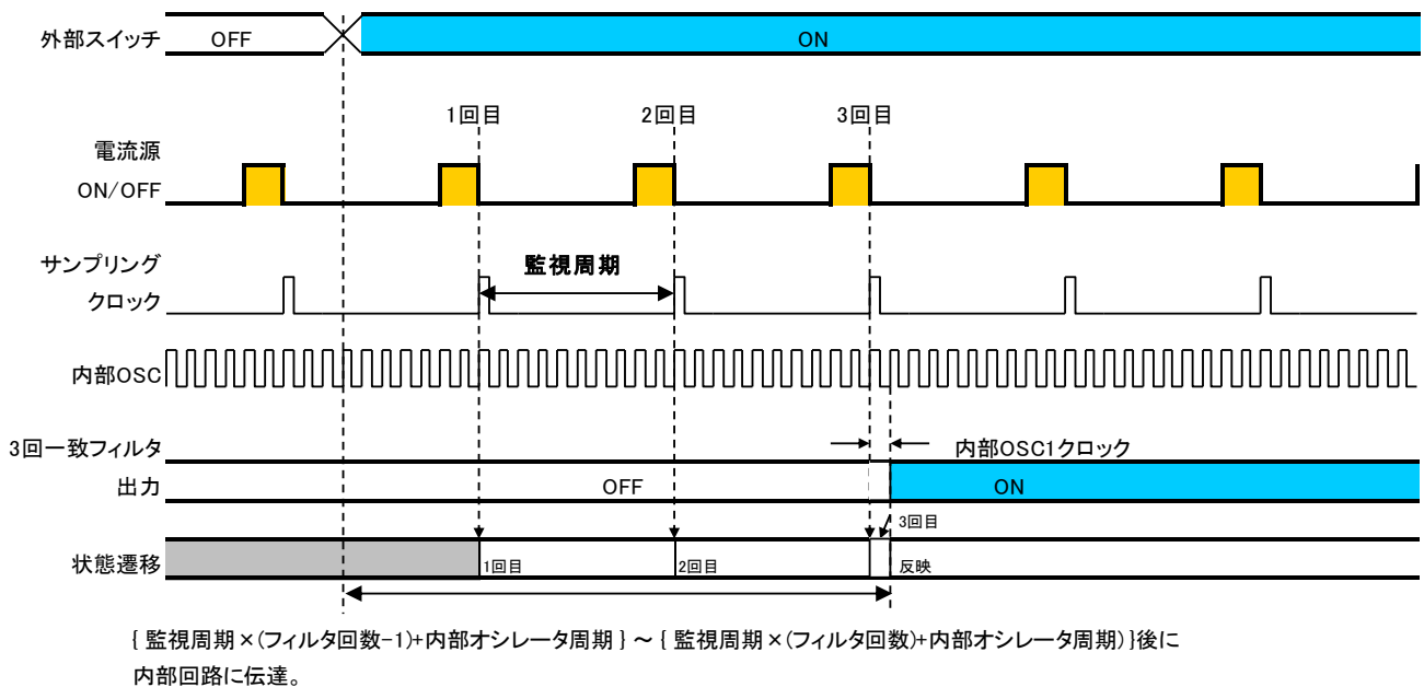
Figure 20. 間欠監視設定時の 3 回一致フィルタ動作例
