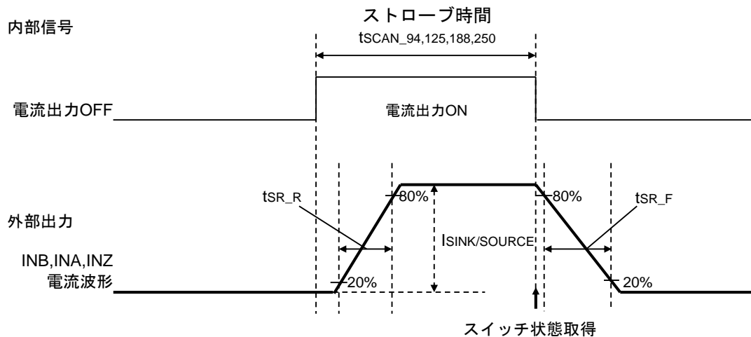
Figure 6. 間欠監視設定(FSQ="0", FSQZ/A/B="0")時のソース/シンク電流立ち上がり/立ち下がり時間
