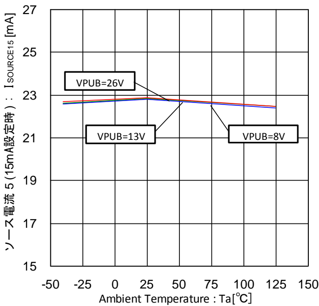
Figure 63. ソース電流 5-温度特性 (15mA 設定時、外部から 0V 印加)
