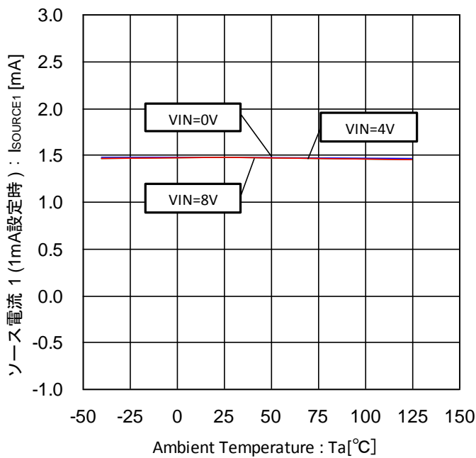
Figure 33. ソース電流 1 -温度特性 (1mA 設定時)
