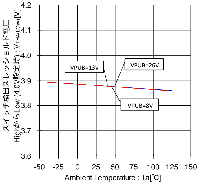
Figure 77. スイッチ検出スレッシュヨルド電圧 High から Low-温度特性(4.0V 設定時)
