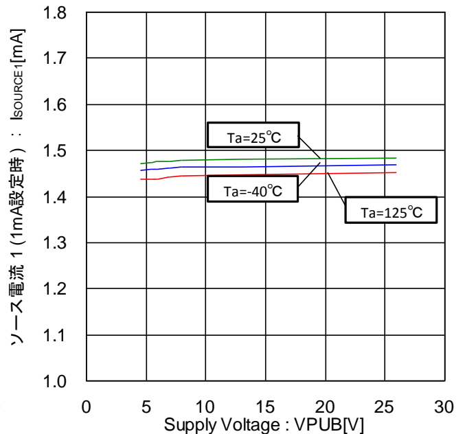
Figure 32. ソース電流 1-電圧特性 (1mA 設定時、外部から 0V 印加)
