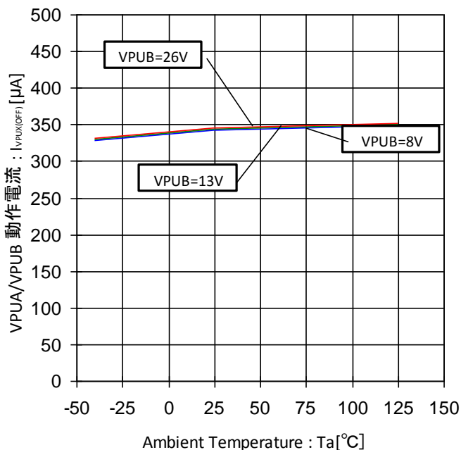
Figure 23. V_{PUA}/V_{PUB} 動作電流-温度特性 (常時監視設定、電流源無効、“Hi-Z”状態)
