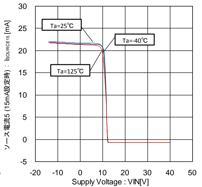
Figure 66. ソース電流 5-電圧特性 (15mA 設定時)
