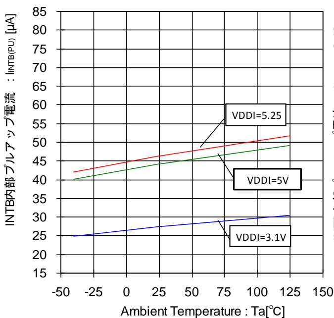
Figure 99. INTB 内部プルアップ電流-温度特性
