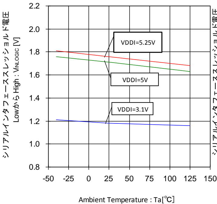
Figure 79. シリアルインタフェーススレッシュヨルド電圧 Low から High-温度特性
