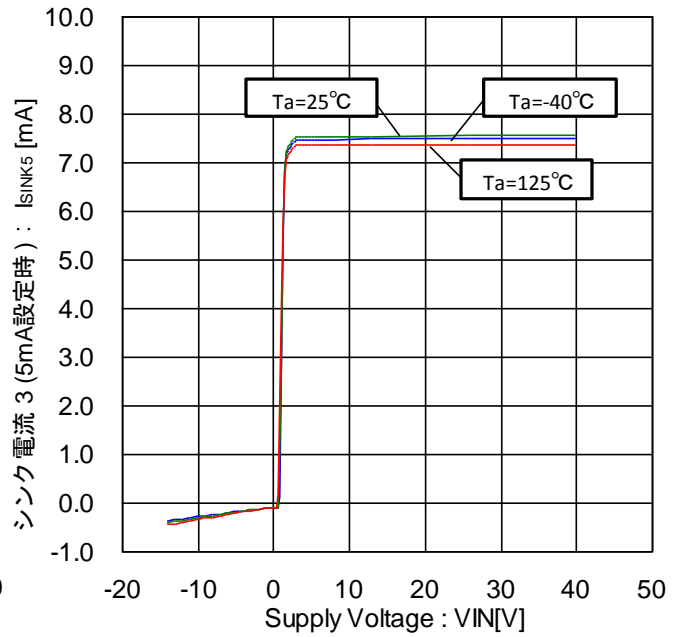
Figure 54. シンク電流 3-電圧特性 (5mA 設定時)
