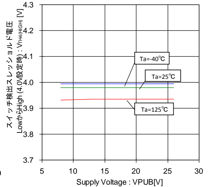
Figure 76. スイッチ検出スレッシュヨルド電圧 Low から High-電圧特性(4.0V 設定時)
