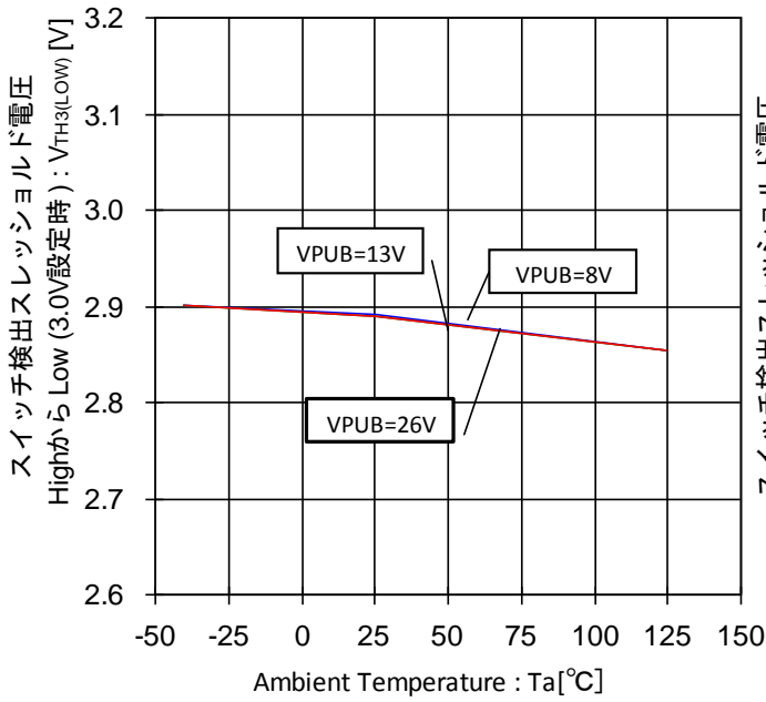
Figure 73. スイッチ検出スレッシュヨルド電圧 High から Low-温度特性(3.0V 設定時)
