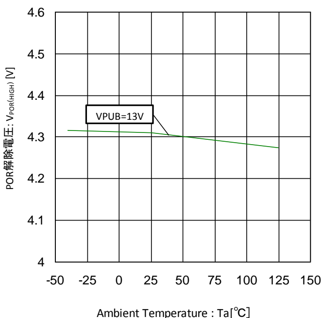
Figure 22. POR(パワーオンリセット)解除電圧-温度特性
