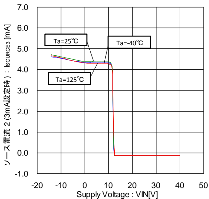
Figure 42. ソース電流 2-電圧特性 (3mA 設定時)
