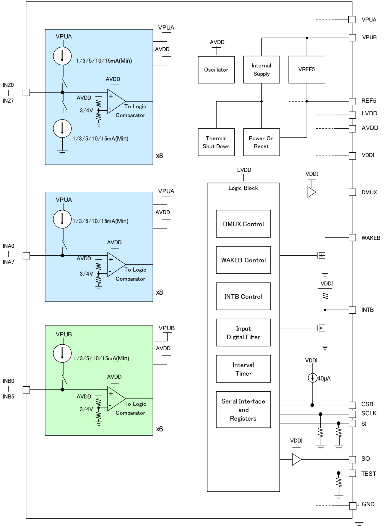
Figure 3. ブロック図
