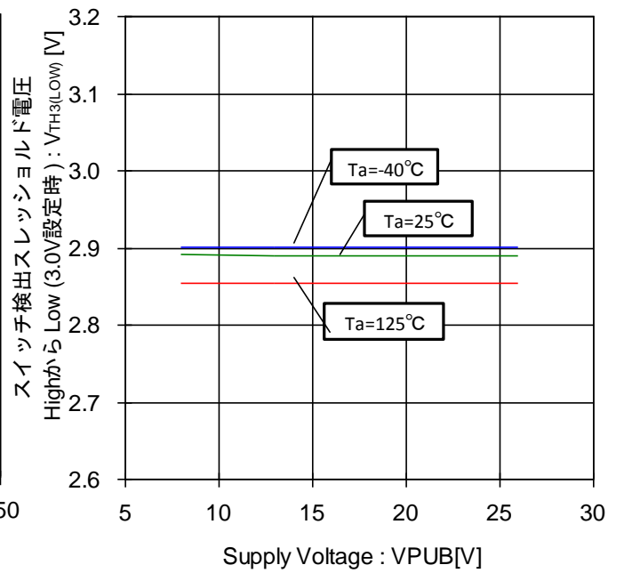
Figure 74. スイッチ検出スレッシュヨルド電圧 High から Low-電圧特性(3.0V 設定時)
