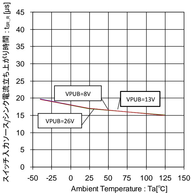
Figure 117. スイッチ入力ソース/シンク電流 立ち上がり時間-温度特性 (FSQ="0", FSQZ/A/B="0", 10mA 設定時 負荷抵抗 100Ω)
