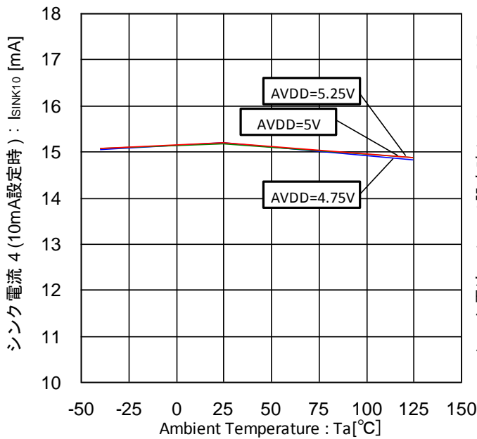
Figure 59. シンク電流 4 -温度特性 (10mA 設定時、外部から 8V 印加)
