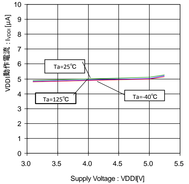
Figure 28. VDDI 動作電流-電圧特性 (INTB="H", CSB="H"時)
