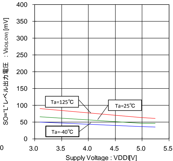
Figure 92. SO="L"レベル出力電圧-電圧特性 (ISINK=1.6mA)
