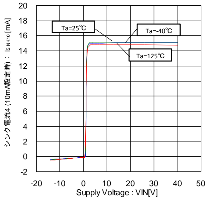
Figure 62. シンク電流 4-電圧特性 (10mA 設定時)
