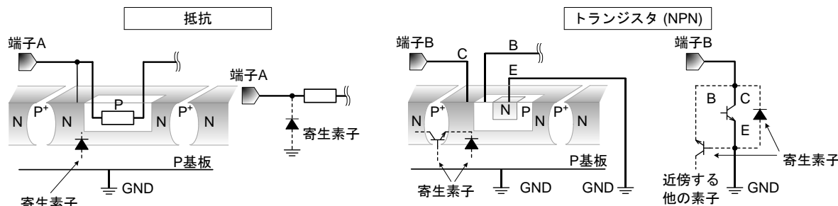
Figure 123. モノリシック IC 構造例
