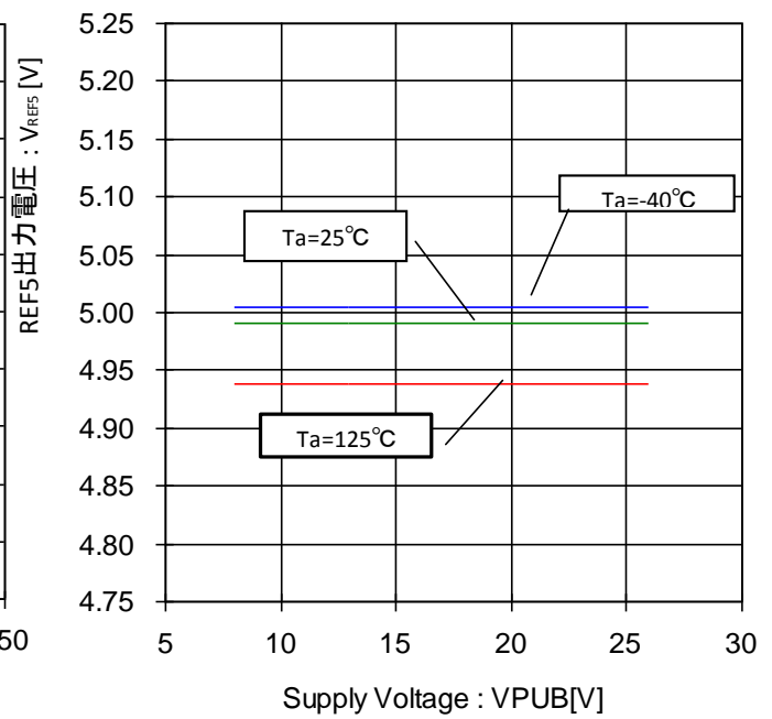
Figure 30. REF5 出力電圧-電圧特性
