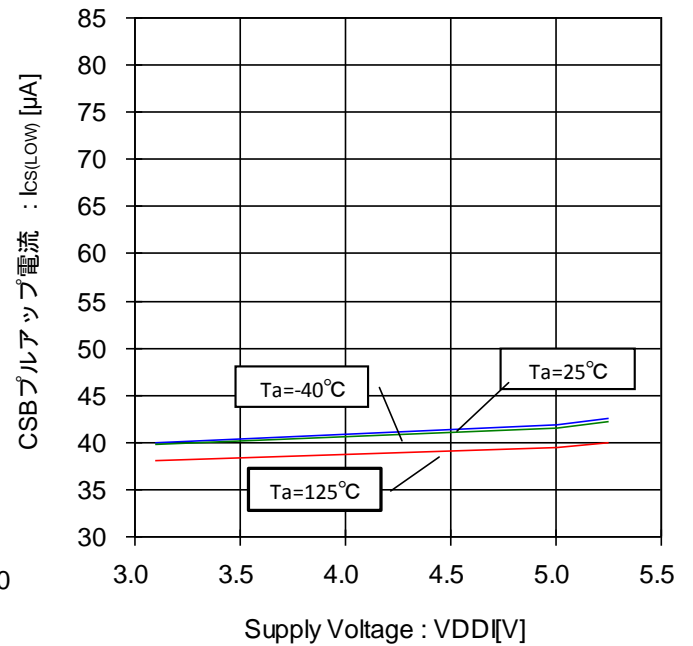
Figure 84. CSB プルアップ電流-電圧特性 (CSB=0V)
