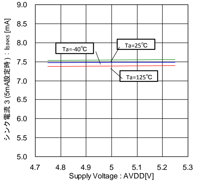
Figure 52. シンク電流 3-電圧特性 (5mA 設定時、外部から 8V 印加)
