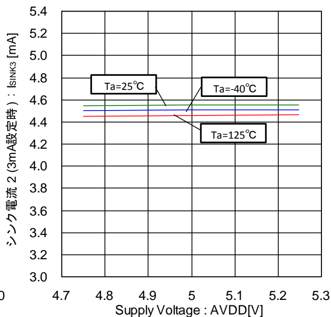
Figure 44. シンク電流 2-電圧特性 (3mA 設定時、外部から 8V 印加)
