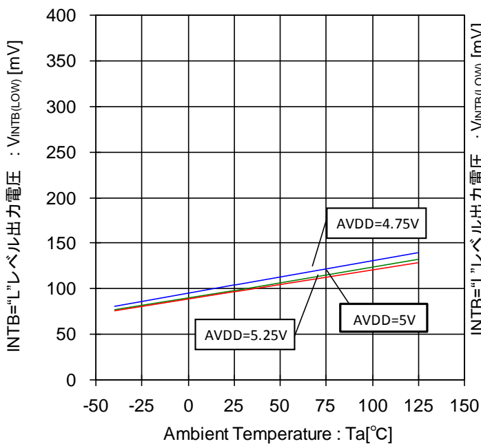
Figure 103. INTB="L"レベル出力電圧-温度特性 (I SINK =1.0mA)
