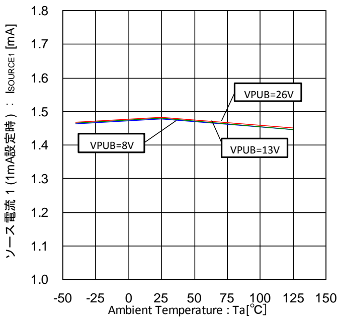
Figure 31. ソース電流 1-温度特性 (1mA 設定時、外部から 0V 印加)
