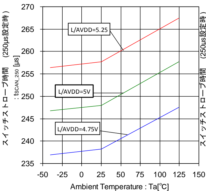
Figure 115. スイッチストロブ時間-温度特性 (250µs 設定時)
