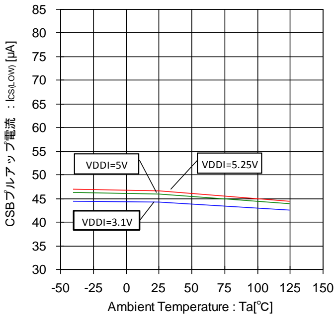
Figure 83. CSB プルアップ電流-温度特性 (CSB=0V)
