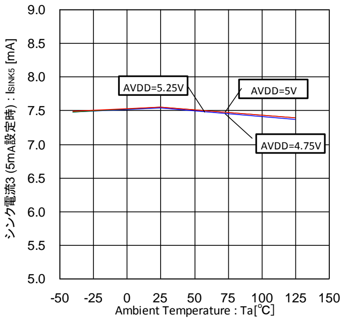
Figure 51. シンク電流 3-温度特性 (5mA 設定時、外部から 8V 印加)
