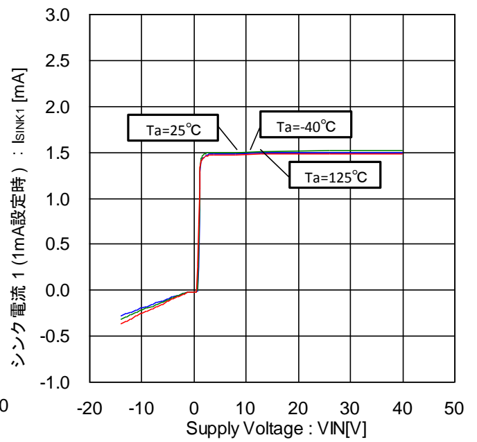
Figure 38. シンク電流 1 -電圧特性 (1mA 設定時)
