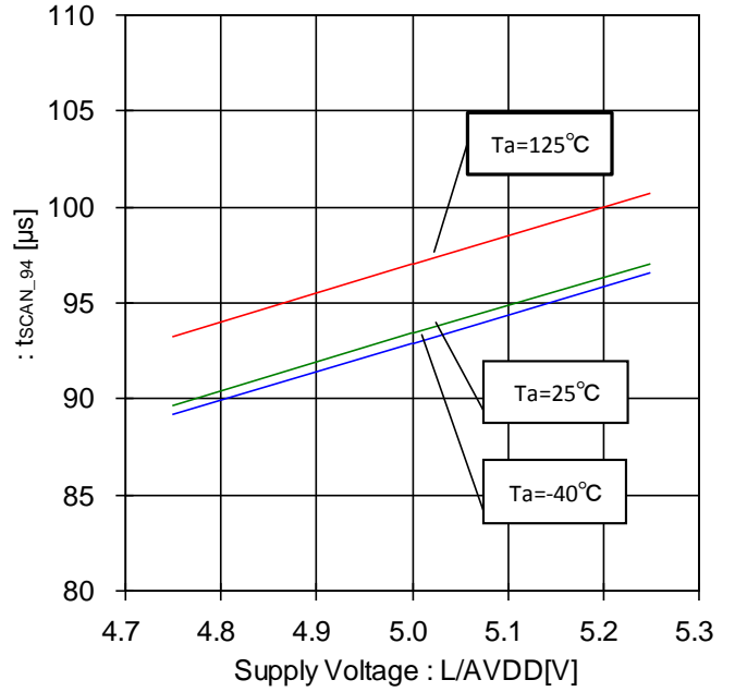
Figure 110. スイッチストロープ時間-電圧特性 (93.75µs 設定時)
