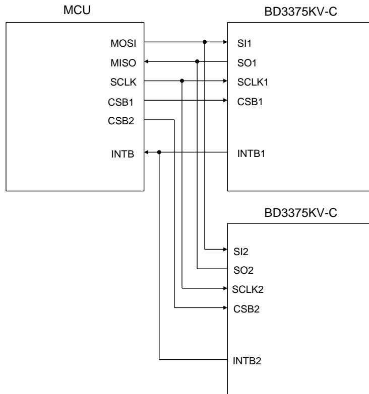
Figure 122. パラレル接続例
