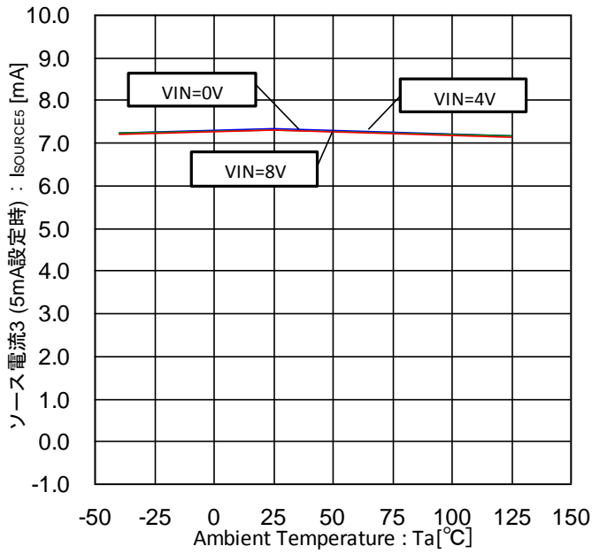
Figure 49. ソース電流 3-温度特性 (5mA 設定時)
