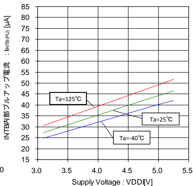
Figure 100. INTB 内部プルアップ電流-電圧特性
