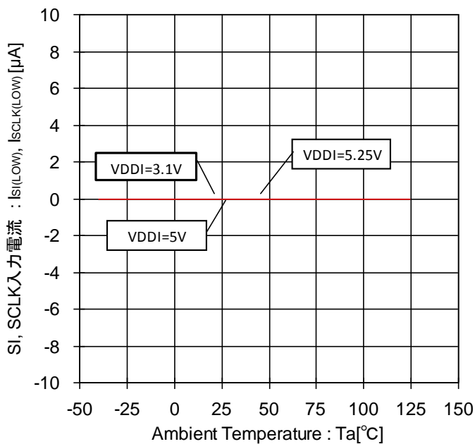
Figure 87. SI, SCLK 入力電流-温度特性 (SI, SCLK=0V)
