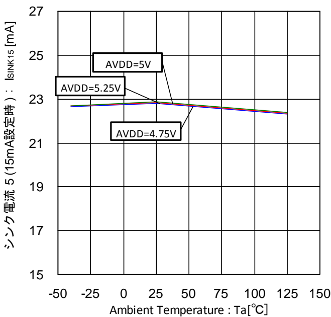
Figure 67. シンク電流 5 -温度特性 (15mA 設定時、外部から 8V 印加)
