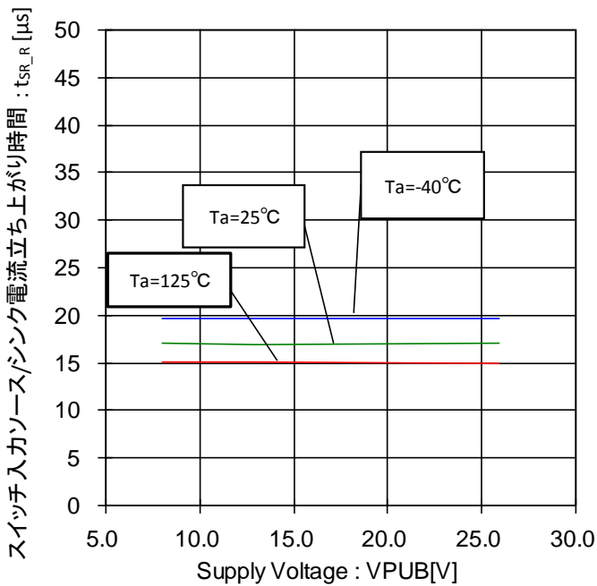
Figure 118. スイッチ入力ソース/シンク電流 立ち上がり時間-電圧特性 (FSQ="0", FSQZ/A/B="0", 10mA 設定時 負荷抵抗 100Ω)
