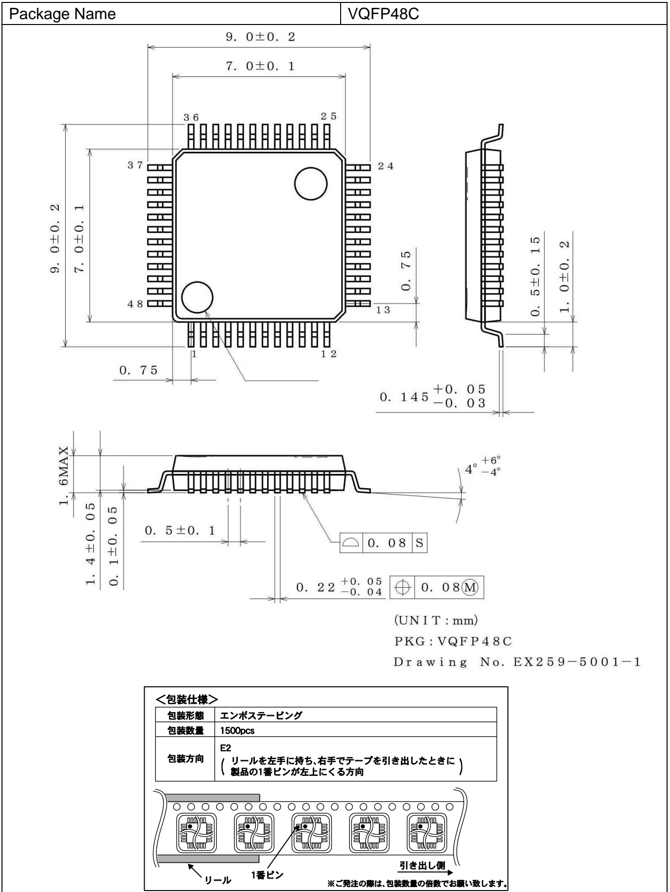
Figure 126. 外形寸法図と包装・フォーミング仕様
