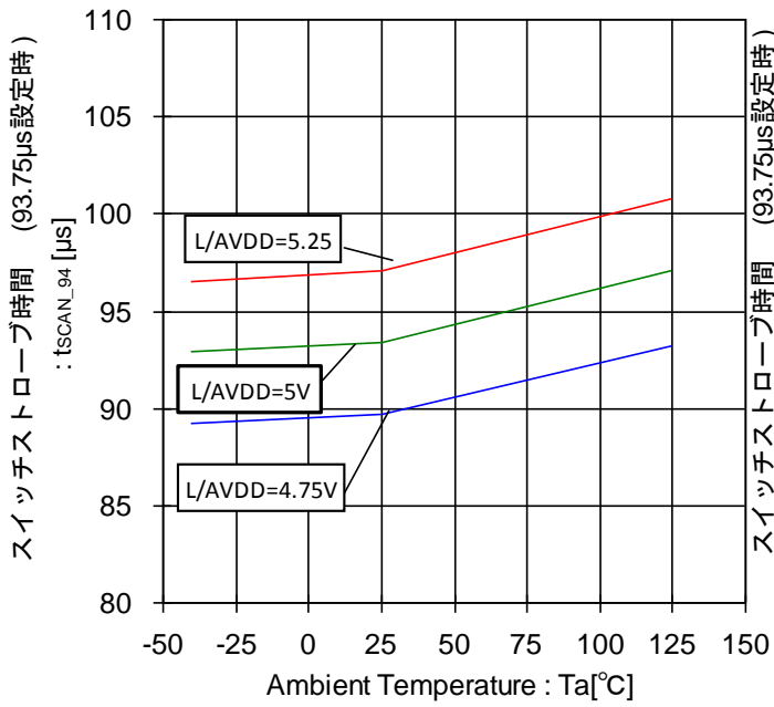
Figure 109. スイッチストロープ時間-温度特性 (93.75µs 設定時)
