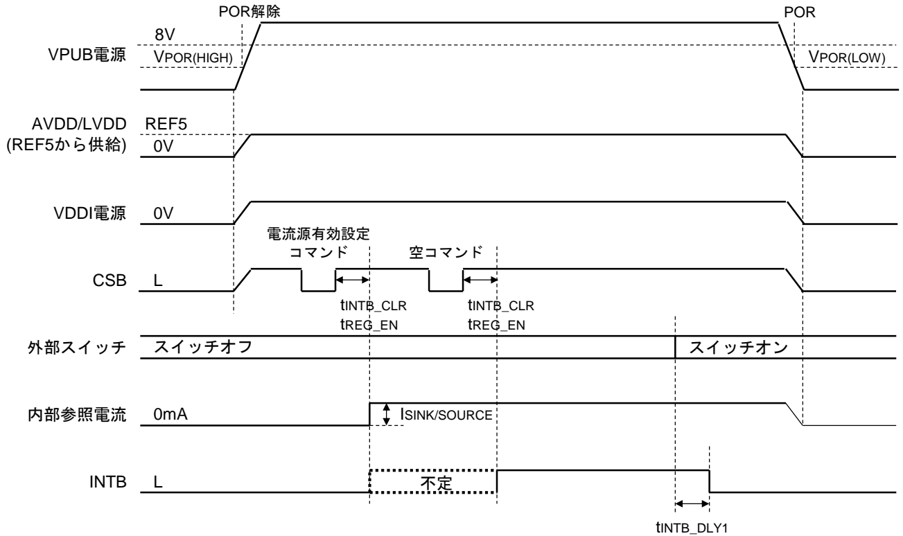
Figure 5.電源立ち上げ/立ち下げシーケンス
