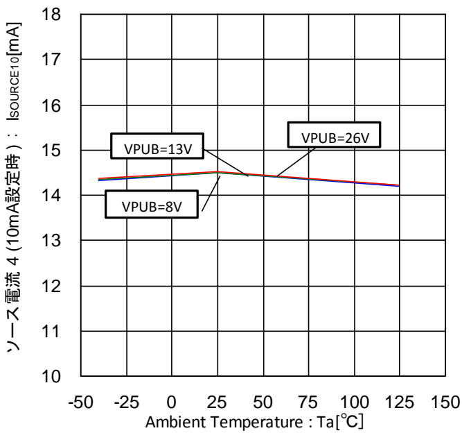
Figure 55. ソース電流 4-温度特性 (10mA 設定時、外部から 0V 印加)
