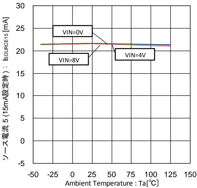
Figure 65. ソース電流 5-温度特性 (15mA 設定時)
