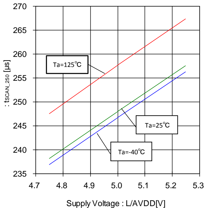
Figure 116. スイッチストロブ時間-電圧特性 (250µs 設定時)
