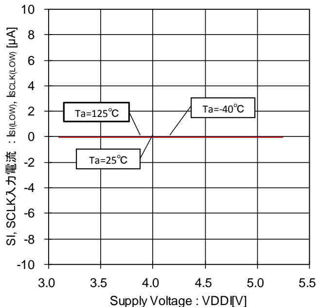
Figure 88. SI, SCLK 入力電流-電圧特性 (SI, SCLK=0V)
