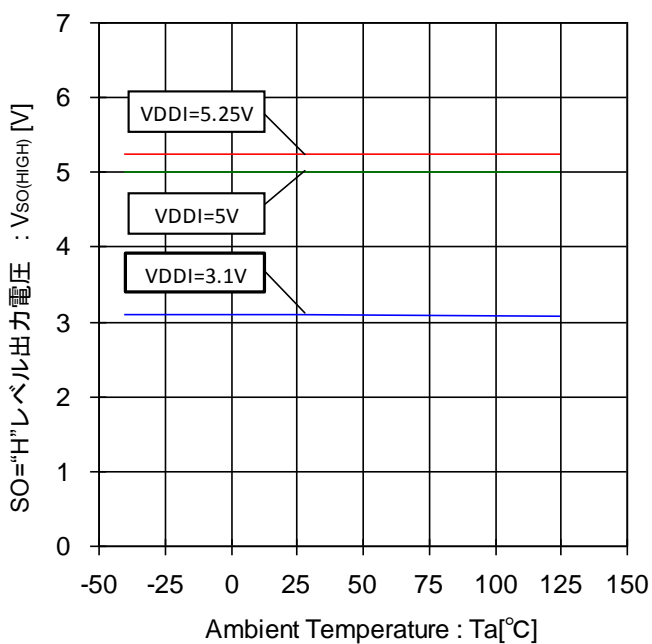
Figure 89. SO="H"レベル出力電圧-温度特性 (Isource=200 \mu A)
