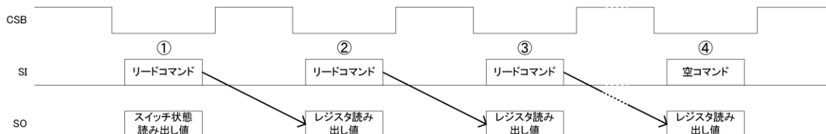
Figure 12. 連続読み出し
