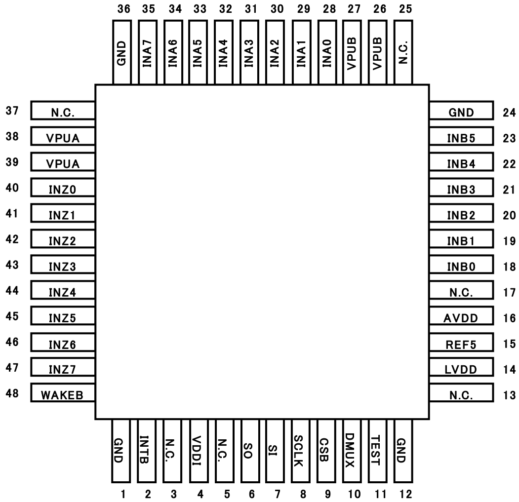
Figure 2. 端子配置图 (Top View)
