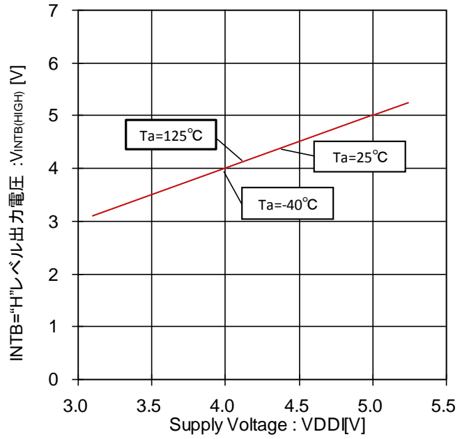
Figure 102. INTB="H"レベル出力電圧-電圧特性 (INTB=OPEN 状態)
