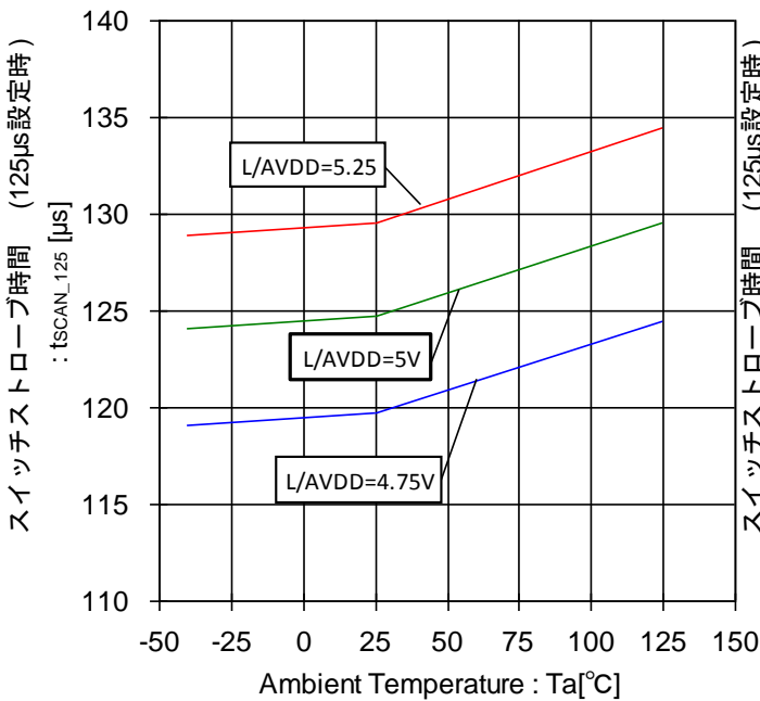
Figure 111. スイッチストロープ時間-温度特性 (125µs 設定時)
