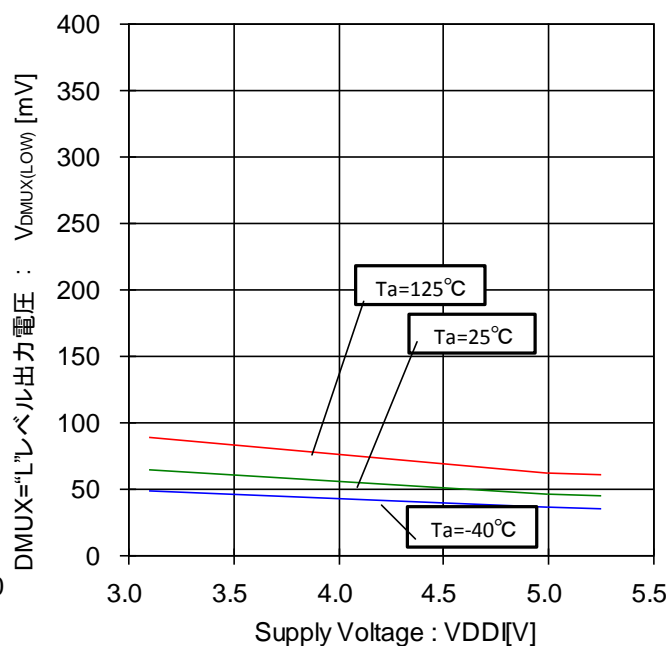
Figure 98. DMUX="L" レベル出力電圧-電圧特性 (ISINK=1.6mA)
