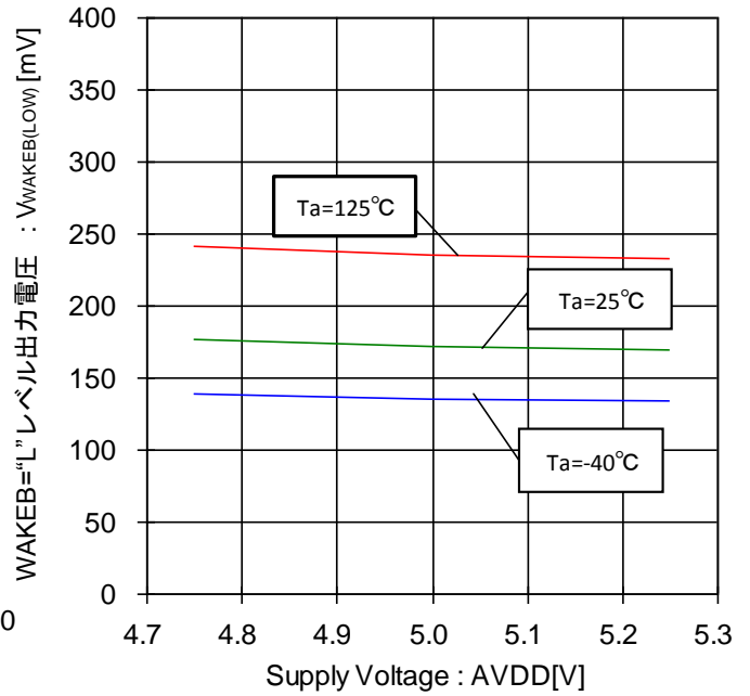
Figure 106. WAKEB="L"レベル出力電圧-電圧特性 (WAKEB=1.0mA)
