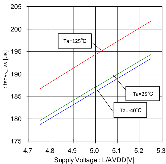
Figure 114. スイッチストロブ時間-電圧特性 (187.5µs 設定時)
