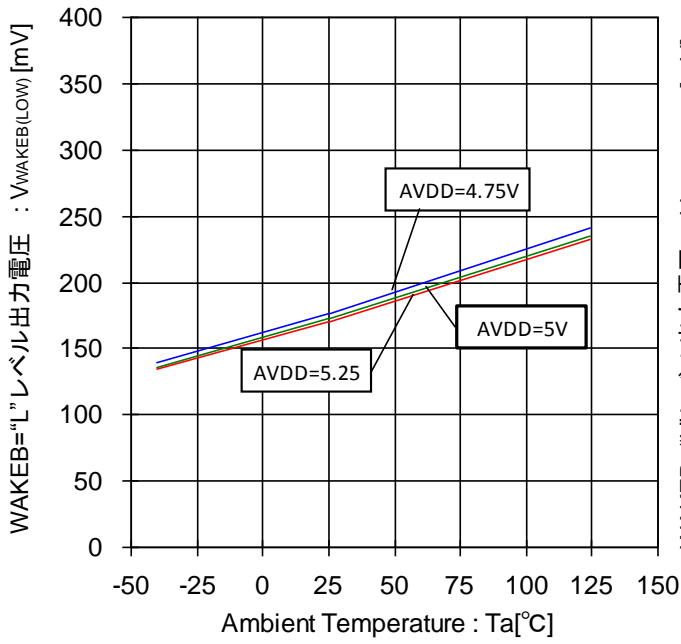
Figure 105. WAKEB="L"レベル出力電圧-温度特性 (WAKEB=1.0mA)
