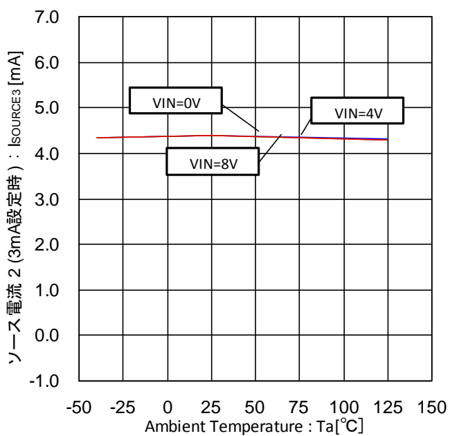
Figure 41. ソース電流 2-温度特性 (3mA 設定時)
