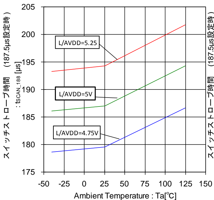
Figure 113. スイッチストロブ時間-温度特性 (187.5µs 設定時)
