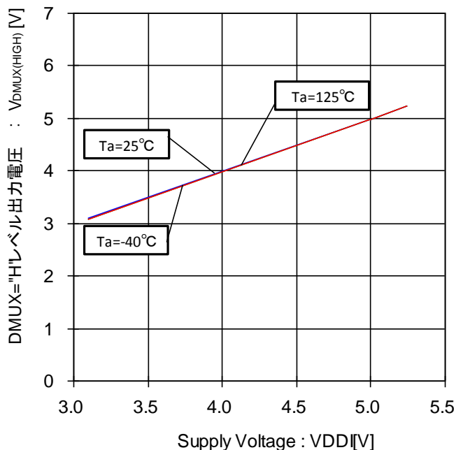
Figure 96. DMUX="H"レベル出力電圧-電圧特性 (Isource=200μA)
