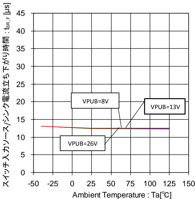
Figure 119. スイッチ入力ソース/シンク電流 立ち下がり時間-温度特性 (FSQ="0", FSQZ/A/B="0", 10mA 設定時 負荷抵抗 100Ω)
