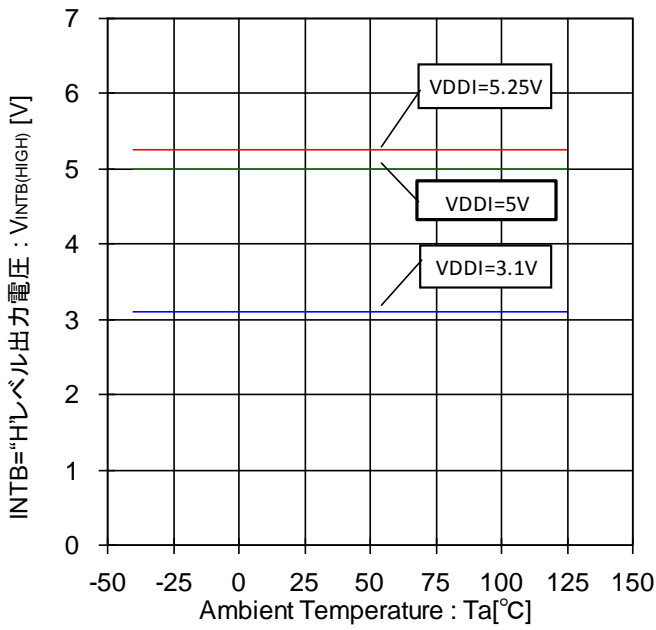
Figure 101. INTB="H"レベル出力電圧-温度特性 (INTB=OPEN 状態)
