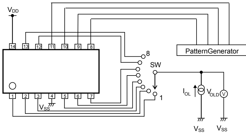
Figure 4. L 出力電圧測定回路
