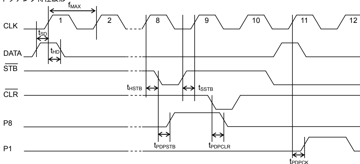
Figure 1. スイッチング特性波形
