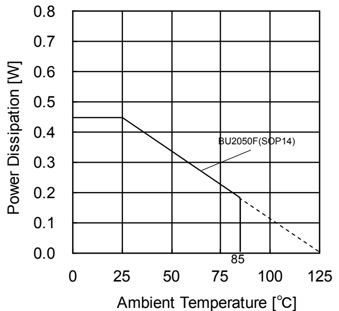
Figure 9. ディレーティングカーブ
