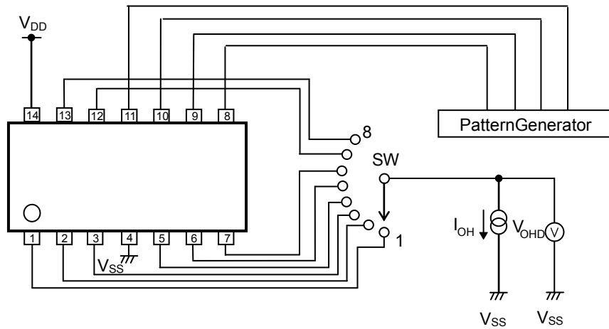
Figure 3. H 出力電圧測定回路
