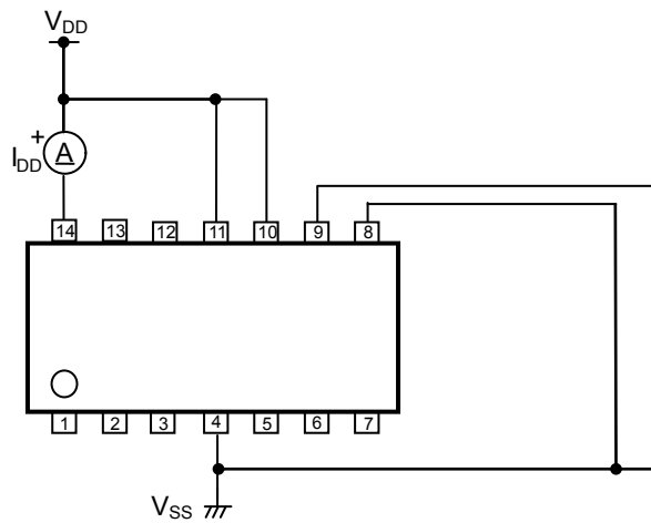
Figure 5. 静的消費電流 測定回路
