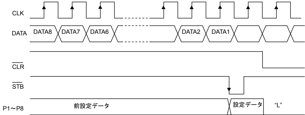
Figure 7. タイミングチャート
