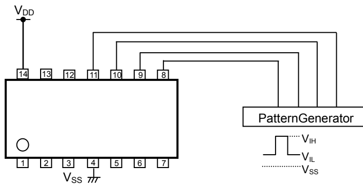
Figure 6. スイッチング特性 測定回路
