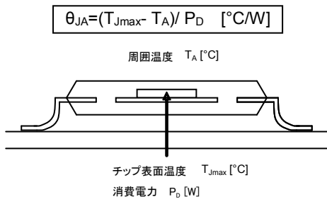
Figure 8. 熱抵抗
