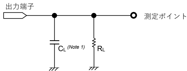
測定回路 ( t_{PLH} , t_{PHL} )
