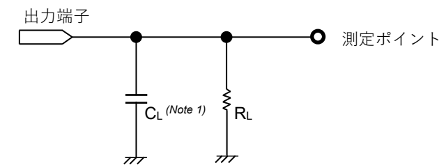
測定回路 ( t_{PLH} , t_{PHL} )
