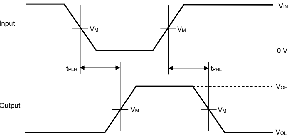
測定回路 / タイミングチャート
