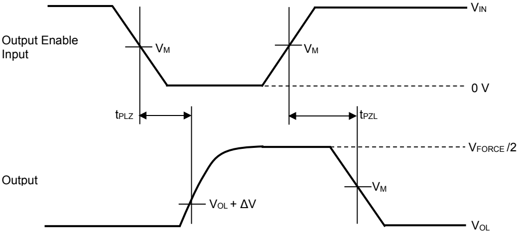
測定回路 / タイミングチャート( t_{PLZ} 、 t_{PZL} ), Input = L
