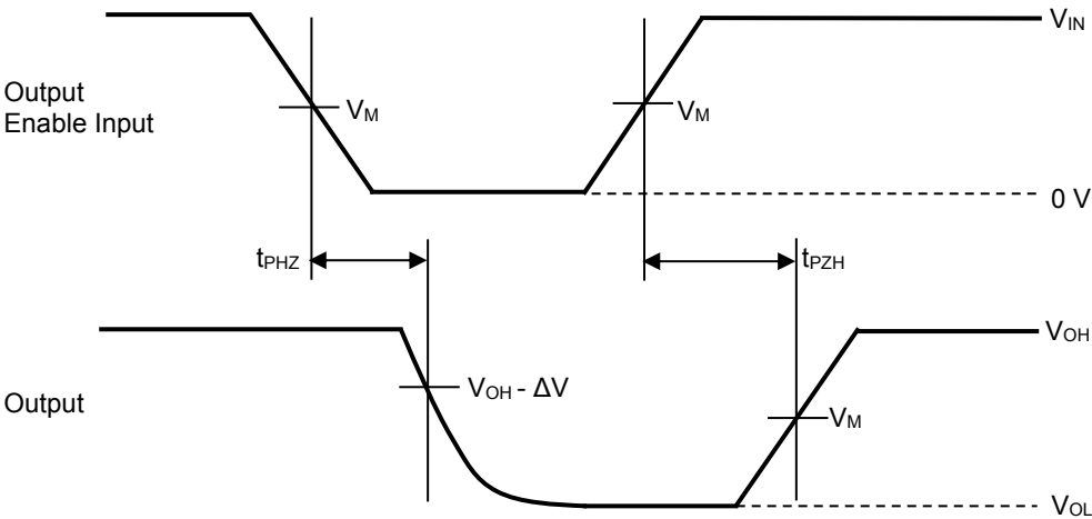
測定回路 / タイミングチャート( t_{PHZ} 、 t_{PZH} ), Input = H
