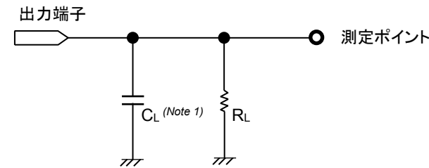
測定回路図 (t PLH 、t PHL )
