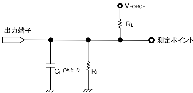
測定回路図 (t PLZ 、t PZL )
