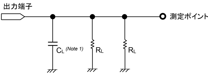
測定回路図 (t PHZ 、t PZH )
