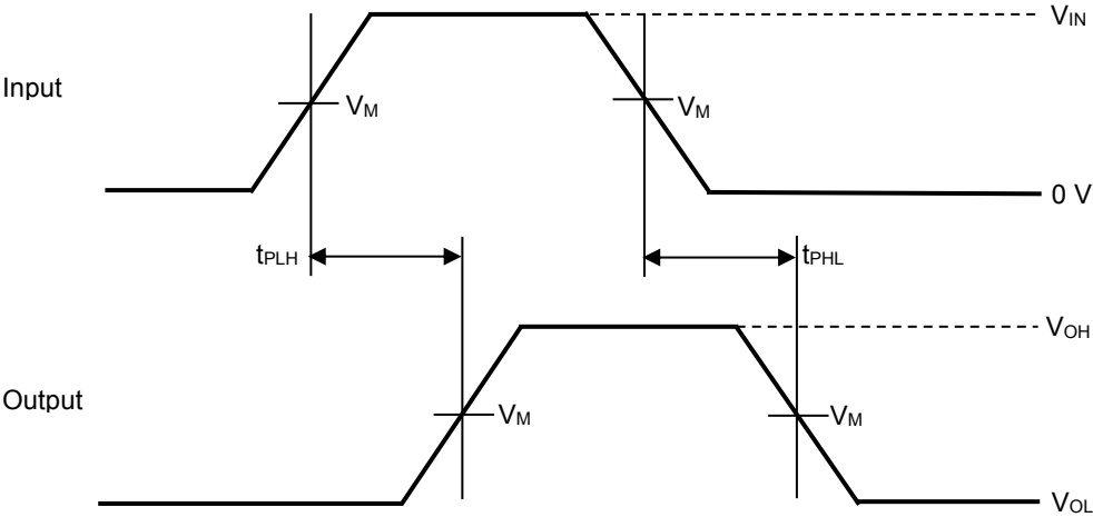
測定回路 / タイミングチャート( t_{PLH} 、 t_{PHL} )
