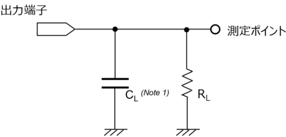
測定回路図 ( t_{PLH} , t_{PHL} )
