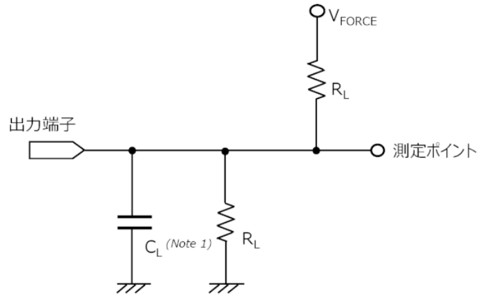
測定回路図 ( t_{PLZ} , t_{PZL} )
