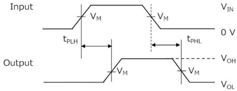
タイミングチャート ( t_{PLH} , t_{PHL} )
