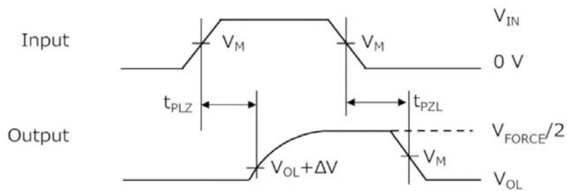
タイミングチャート ( t_{PLZ} , t_{PZL} )
