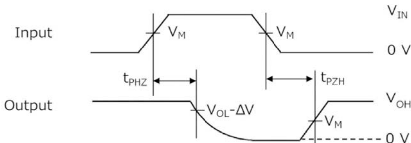
タイミングチャート ( t_{PHZ} , t_{PZH} )
