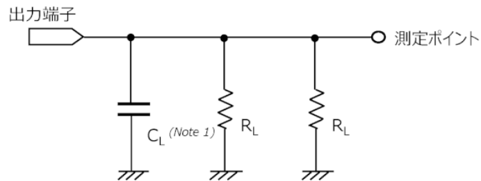
測定回路図 ( t_{PHZ} , t_{PZH} )
