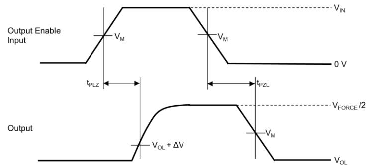
タイミングチャート( t_{PLZ} 、 t_{PZL} )
