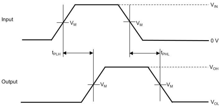
タイミングチャート( t_{PLH} 、 t_{PHL} )
