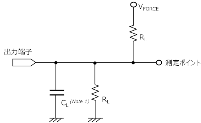
測定回路図 ( t_{PLZ} , t_{PZL} )
