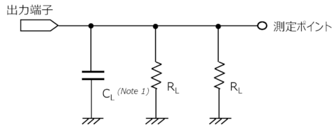
測定回路図 ( t_{PHZ} , t_{PZH} )
