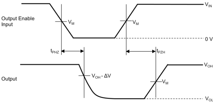
タイミングチャート( t_{PHZ} 、 t_{PZH} )
