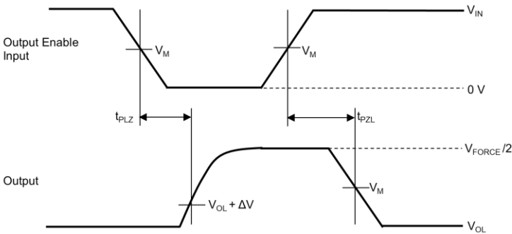
タイミングチャート( t_{PLZ} 、 t_{PZL} )
