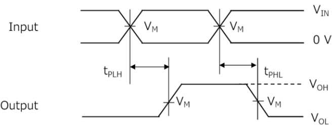
測定回路 / タイミングチャート
