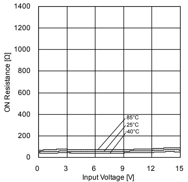
Figure 10. ON 抵抗 vs 入力電圧特性 V DD =15V
