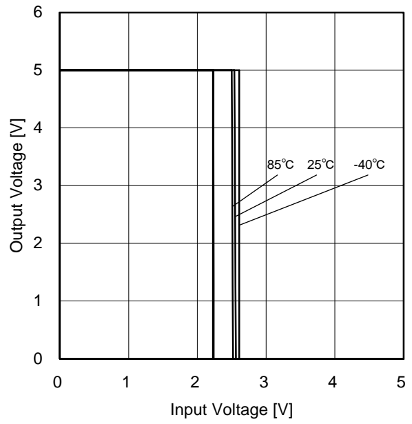
Figure 2. 出力電圧 vs 入力電圧特性 ( V_{DD}=5V / V_{SS}=0V )
