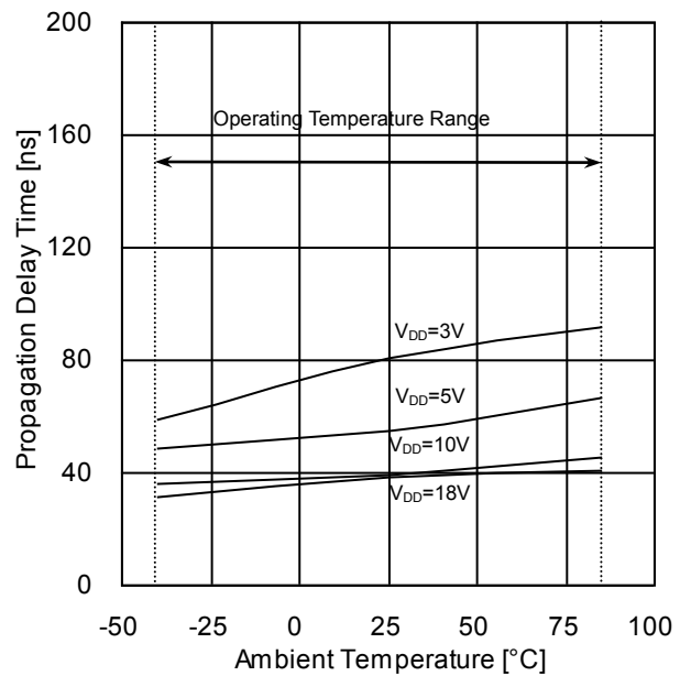
Figure 15. 伝達遅延時間 CONT→OUT(t PHZ )—温度特性
