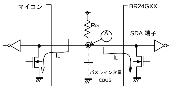
Figure 44. I/O 回路図
