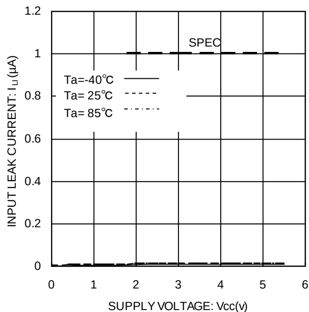
Figure 8. 入力リーク電流 ILI (A1,A2,SCL,WP)
