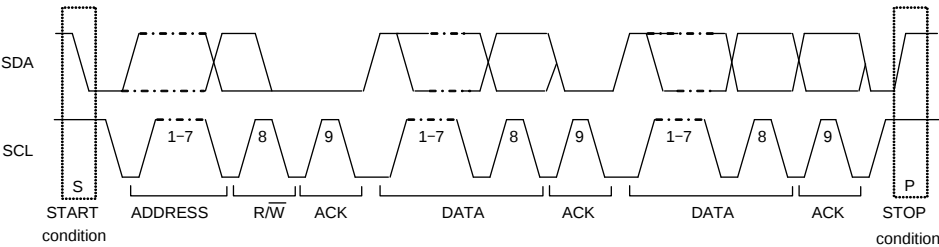
Figure 39. データ転送タイミング
