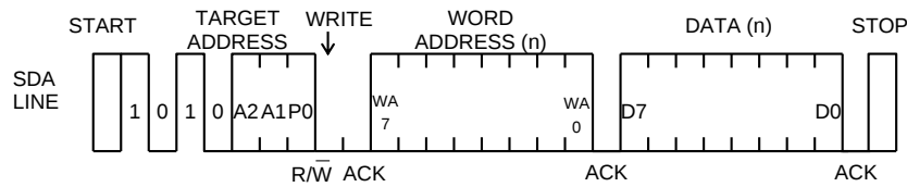
Figure 40. バイトライト
