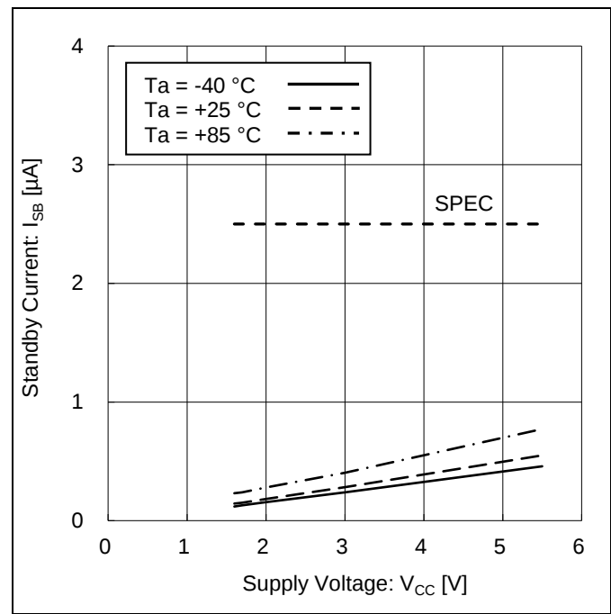
Figure 14. スタンバイ電流 vs 電源電圧
