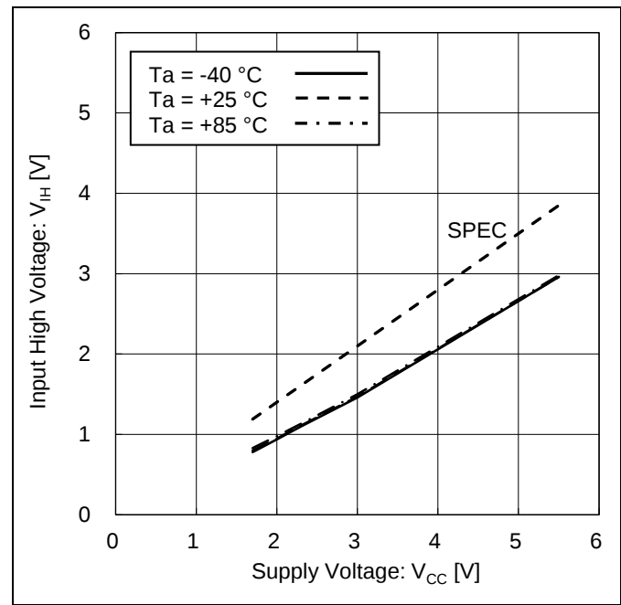
Figure 6. 'HIGH'入力電圧 1,2 vs 電源電圧
