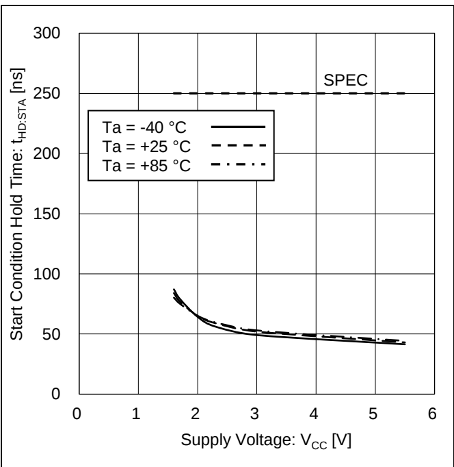
Figure 19. スタートコンディションホールド時間 vs 電源電圧
