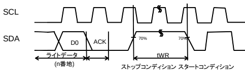
Figure 2(c). 書き込みサイクルタイミング
