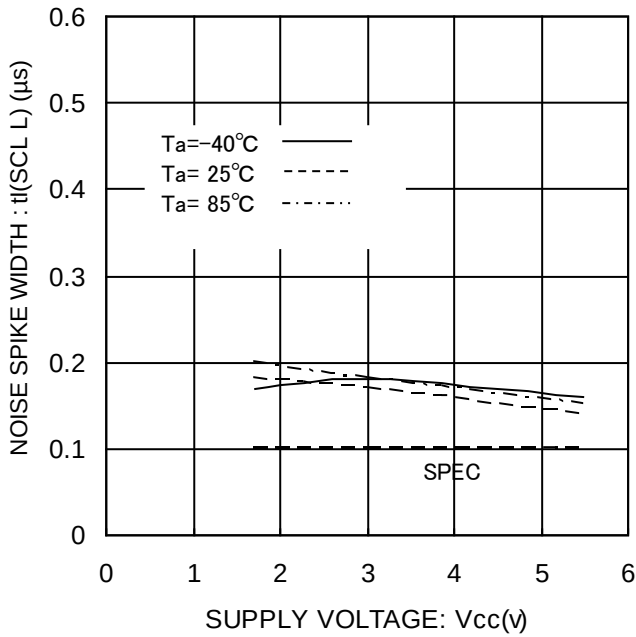
Figure 28. ノイズ除去有効時間 t_I (SCL L)
