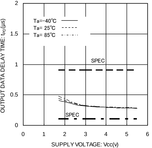
Figure 22. 出力データ遅延時間 t_{PD} (LOW)
