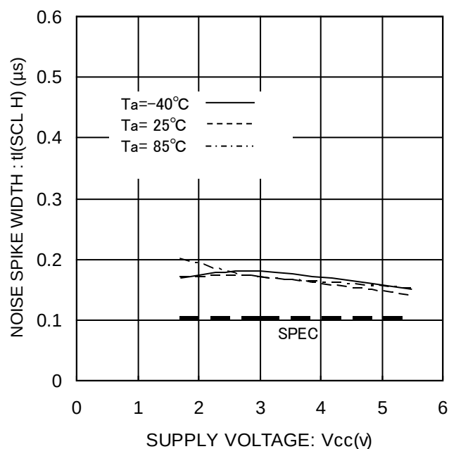
Figure 27. ノイズ除去有効時間 t_l (SCL H)
