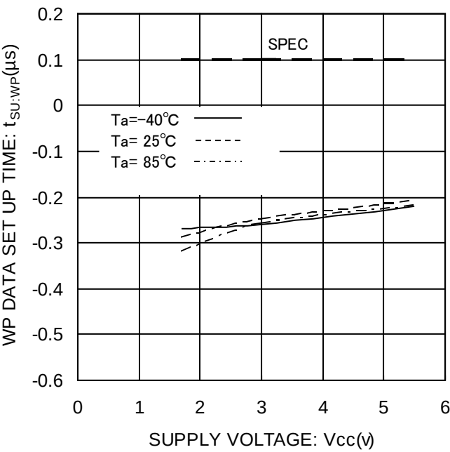
Figure 32. WP セットアップ時間 t_{SU:WP}
