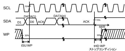
Figure 2(d). ライト実行時 WP タイミング
