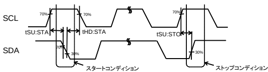
Figure 2(b). スタート・ストップタイミング
