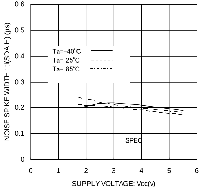
Figure 29. ノイズ除去有効時間 t_I (SDA H)
