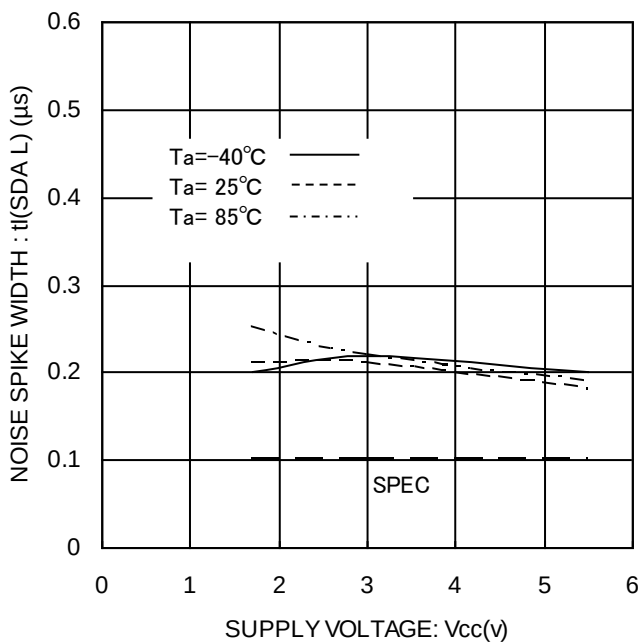
Figure 30. ノイズ除去有効時間 t_I (SDA L)
