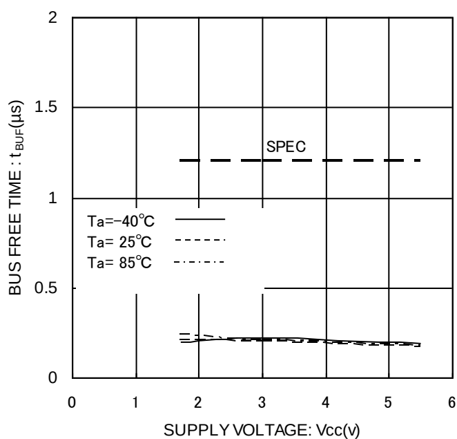
Figure 25. 転送開始前バス開放時間 t_{BUF}
