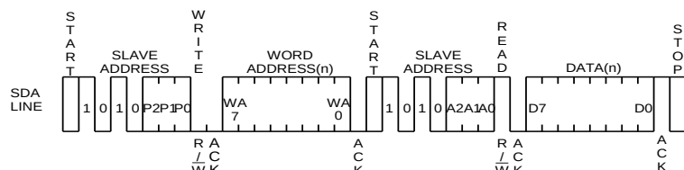
Figure 37. ランダムリードサイクル
