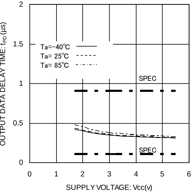
Figure 23. 出力データ遅延時間 t_{PD} (HIGH)
