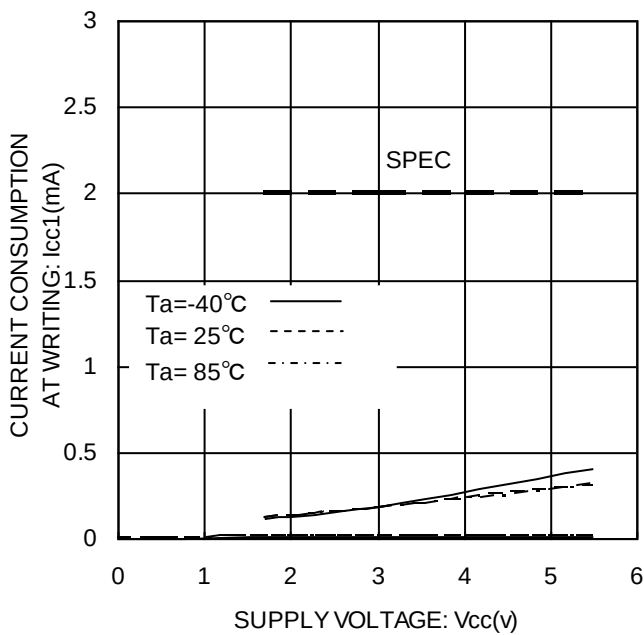
Figure 10. ライト動作時消費電流 ICC1 (fsc1=400kHz)
