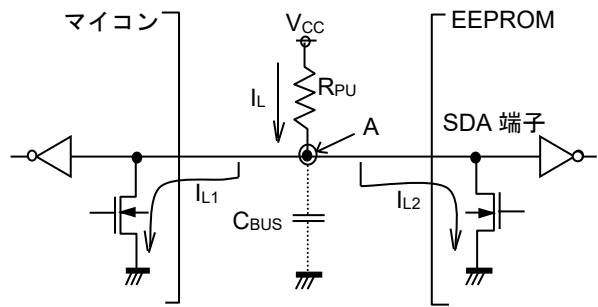
Figure 51. I/O 回路図
