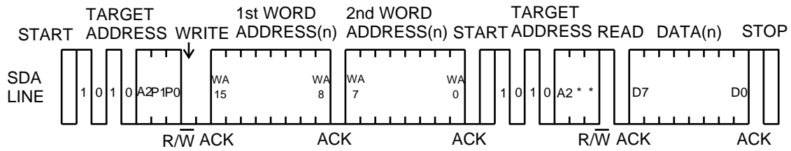
Figure 44. ランダムリード
