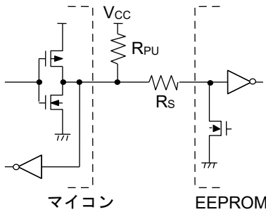
Figure 52. I/O 回路図
