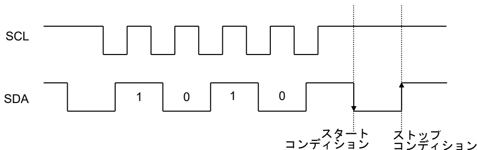
Figure 50. ターゲットアドレス入力中にスタート・ストップコンディションでキャンセルした場合
